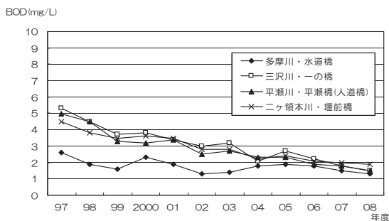
多摩川水系のBOD経年変化(年度平均値)
