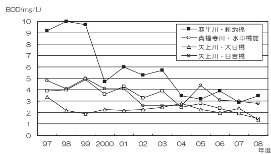
鶴見川水系のBOD経年変化(年度平均値)
