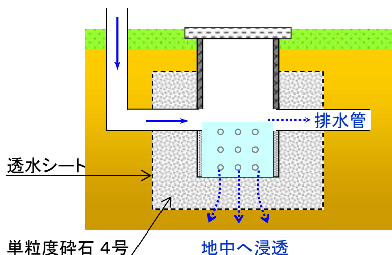
雨水浸透ますの構造
