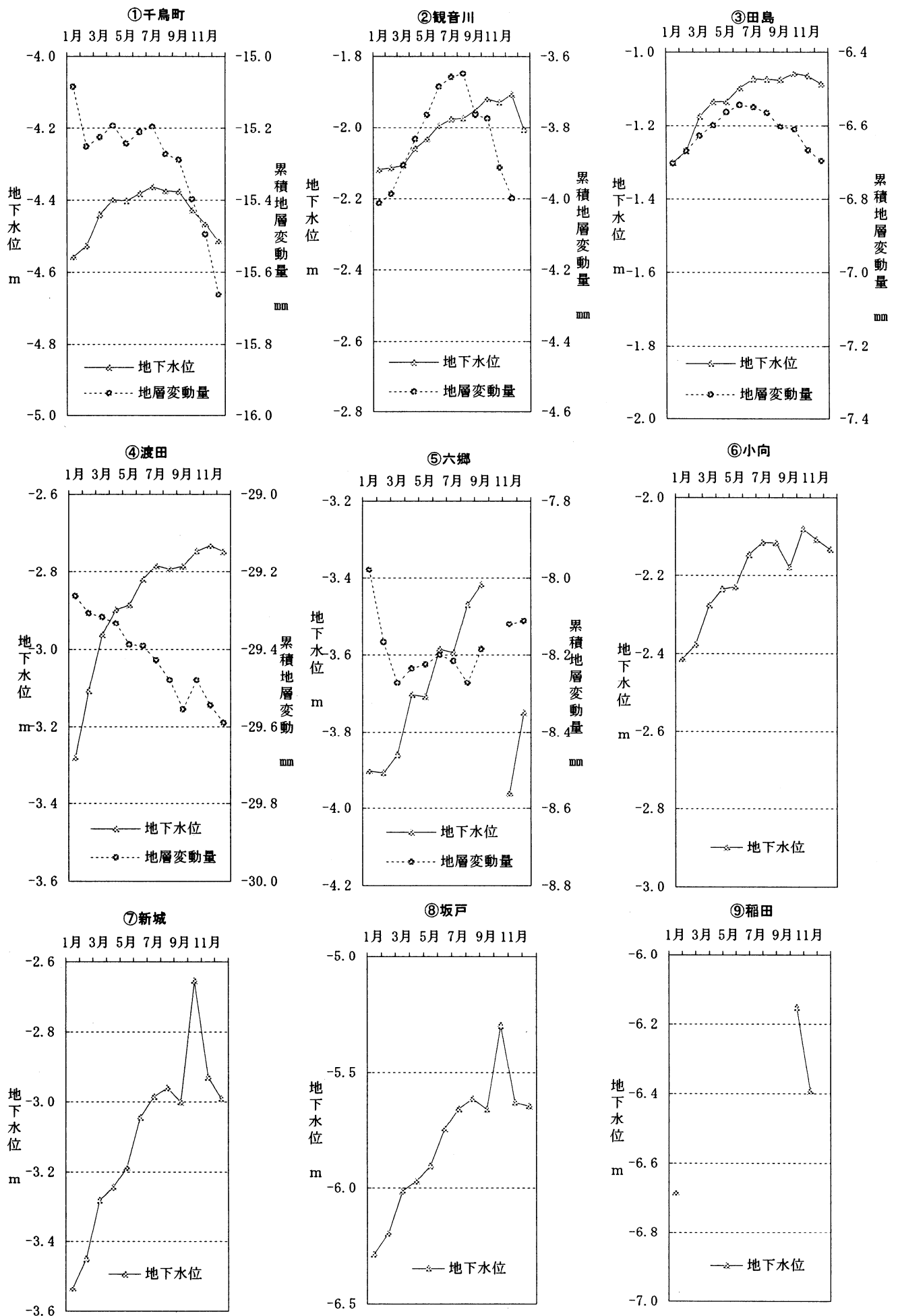
図15 地下水位-地層年間変動の年間推移 (月平均 H18.1~H18.12) (⑥~⑨は地下水位のみ)
