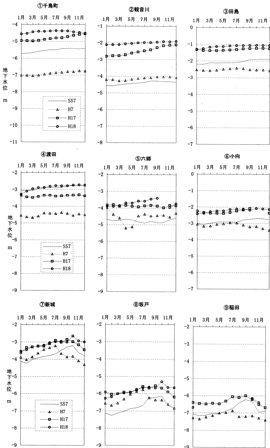
図13 地下水位の年間変動の経年推移
