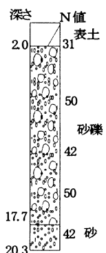
伏流水地域柱状図
