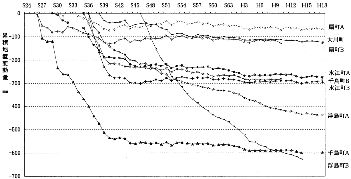
図9 主要水準点における累積地盤変動量の経年推移
