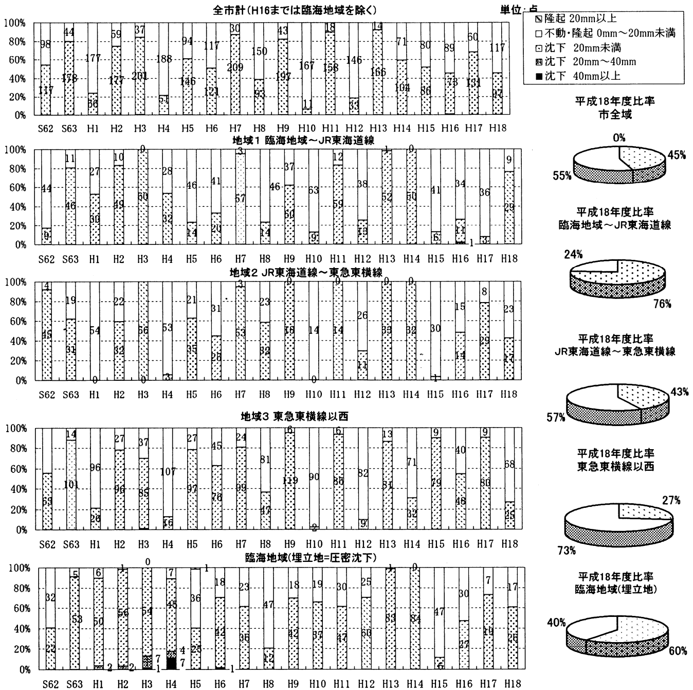
図7 精密水準測量結果の経年推移
