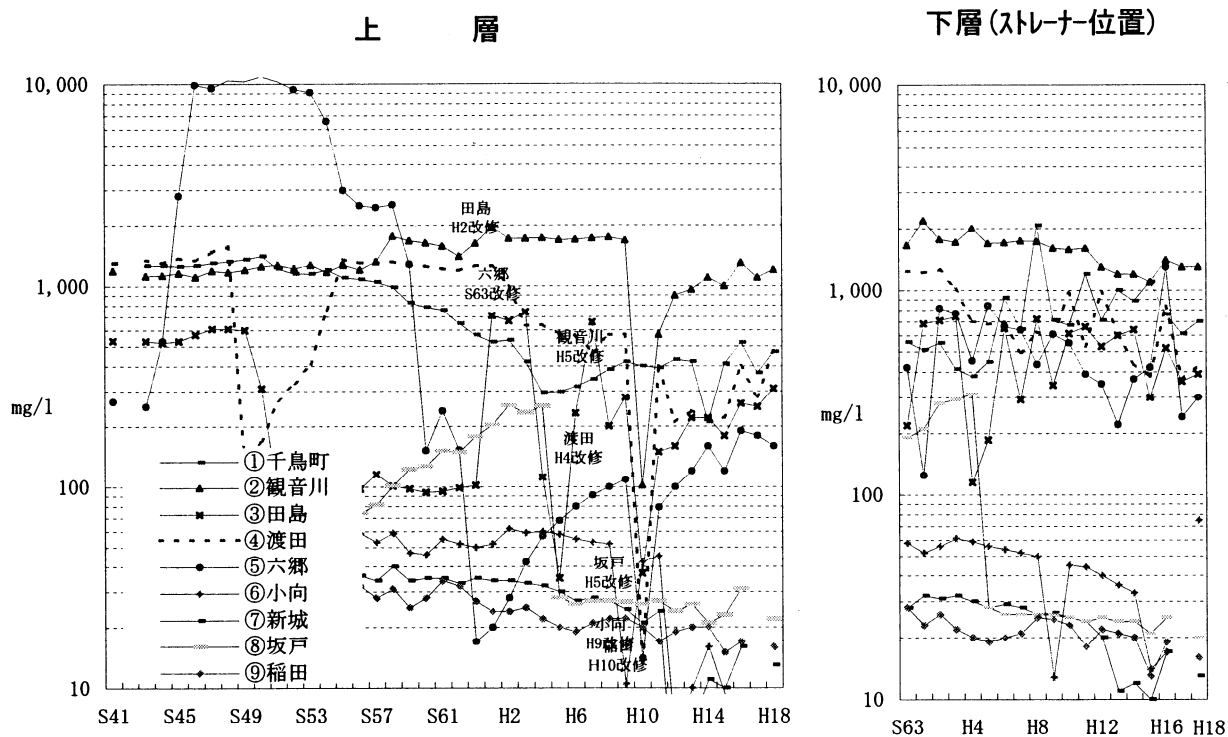
図17 地下水塩化物イオン濃度の経年推移
