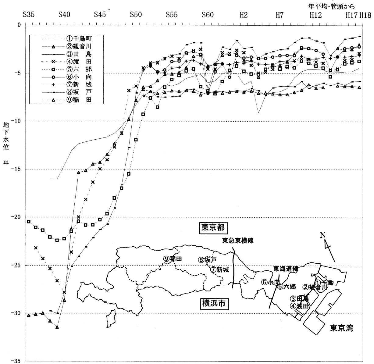
図14 地下水位の経年推移
