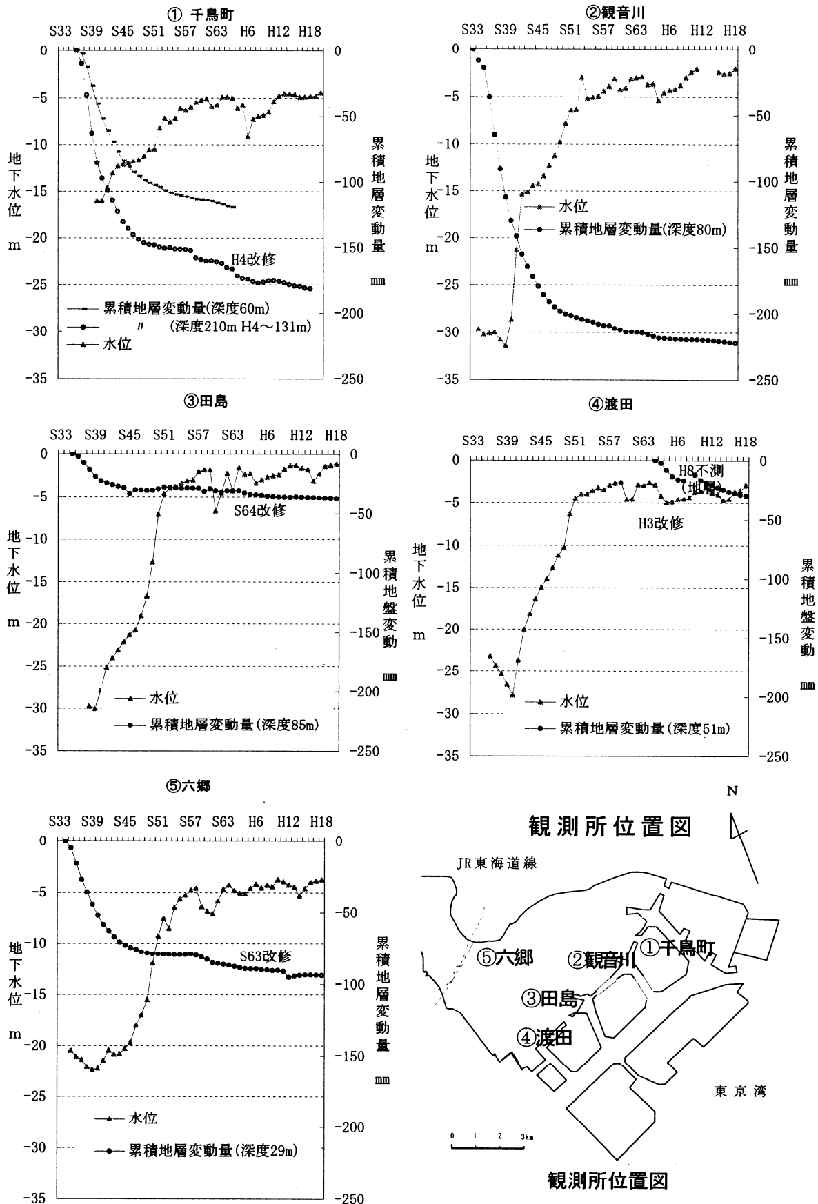
図16 地下水位-累積地層変動量の経年推移
