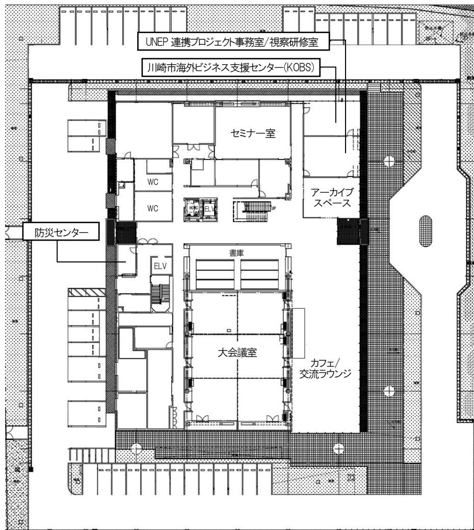
1階 平面図
