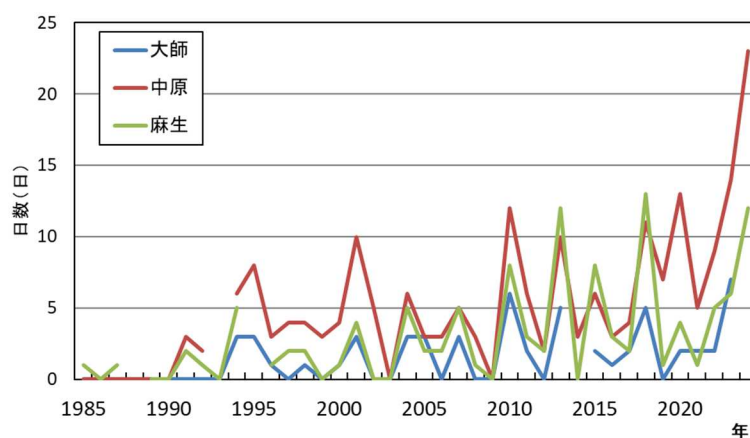
図 10 猛暑日の日数の経年変化
