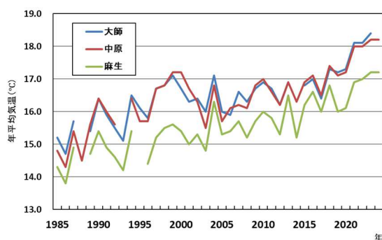
図2 年平均気温の経年変化
