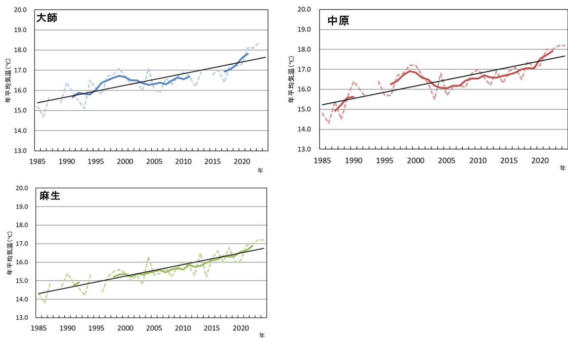
図3 年平均気温の5年移動平均と変化傾向
