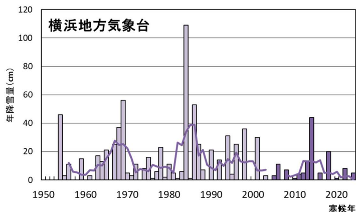
図 25 年降雪量の経年変化（横浜地方気象台、1954 年～2024 年） 9
