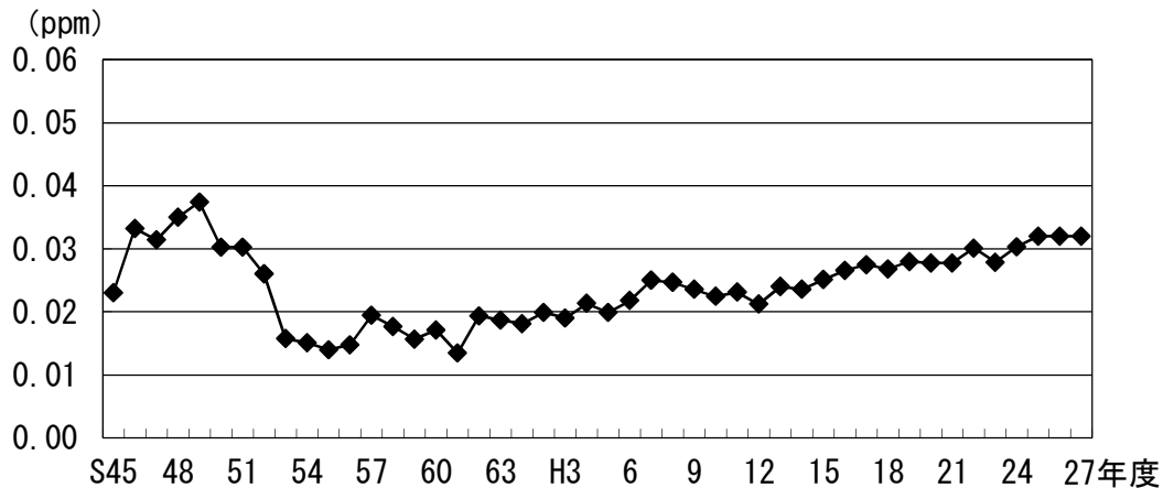
光化学オキシダント昼間年平均値の経年推移 (一般環境大気測定局平均)
