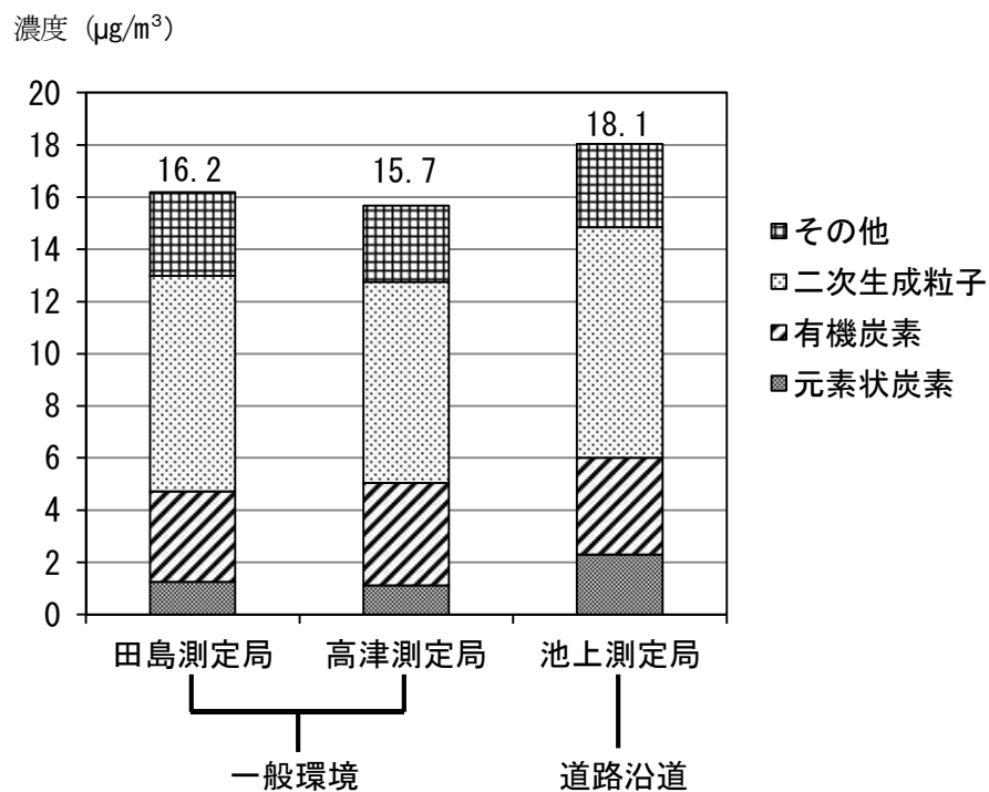
平成27年度微小粒子状物質濃度及びその成分濃度（年平均値）
