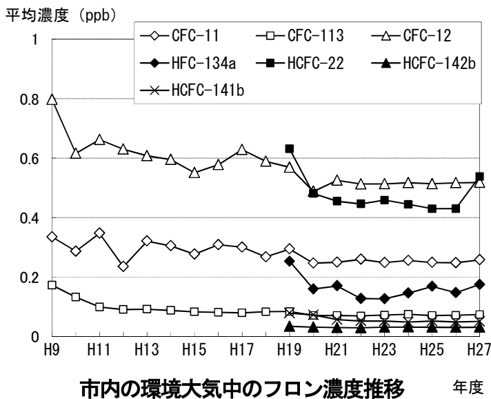
平成27年度フロン大気環境調査結果
