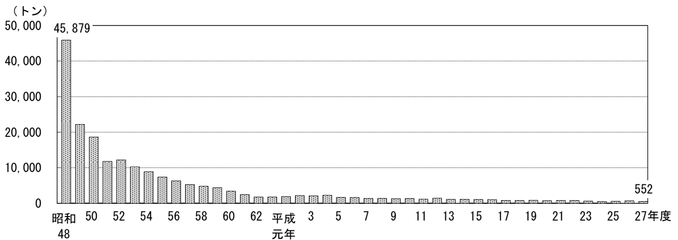
工場・事業場の硫黄酸化物排出量の経年推移
