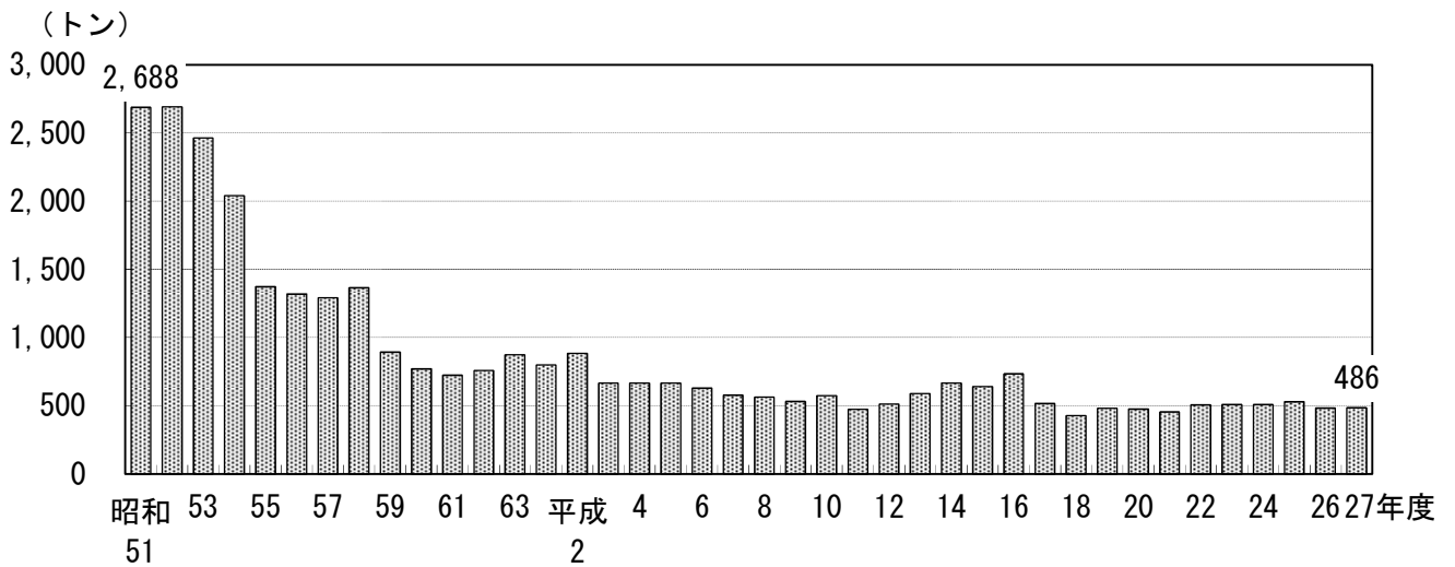
工場・事業場のばいじん排出量の経年推移
