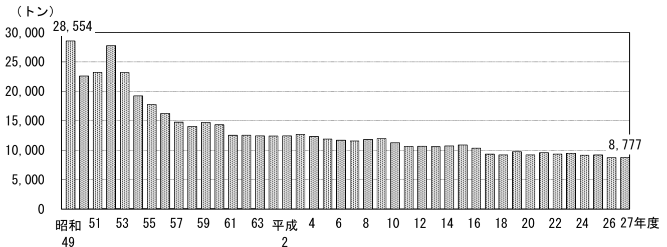
工場・事業場の窒素酸化物排出量の経年推移
