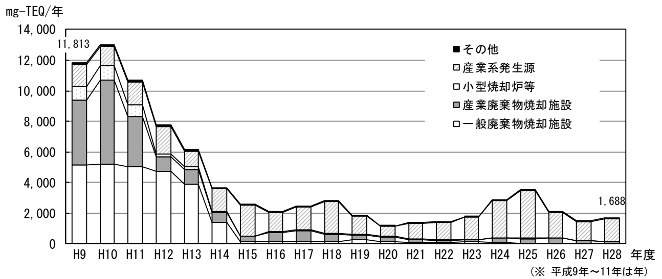
排出インベントリーの経年推移
