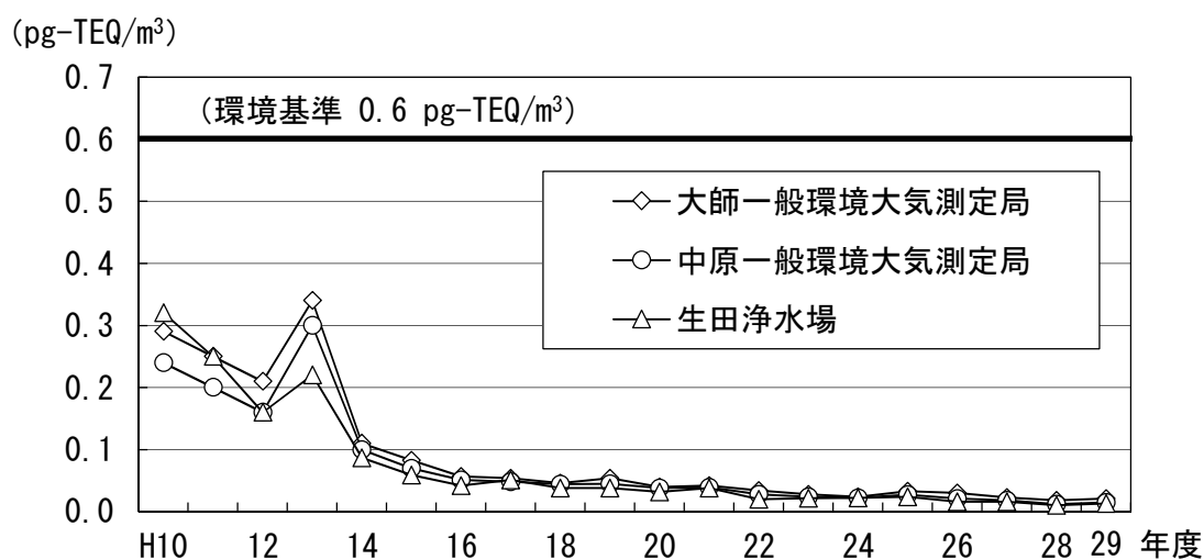
ダイオキシン類濃度の年平均値の推移（一般環境・大気）
