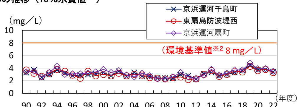
運河部のCODの推移（75%水質値※ 1 ）
