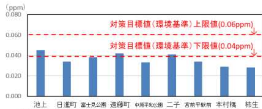
2022年度二酸化窒素濃度の対策目標値(環境基準)との比較 (自排局)
