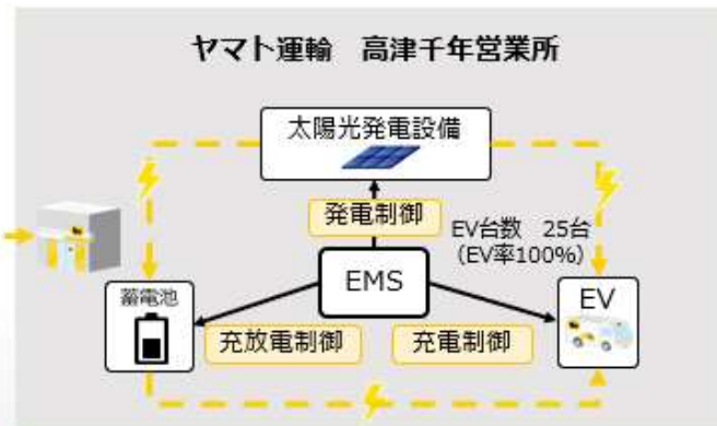
エネルギーマネジメントシステムの運用イメージ
