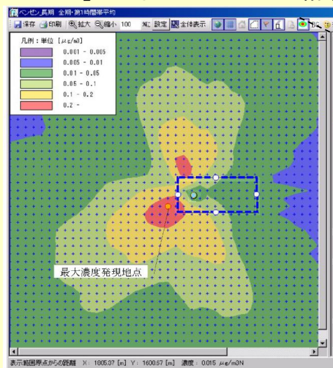
↓ 「METI-LIS *1 」によるシミュレーション結果のイメージ
