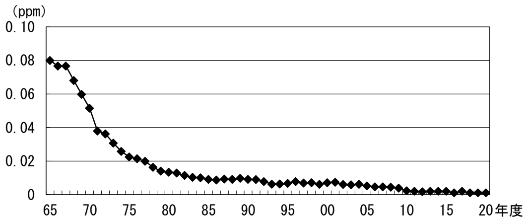
図9 二酸化硫黄濃度の年平均値の経年推移（一般環境大気測定局平均）
