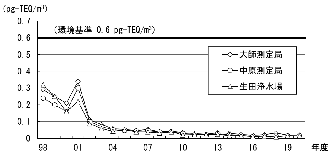
図12 大気中のダイオキシン類の年平均値の推移
