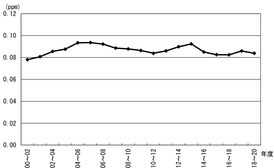
図8 日最高8時間値の年間99パーセンタイル値3年移動平均値の経年推移
