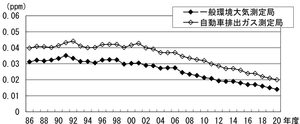
図2 二酸化窒素濃度の年平均値の経年推移
