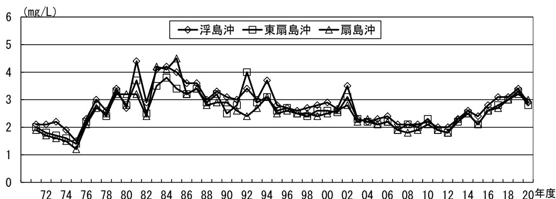
図19 海域・B類型のCODの年間平均値の経年推移
