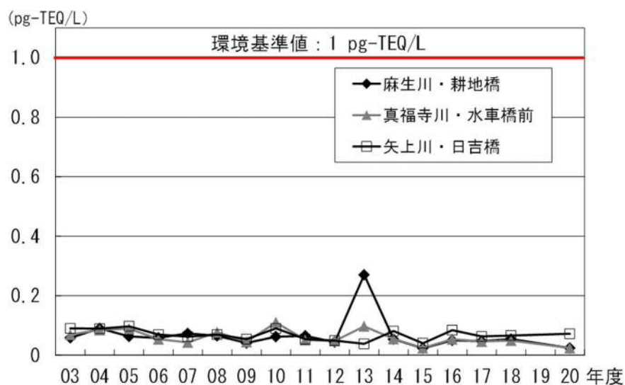
図 17 ダイオキシン類濃度の経年推移 (3 地点) (河川・水質)
