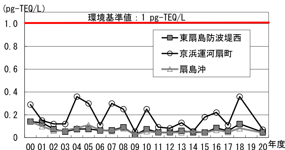
図 23 ダイオキシン類濃度の経年推移(3 地点)(海域・水質)
