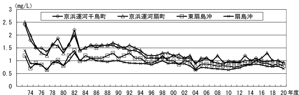
図21 海域の全窒素の年間平均値（全層）の経年推移
