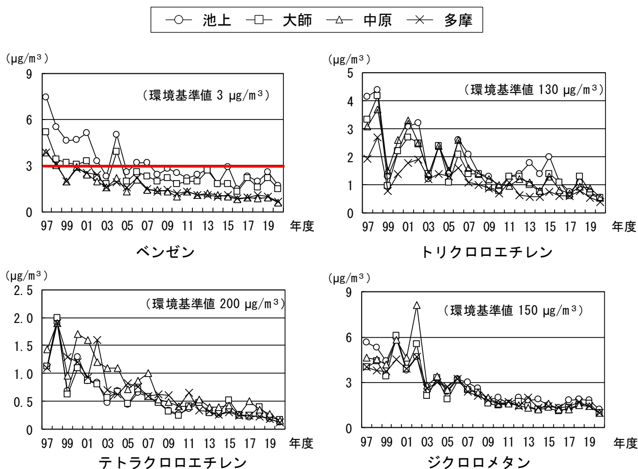
図11 有害大気汚染物質の年平均値の推移（環境基準が設定されている物質）
