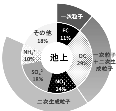
図 4 微小粒子状物質の成分分析結果 (年平均値)
