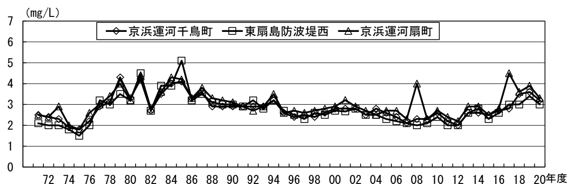
図20 海域・C類型のCODの年間平均値の経年推移
