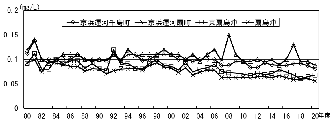
図 22 海域の全磷の年間平均値（全層）の経年推移
