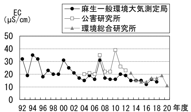
降水中の導電率(EC)の経年推移
