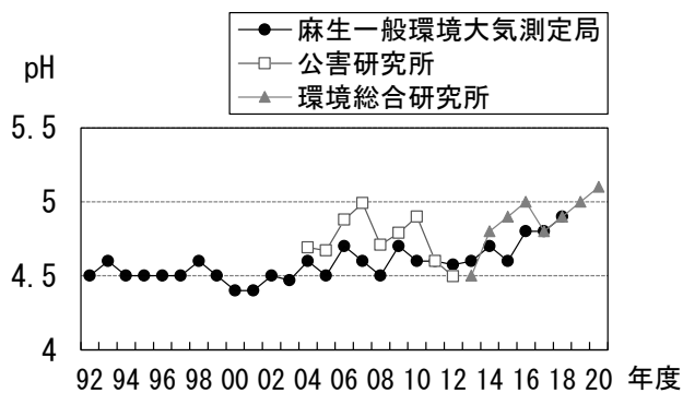
降水中のpHの経年推移
