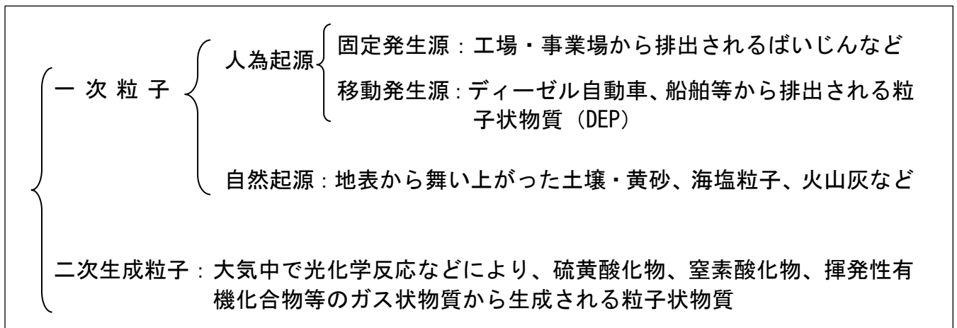
浮遊粒子状物質及び微小粒子状物質の発生源
