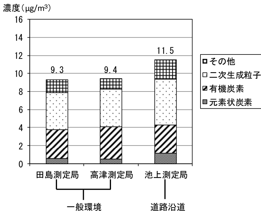
令和2(2020)年度微小粒子状物質濃度及びその成分濃度（年平均値）
