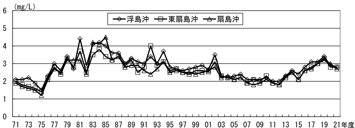
図21 海域・B類型のCODの年間平均値の経年推移
