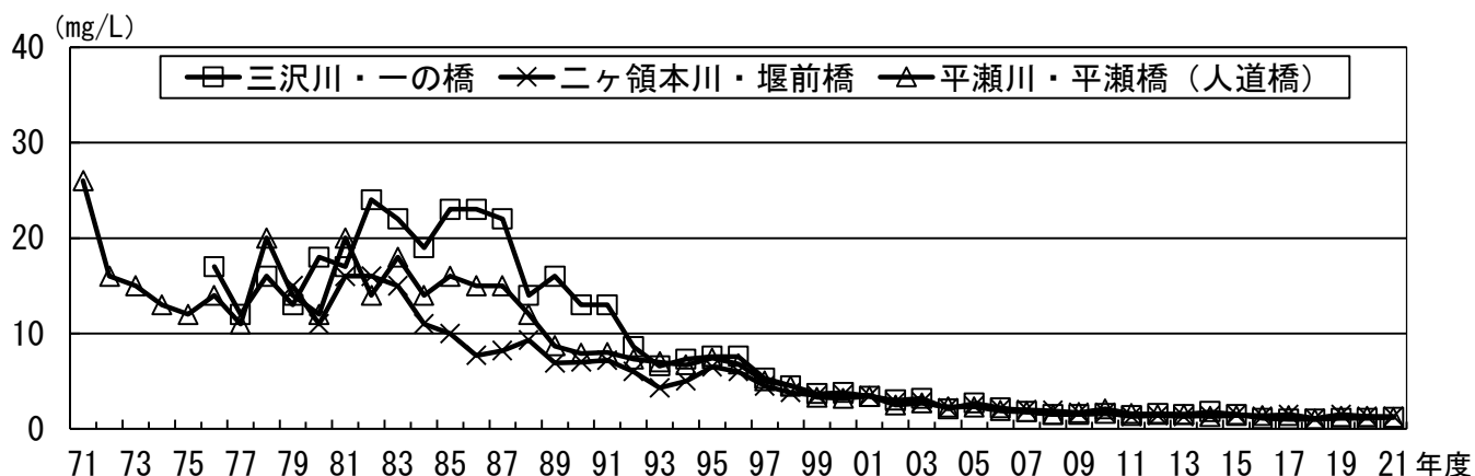
図 17 多摩川水系の BOD の年間平均値の経年推移
