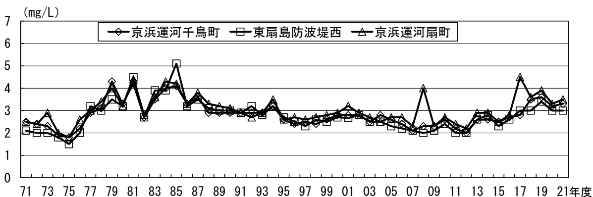
図22 海域・C類型のCODの年間平均値の経年推移
