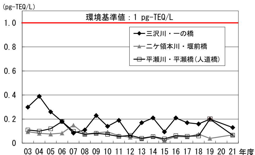
図 19 ダイオキシン類濃度の経年推移(3 地点) (河川・水質)
