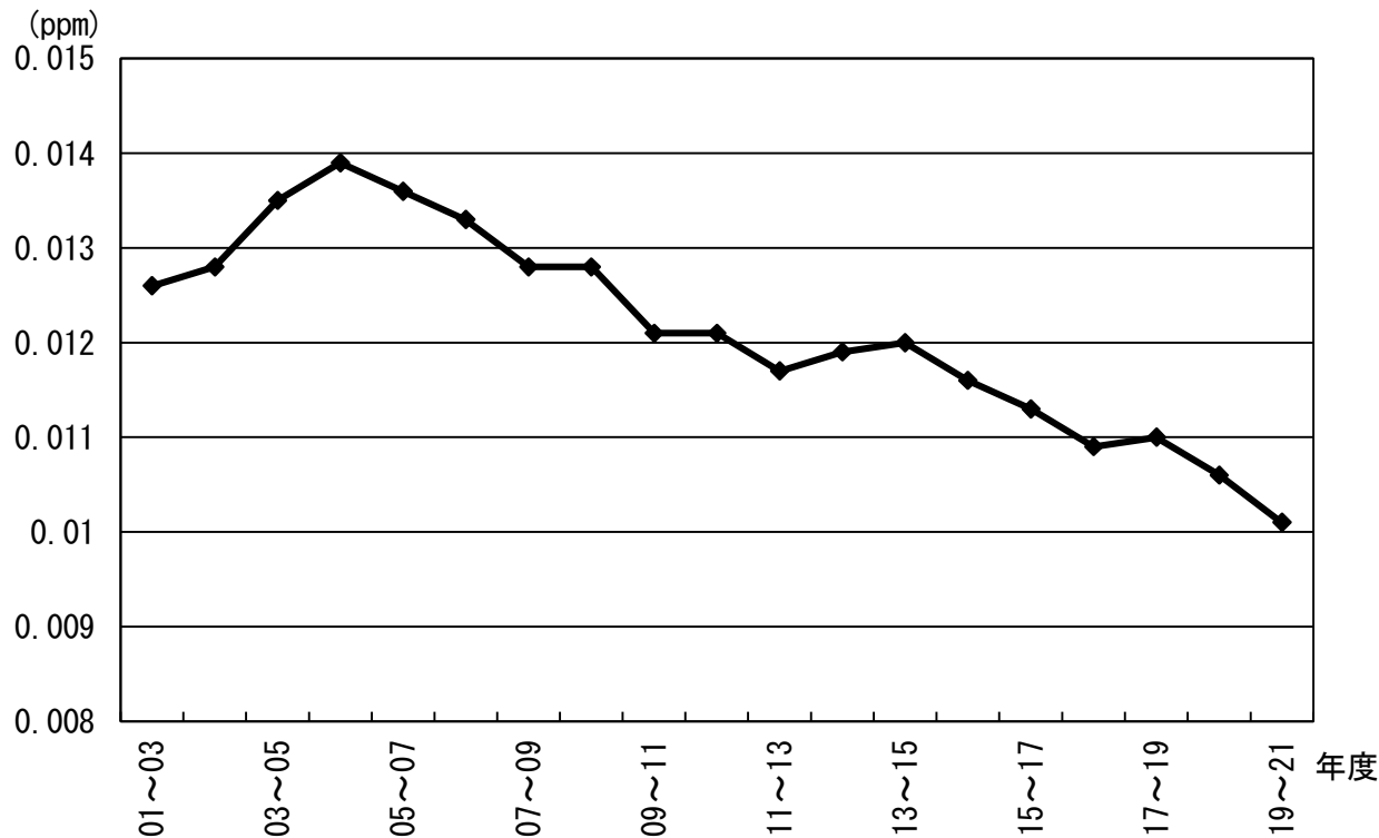
図10 光化学オキシダント環境改善評価指標値の経年推移
