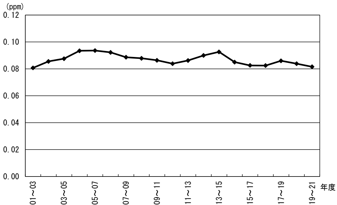
図8 光化学オキシダント濃度8時間値の日最高値の年間99パーセンタイル値の3年平均値の経年推移
