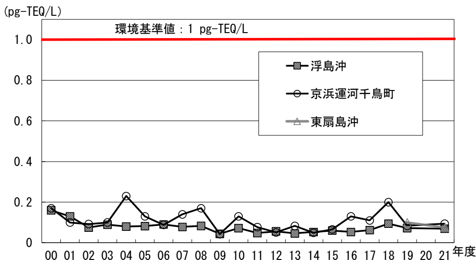
図 25 ダイオキシン類濃度の経年推移(3 地点) (海域・水質)
