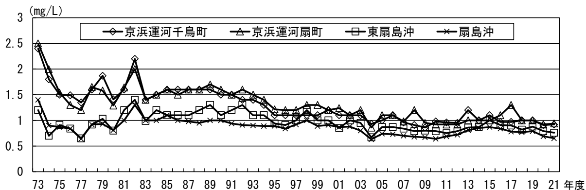
図23 海域の全窒素の年間平均値（全層）の経年推移
