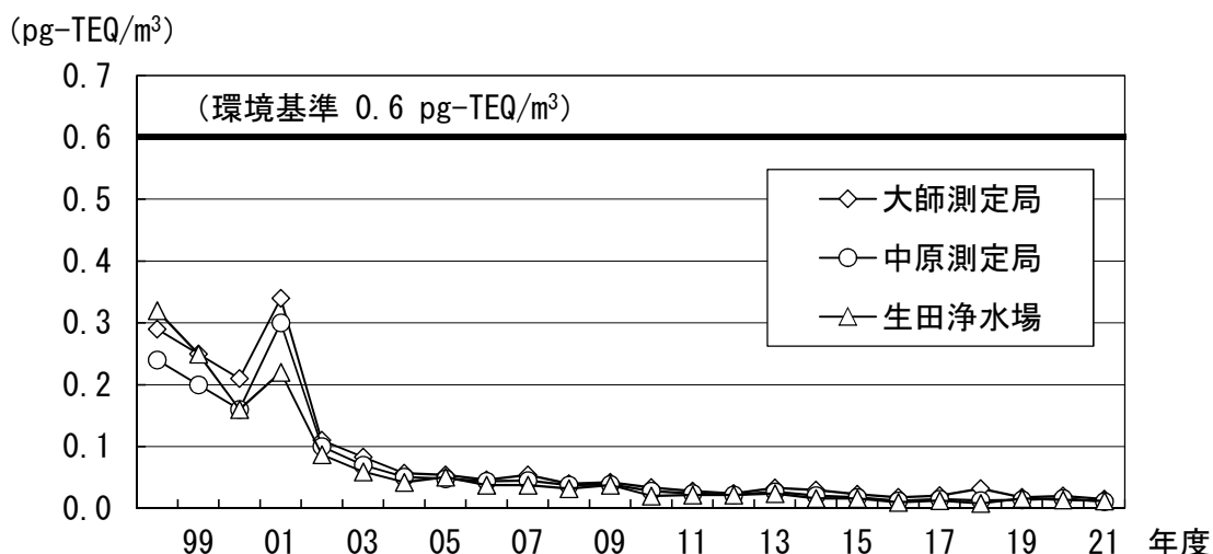
図14 大気中のダイオキシン類の年平均値の推移
