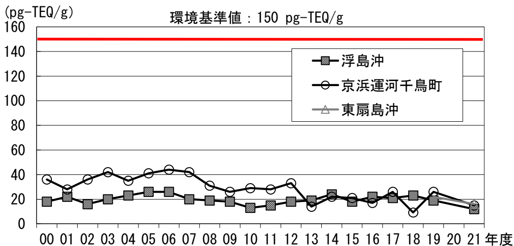
図26 ダイオキシン類濃度の経年推移(3地点) (海域・底質)
