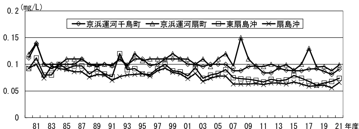
図 24 海域の全燐の年間平均値（全層）の経年推移
