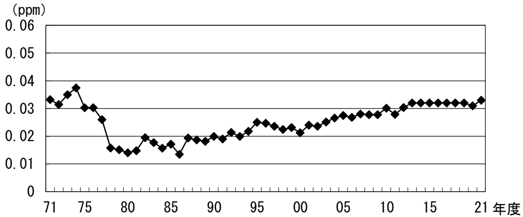
図7 光化学オキシダント濃度の昼間の年平均値の経年推移（一般環境大気測定局平均）
