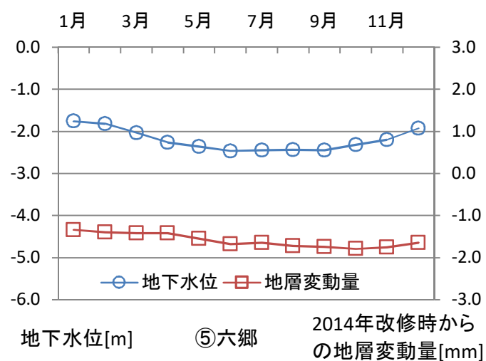
図V-15 地下水位[管頭から]-地層年間変動の年間推移(月平均 2021.1~2021.12)
