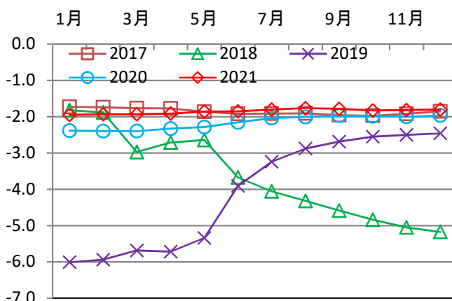
地下水位[m] ②観音川
