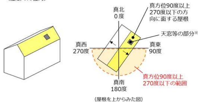
(屋根を上からみた図)
