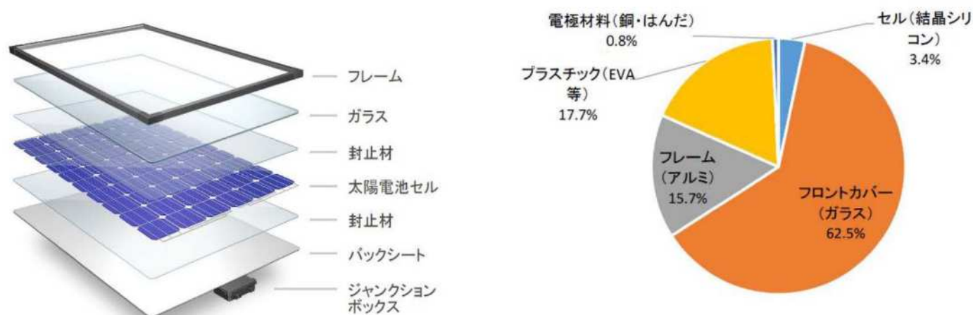
結晶シリコン系太陽電池モジュール(パネル)の構造と重量比
