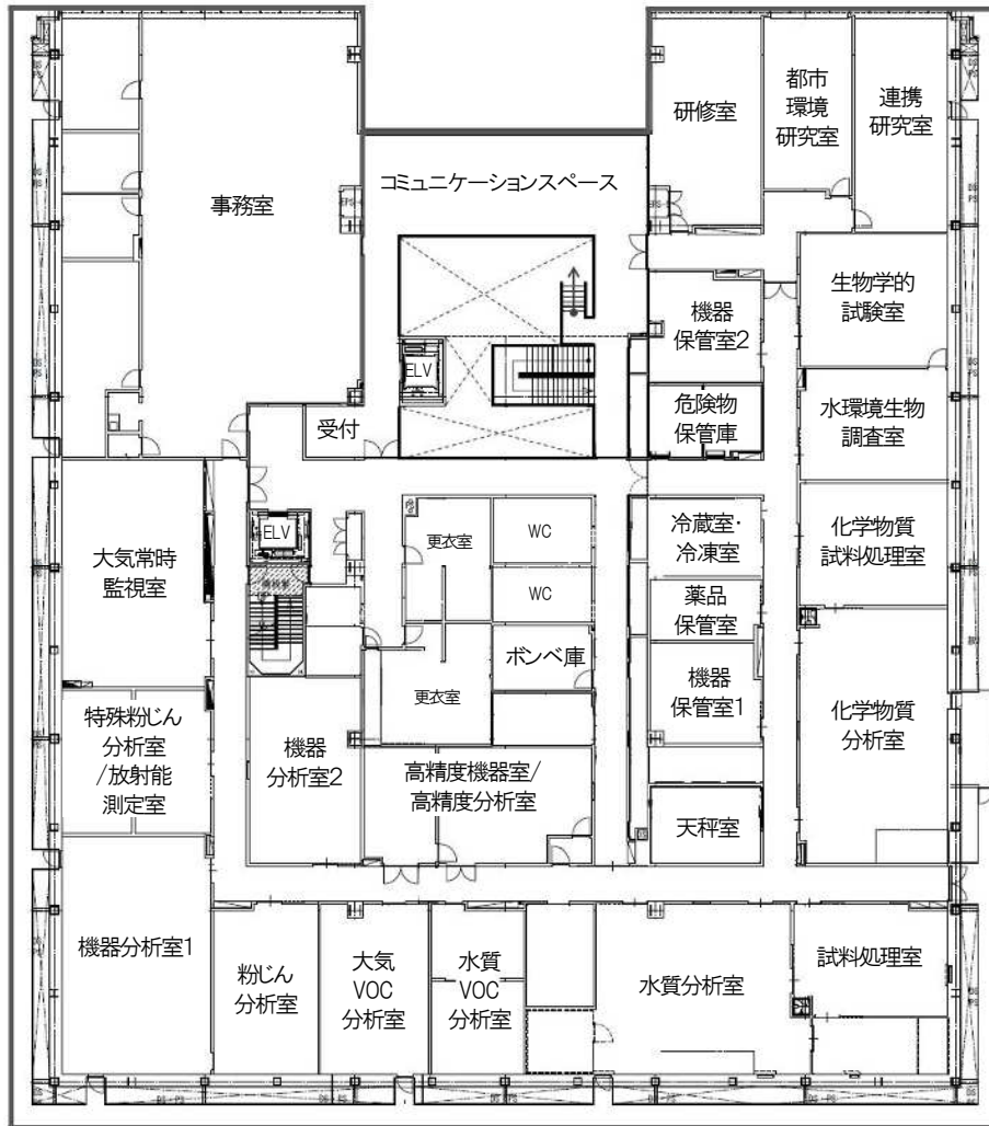
3階 平面図
