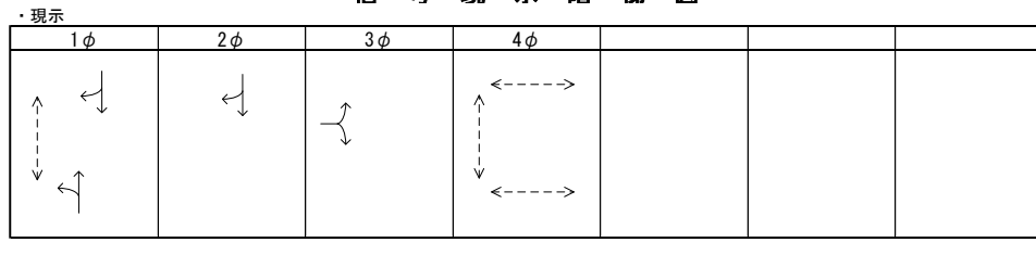
信号現示階梯図
