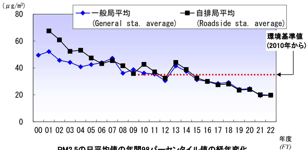
PM2.5の日平均値の年間98パーセンタイル値の経年変化 (A Long-Term Trend of 98th Percentile Value of Daily Average PM2.5 Concentration)
