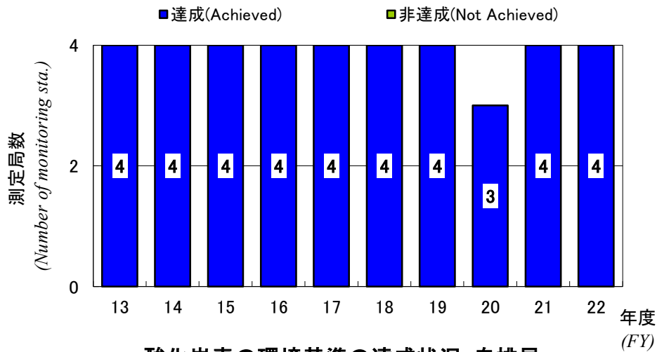
一酸化炭素の環境基準の達成状況：自排局 (Situation of Achievement for CO EQS: Roadside sta.)
