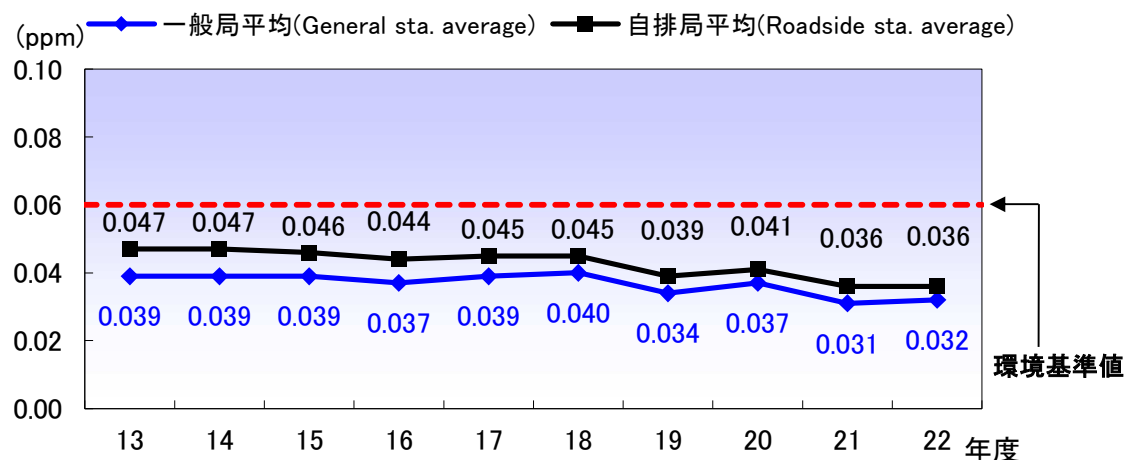
二酸化窒素の日平均値の年間98%値の推移(過去10年間) (FY) (Trend of 98 % Value of Daily Average NO 2 Concentration (The Last Ten Years))
