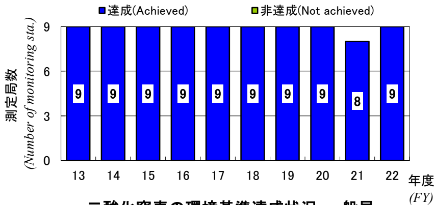
二酸化窒素の環境基準達成状況：一般局 (Situation of Achievement for NO_2 EQS:General sta.)
