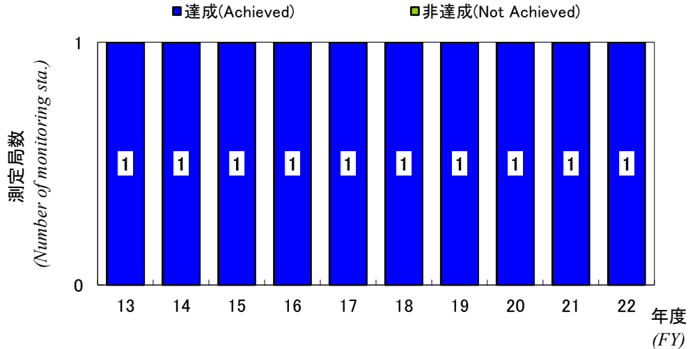
一酸化炭素の環境基準の達成状況：一般局 (Situation of Achievement for CO EQS: General sta.)
