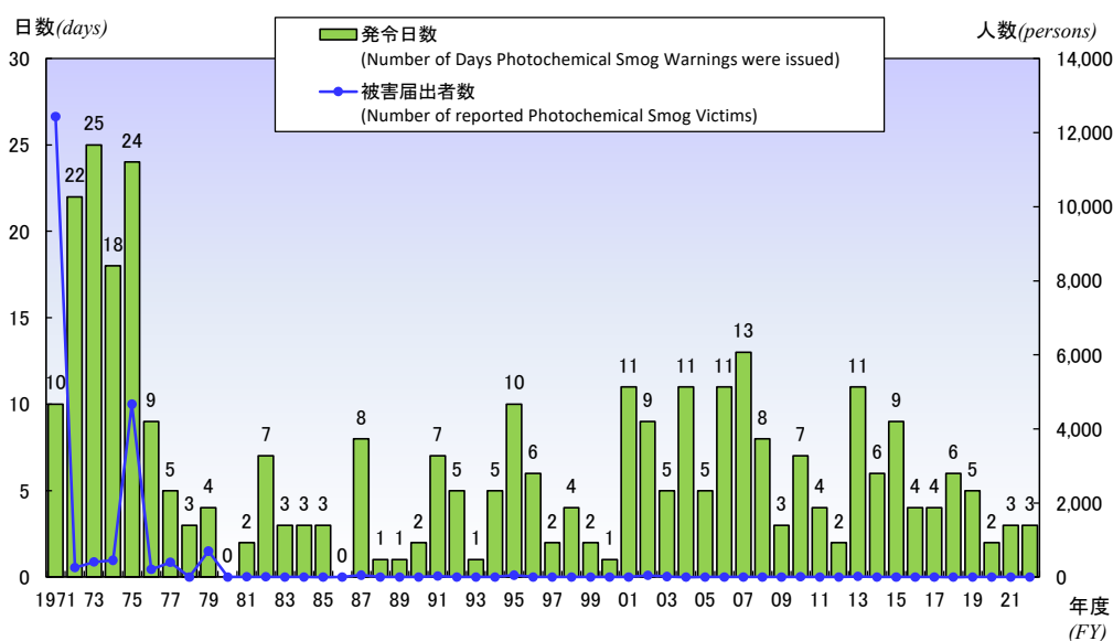
光化学スモッグ注意報の発令日数と被害届出者数の経年変化
