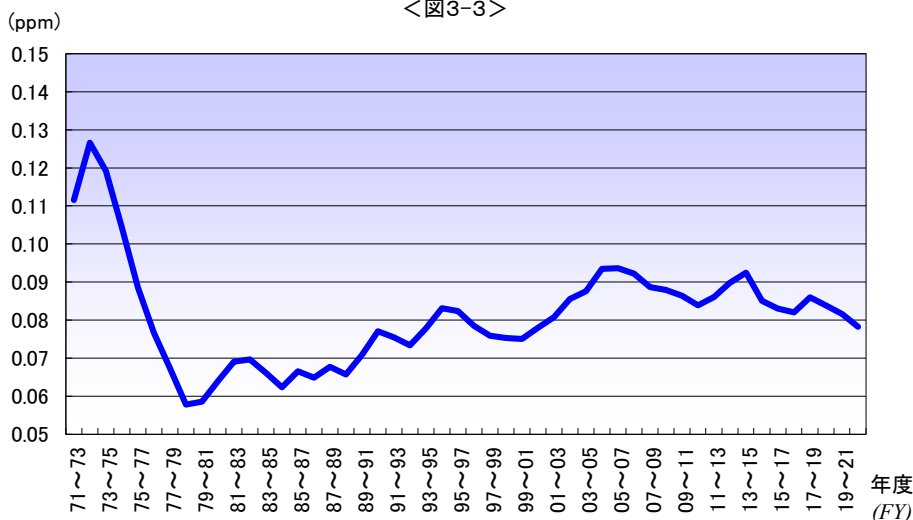
光化学オキシダント濃度8時間値の日最高値の年間99パーセンタイル値の3年平均値の経年変化
