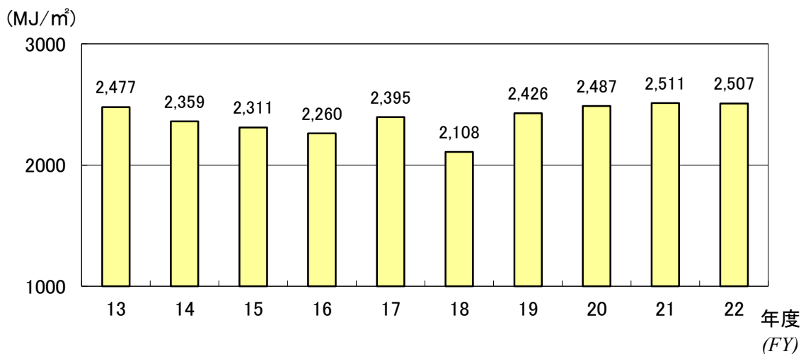
放射収支量の年合計値の推移(過去10年間) (Trend of Total Yearly Amount of Radiation Balance(The Last Ten Years)) <図9-8>
