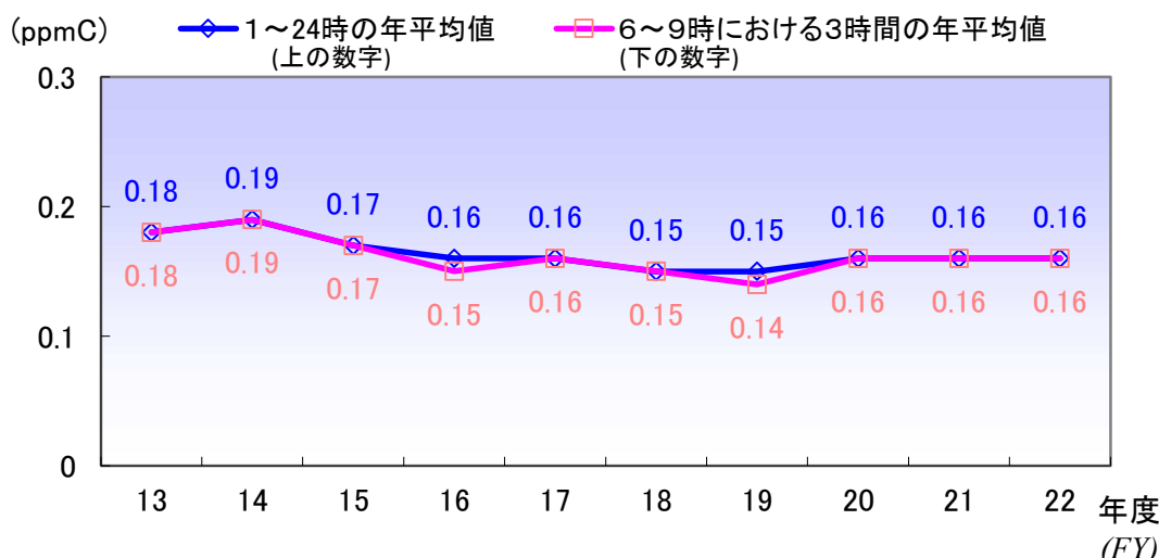
非メタン炭化水素の年平均値及び3時間平均値の推移(過去10年間) (Trend of Annual Average and 3-hour Average of NMHC Concentration(The Last Ten Years))
