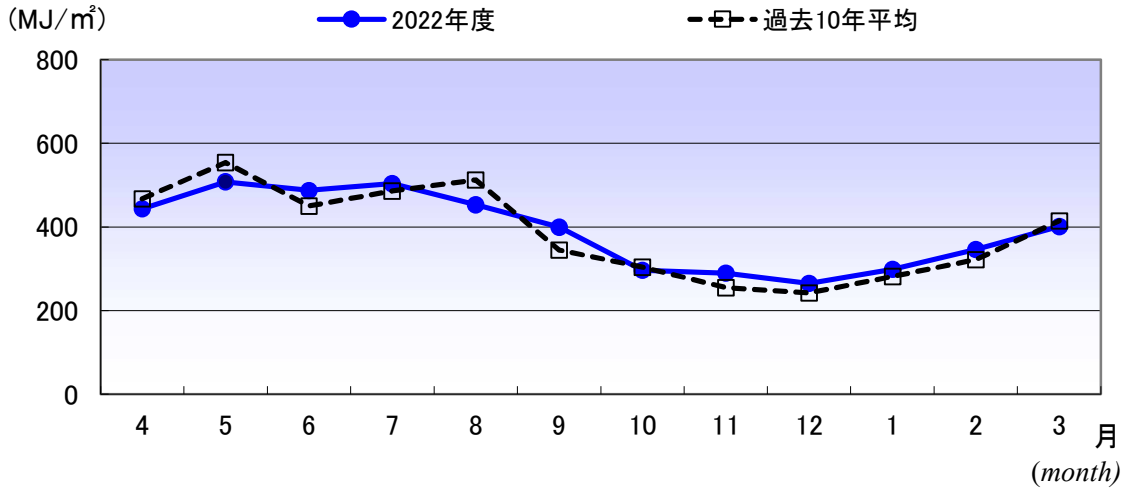
日射量の月合計値の平均の推移 注) (Trend of Total Monthly Amount of Solar Radiation) <図9-5>
