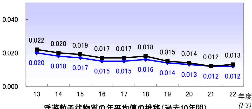
浮遊粒子状物質の年平均値の推移(過去10年間) (Trend of Annual Average SPM Concentration (The Last Ten Years))
