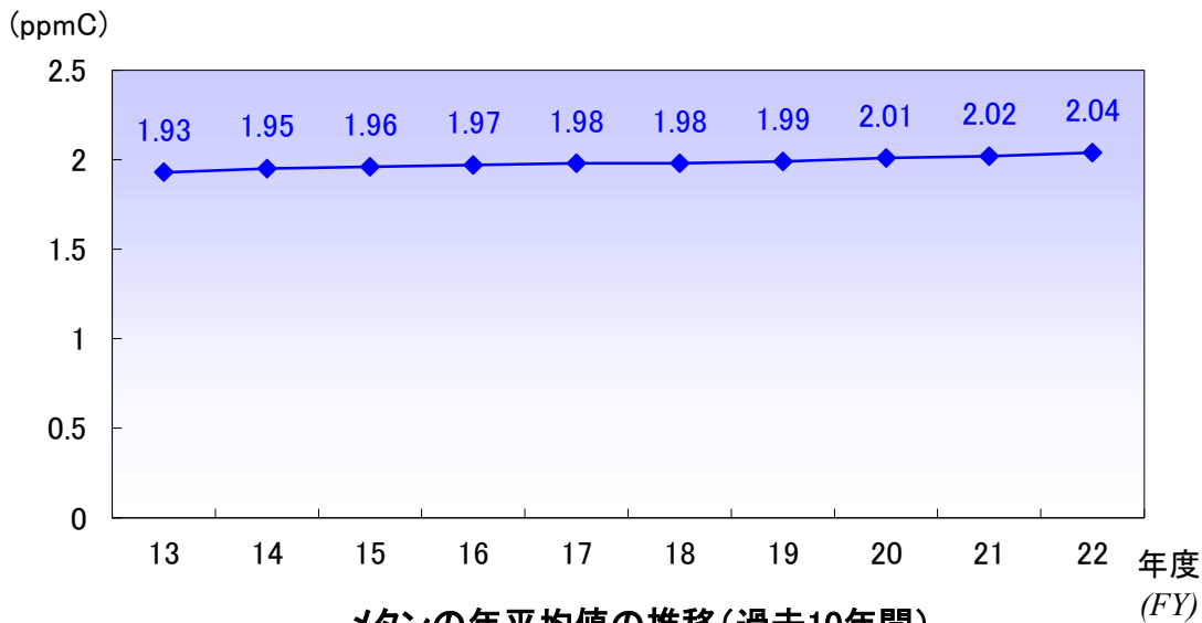
メタンの年平均値の推移(過去10年間) (Trend of Annual Average CH_4 Concentration(The Last Ten Years))
