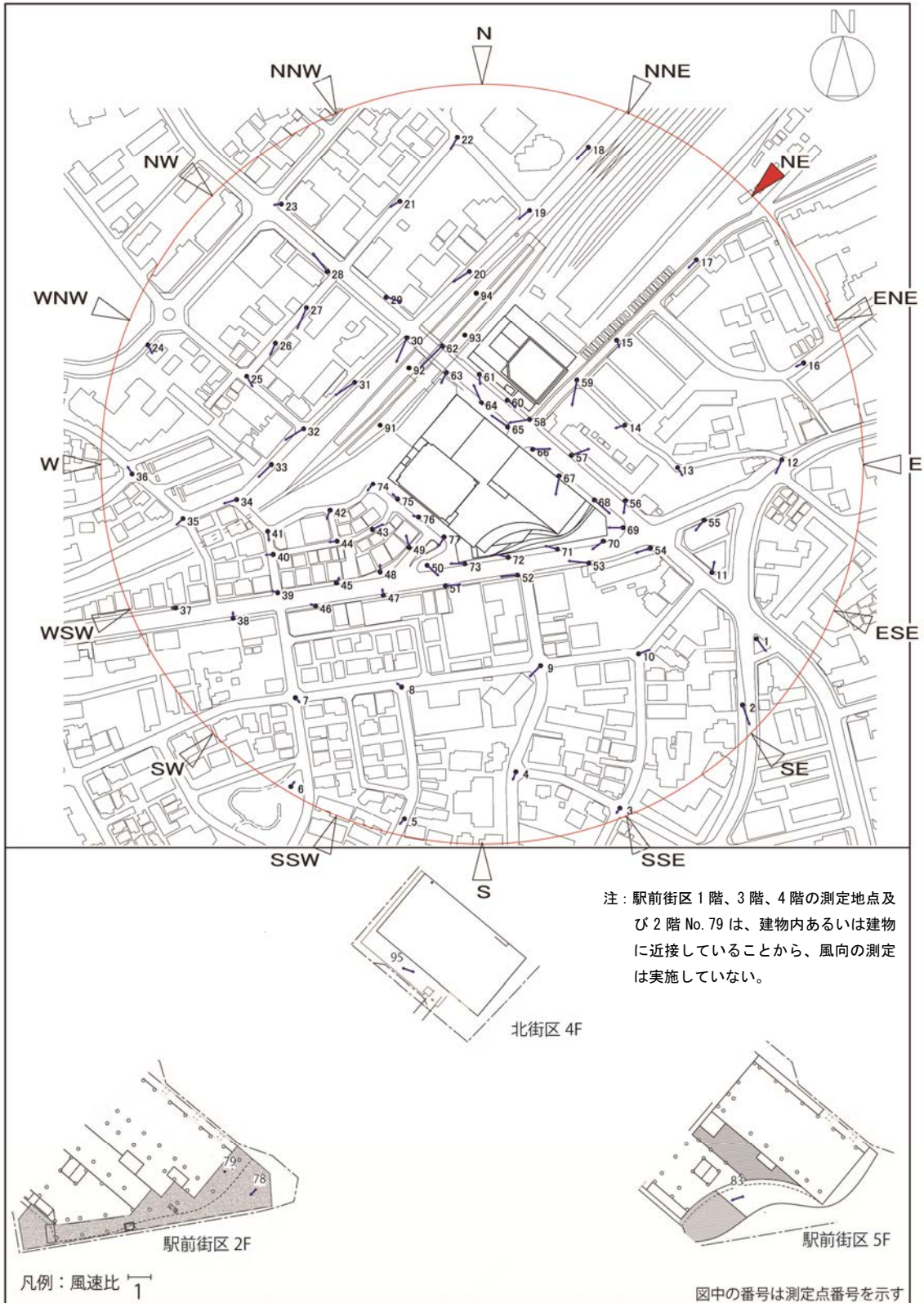
図 8-5 (3) 風速比ベクトル図 (建設後対策後：北東)
