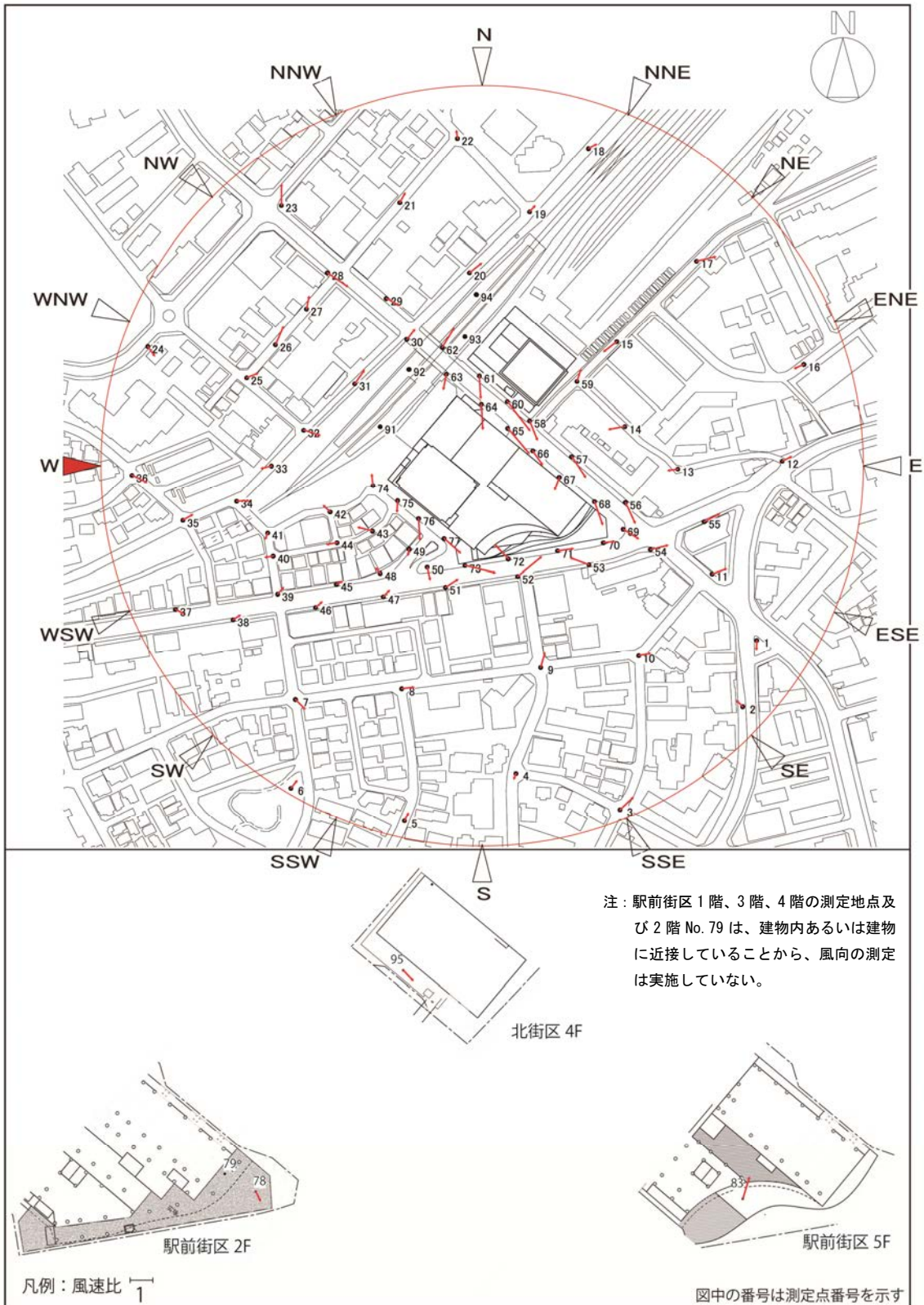
図 8-4 (13) 風速比ベクトル図 (建設後：西)
