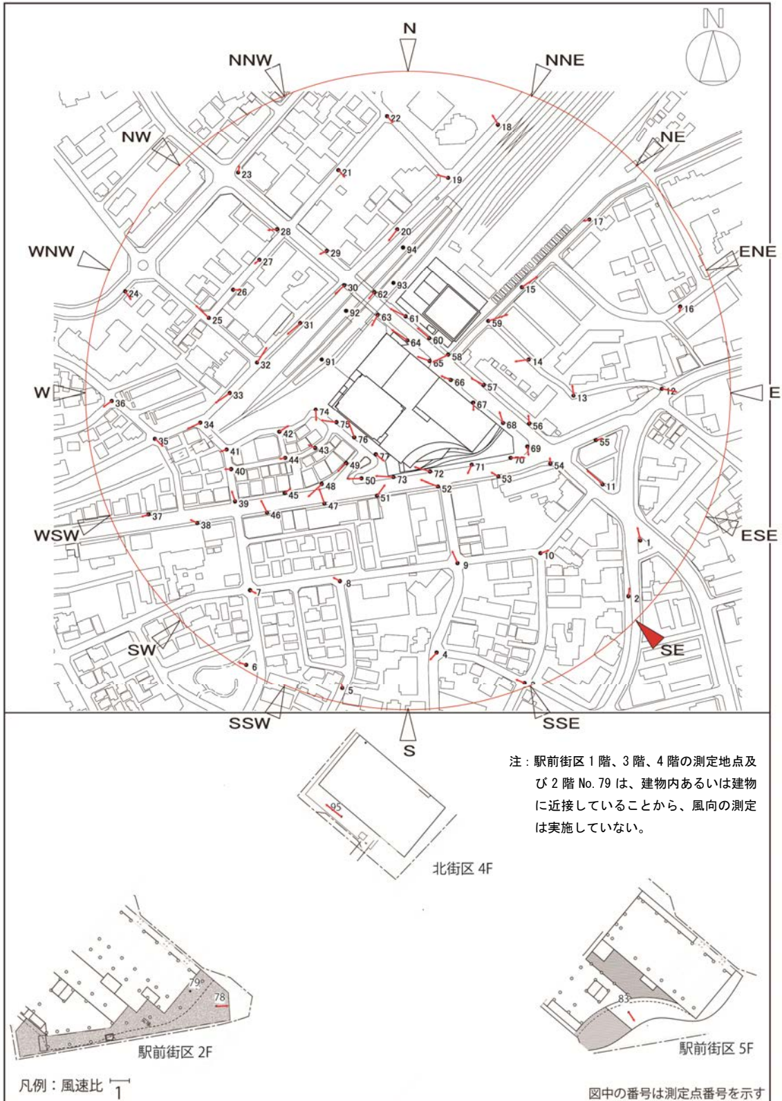
図 8-4 (7) 風速比ベクトル図 (建設後：南東)
