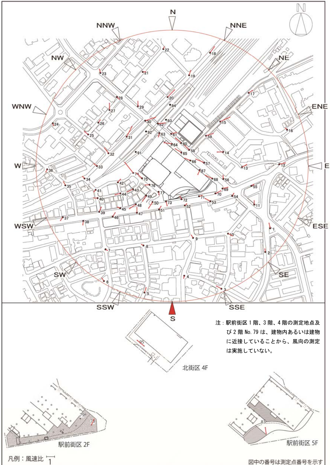
図 8-4 (9) 風速比ベクトル図 (建設後：南)
