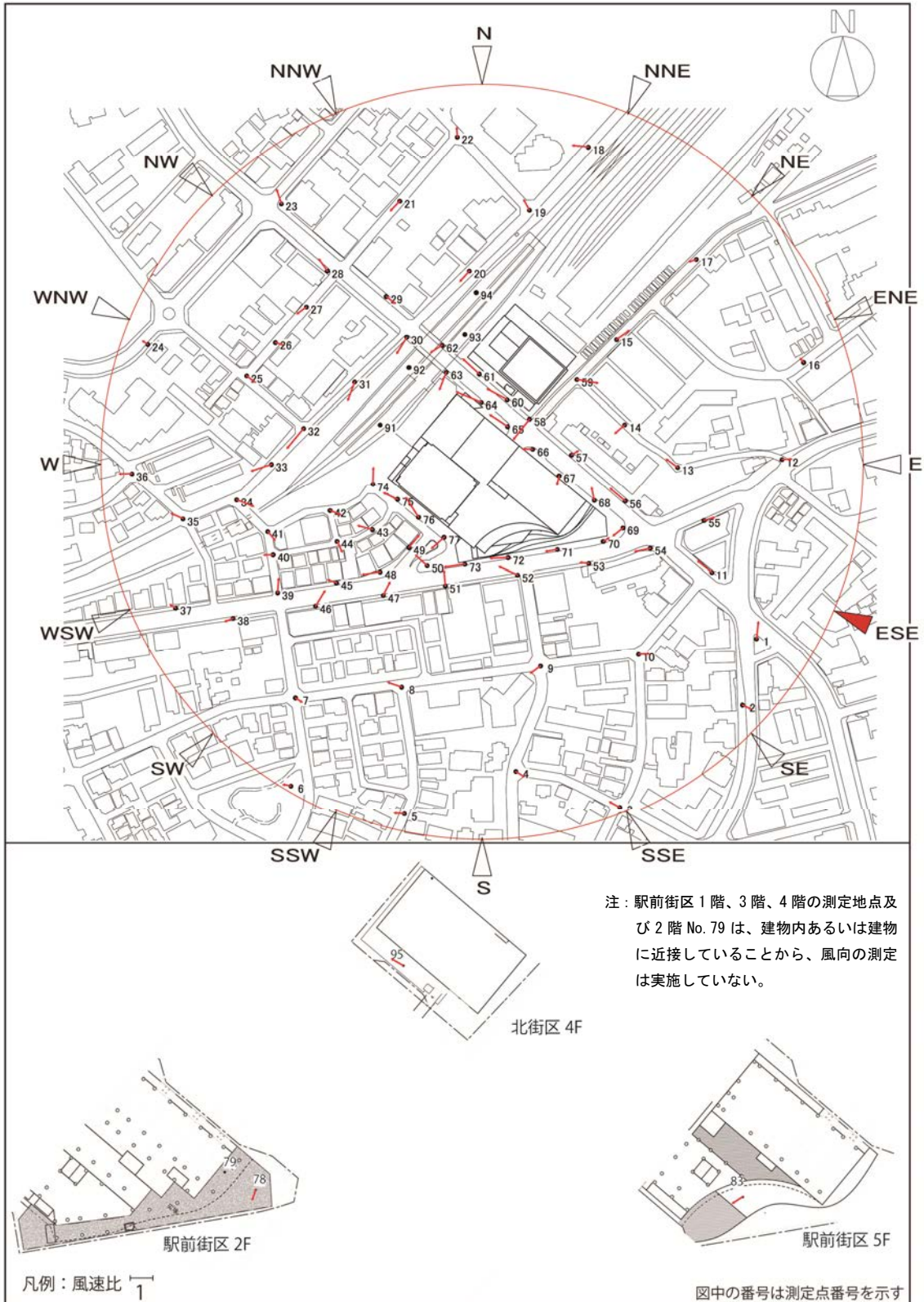
図 8-4 (6) 風速比ベクトル図 (建設後：東南東)
