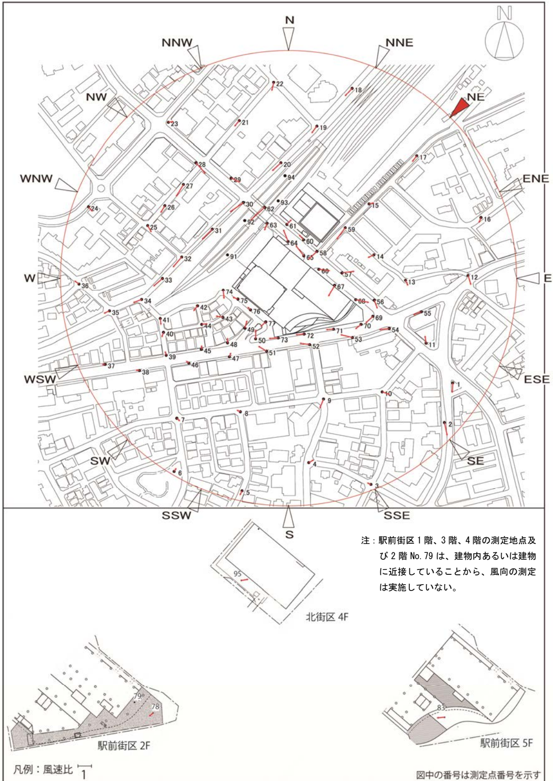
図 8-4 (3) 風速比ベクトル図 (建設後：北東)
