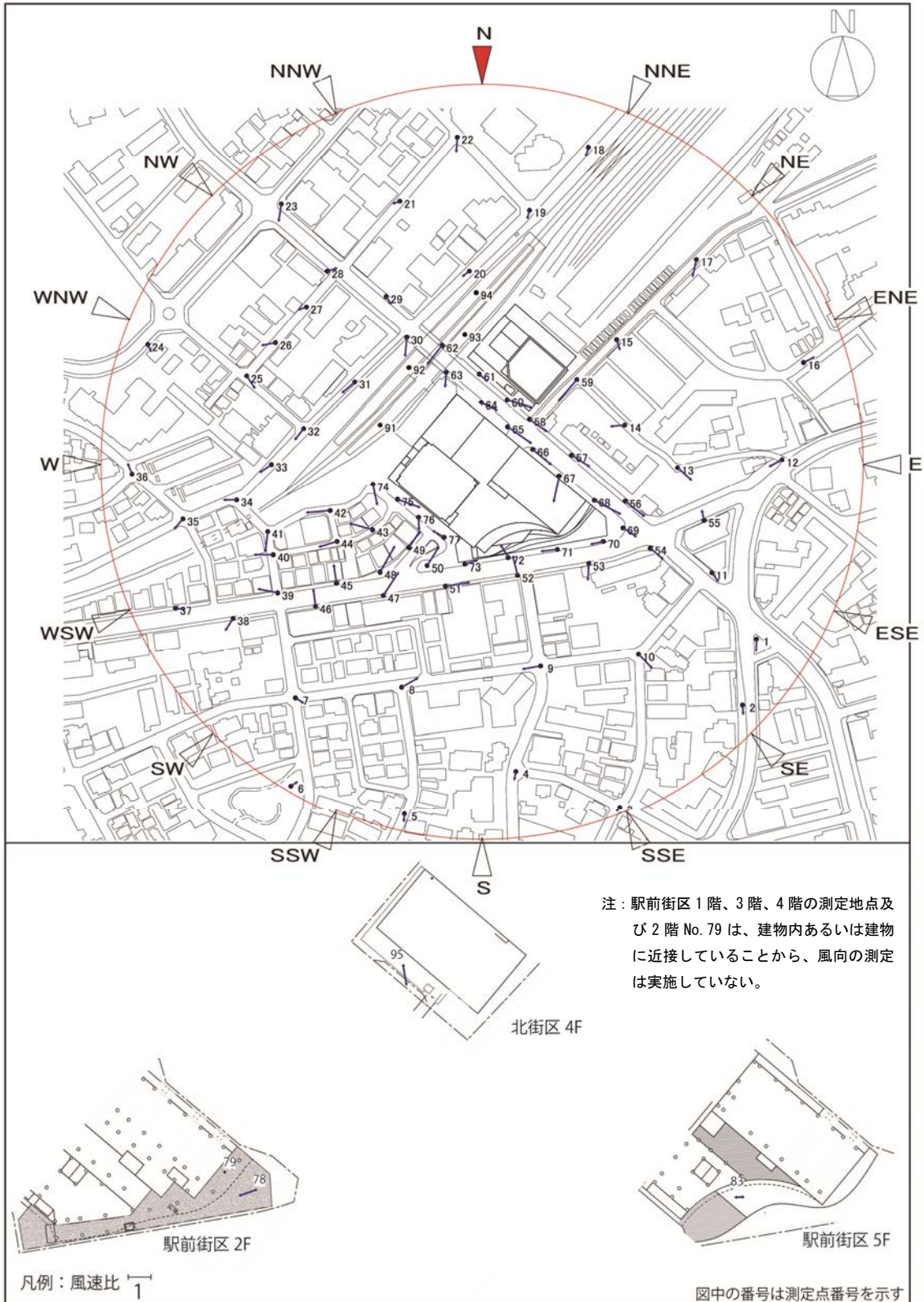
図 8-5 (1) 風速比ベクトル図 (建設後対策後：北)
