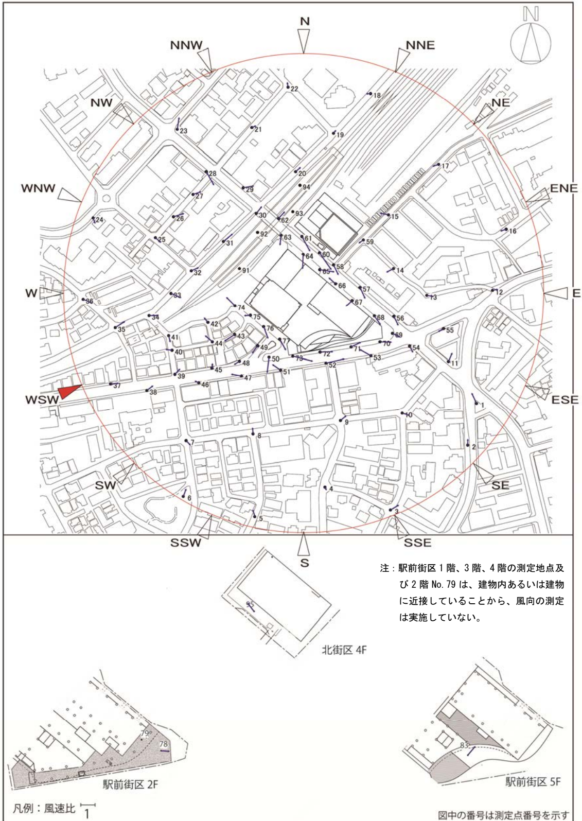
図 8-5 (12) 風速比ベクトル図（建設後対策後：西南西）
