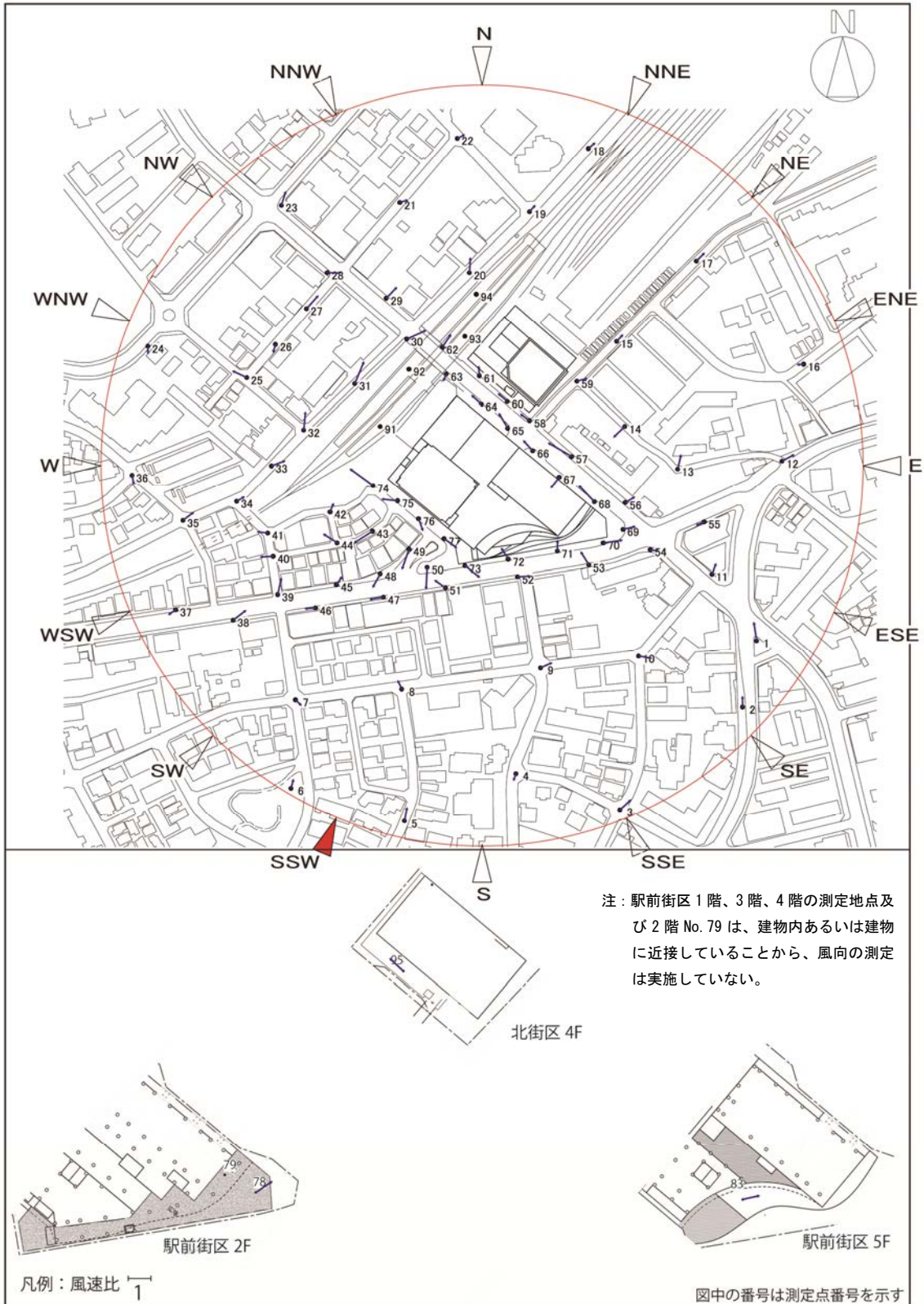
図 8-5 (10) 風速比ベクトル図（建設後対策後：南南西）
