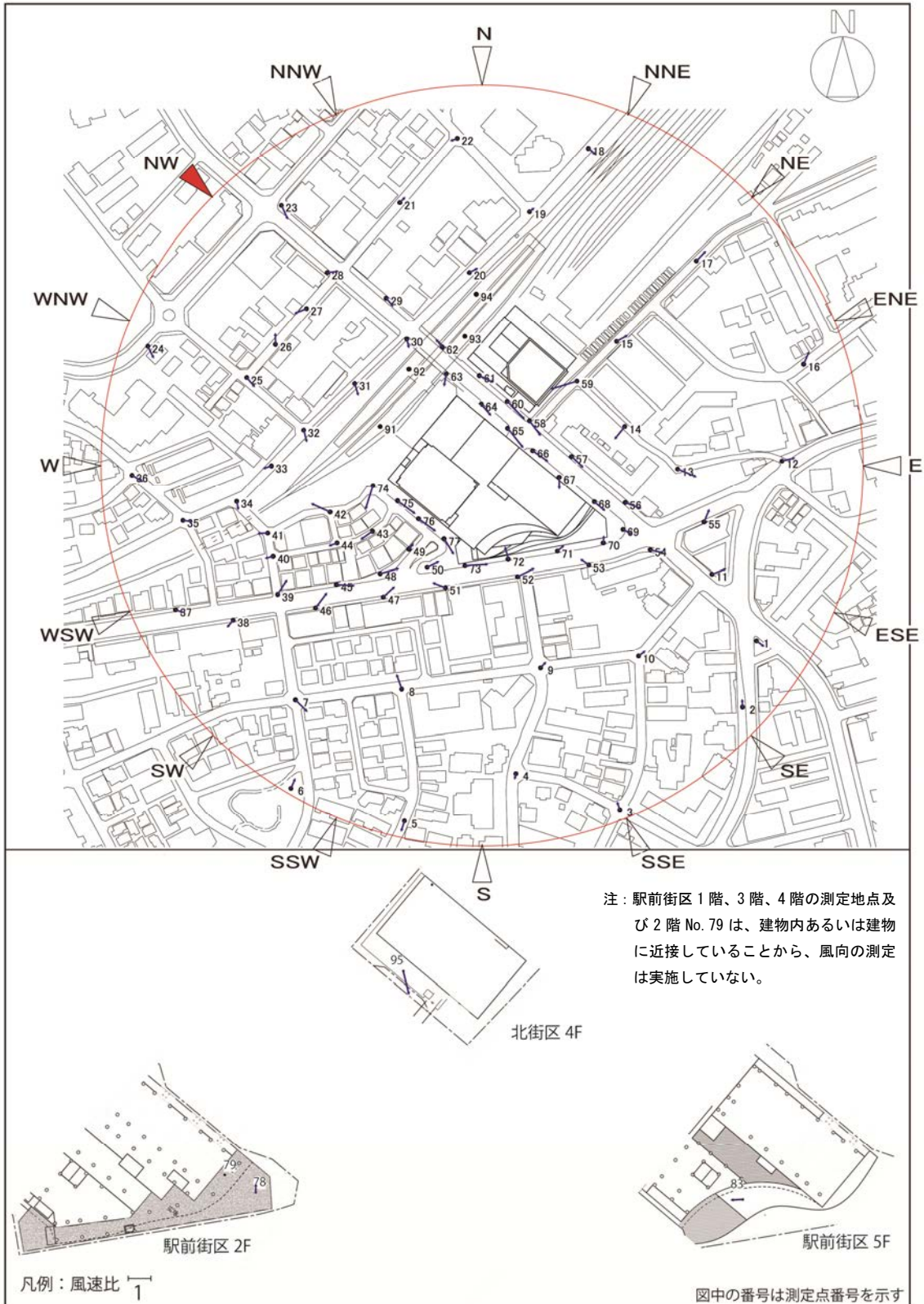
図 8-5 (15) 風速比ベクトル図 (建設後対策後：北西)
