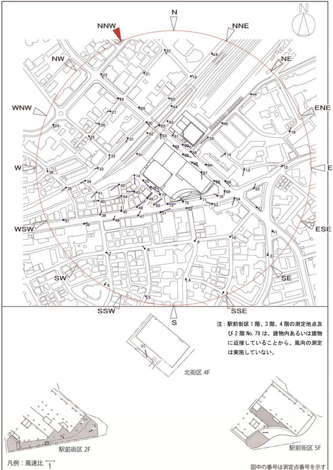
図 8-5 (16) 風速比ベクトル図（建設後対策後：北北西）
