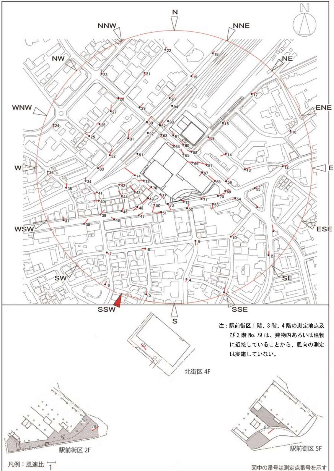
図 8-4 (10) 風速比ベクトル図 (建設後：南南西)
