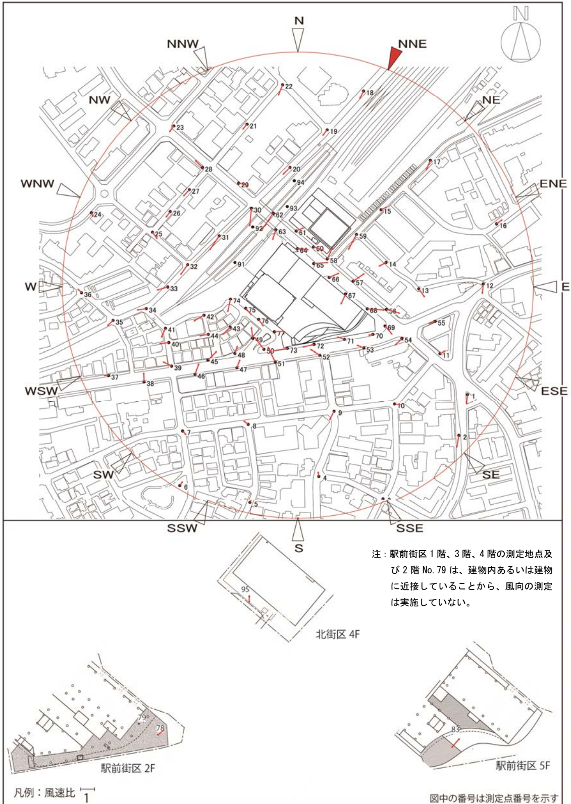
図 8-4 (2) 風速比ベクトル図 (建設後：北北東)
