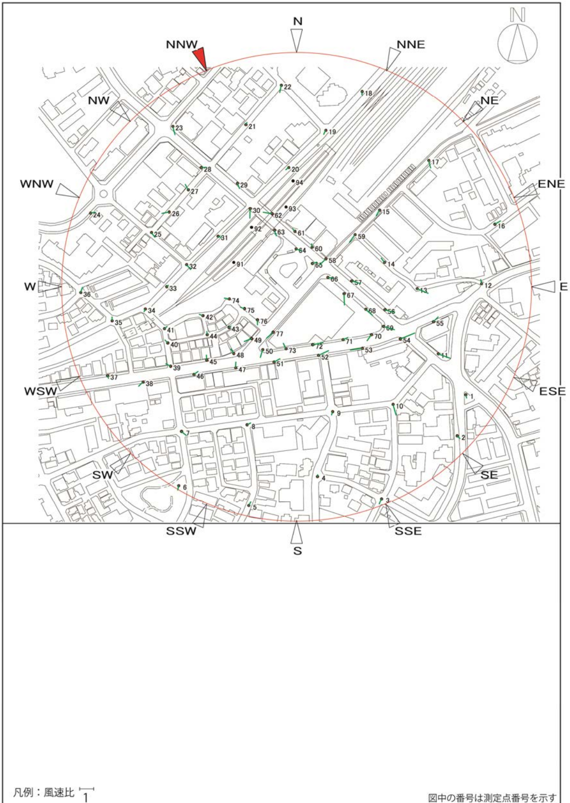
図 8-3 (16) 風速比ベクトル図 (建設前：北北西)
