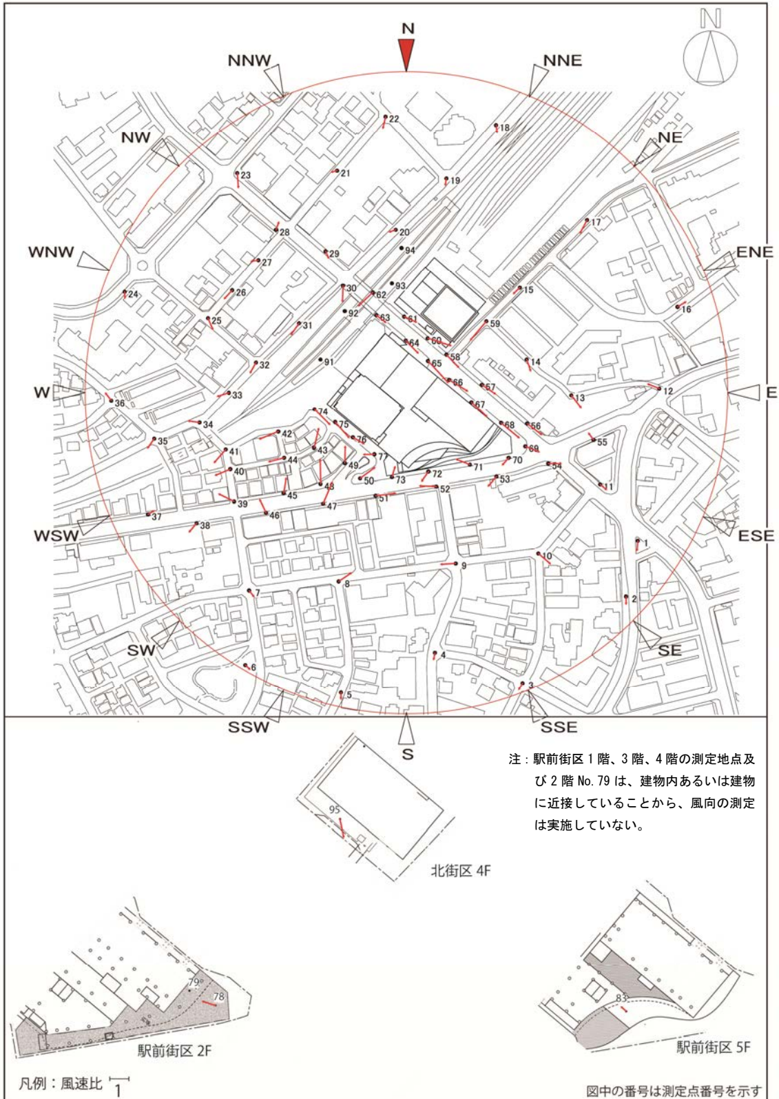
図 8-4 (1) 風速比ベクトル図 (建設後：北)
