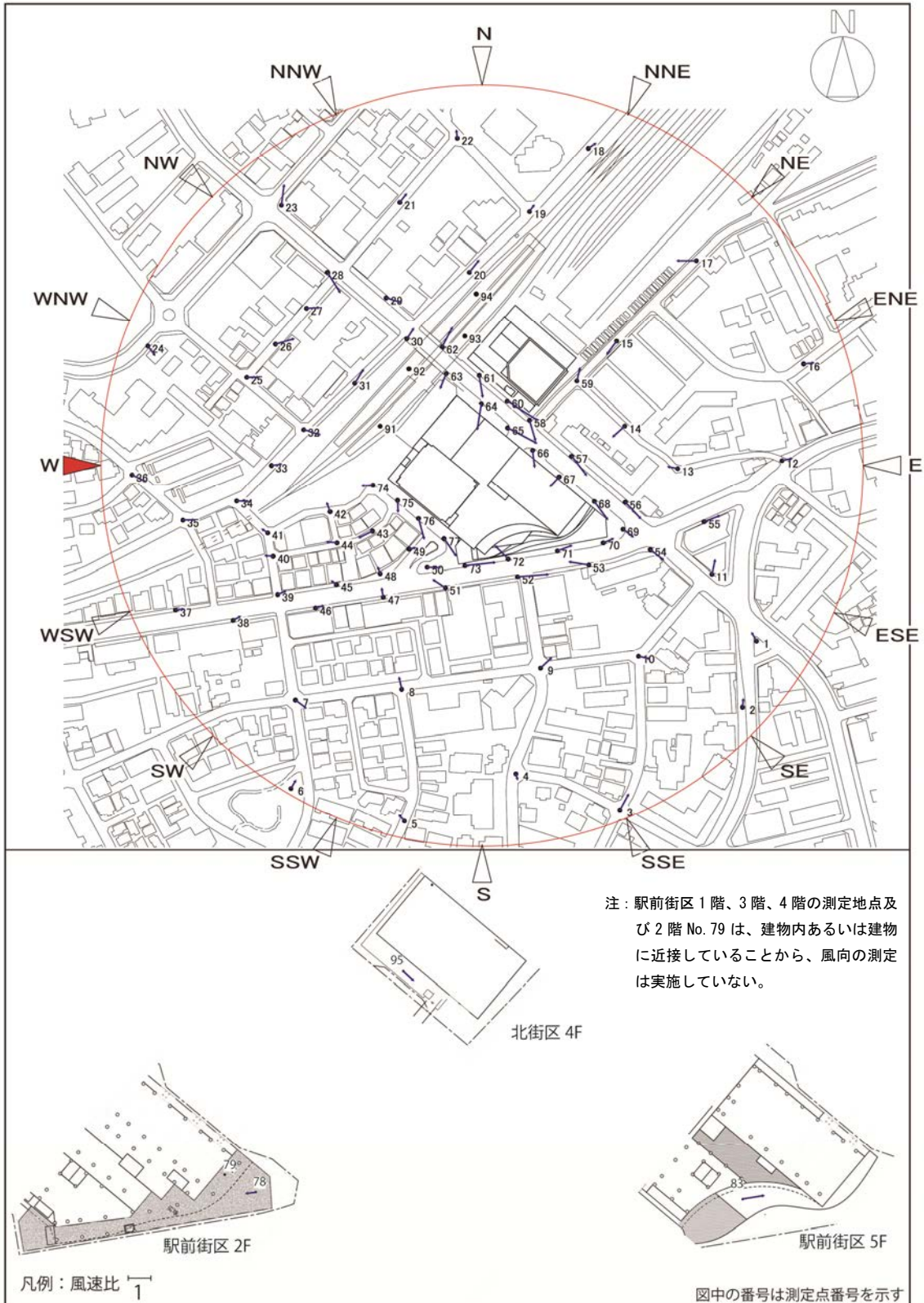
図 8-5 (13) 風速比ベクトル図 (建設後対策後：西)
