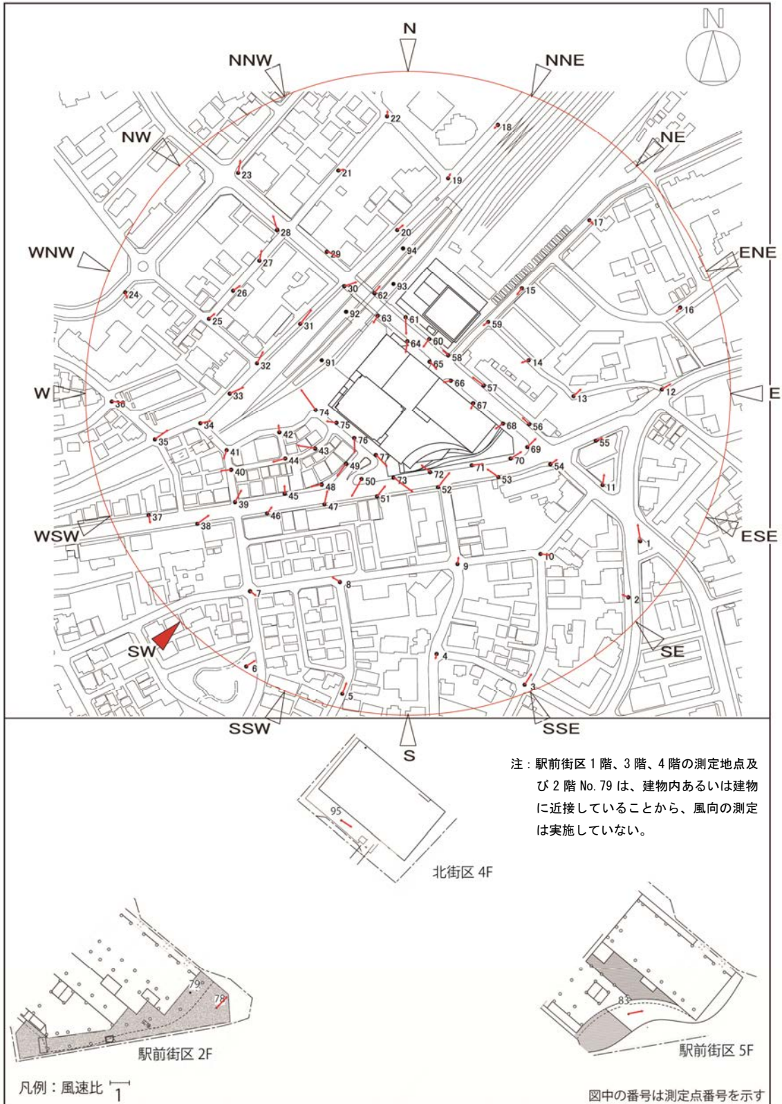
図 8-4 (11) 風速比ベクトル図 (建設後：南西)
