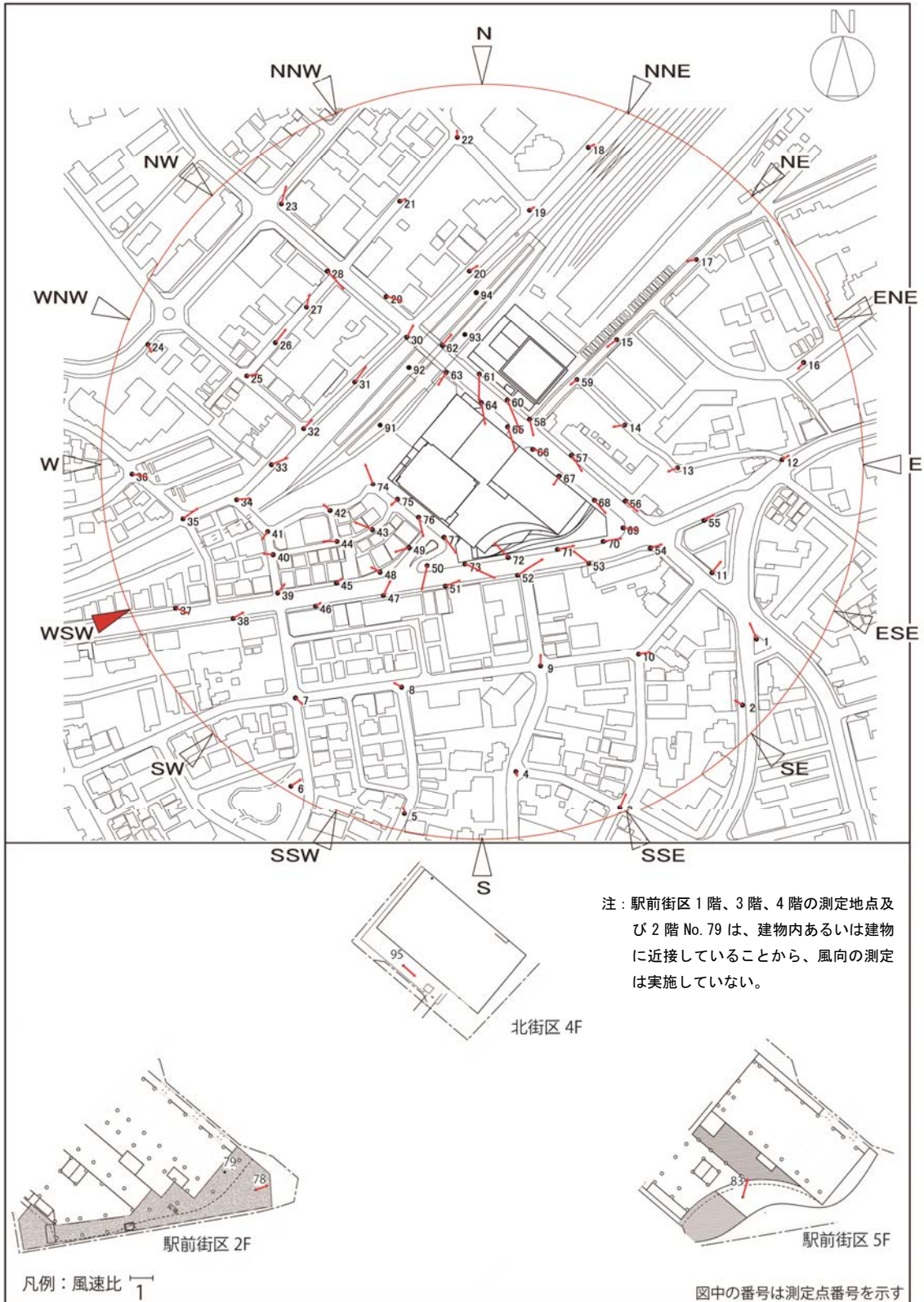
図 8-4 (12) 風速比ベクトル図 (建設後：西南西)
