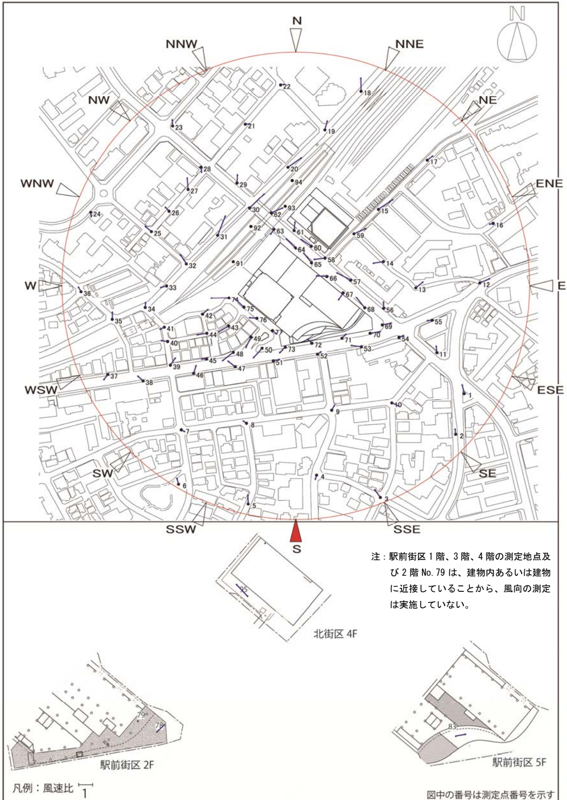
図 8-5(9) 風速比ベクトル図（建設後対策後：南）
