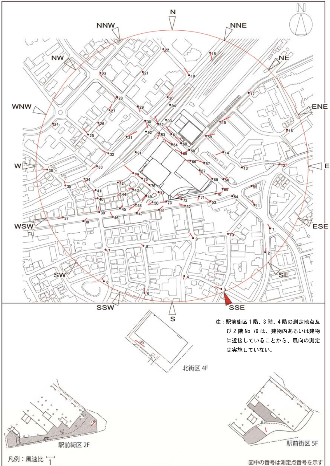
図 8-4 (8) 風速比ベクトル図 (建設後：南南東)
