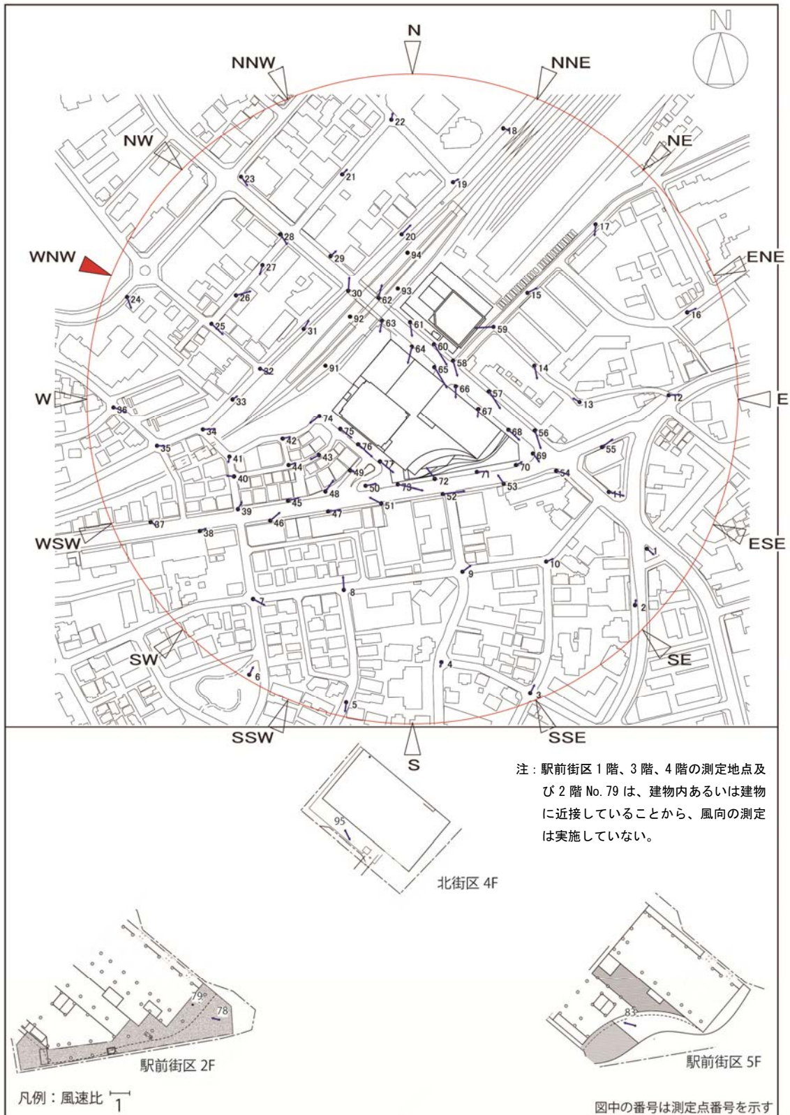
図 8-5 (14) 風速比ベクトル図（建設後対策後：西北西）
