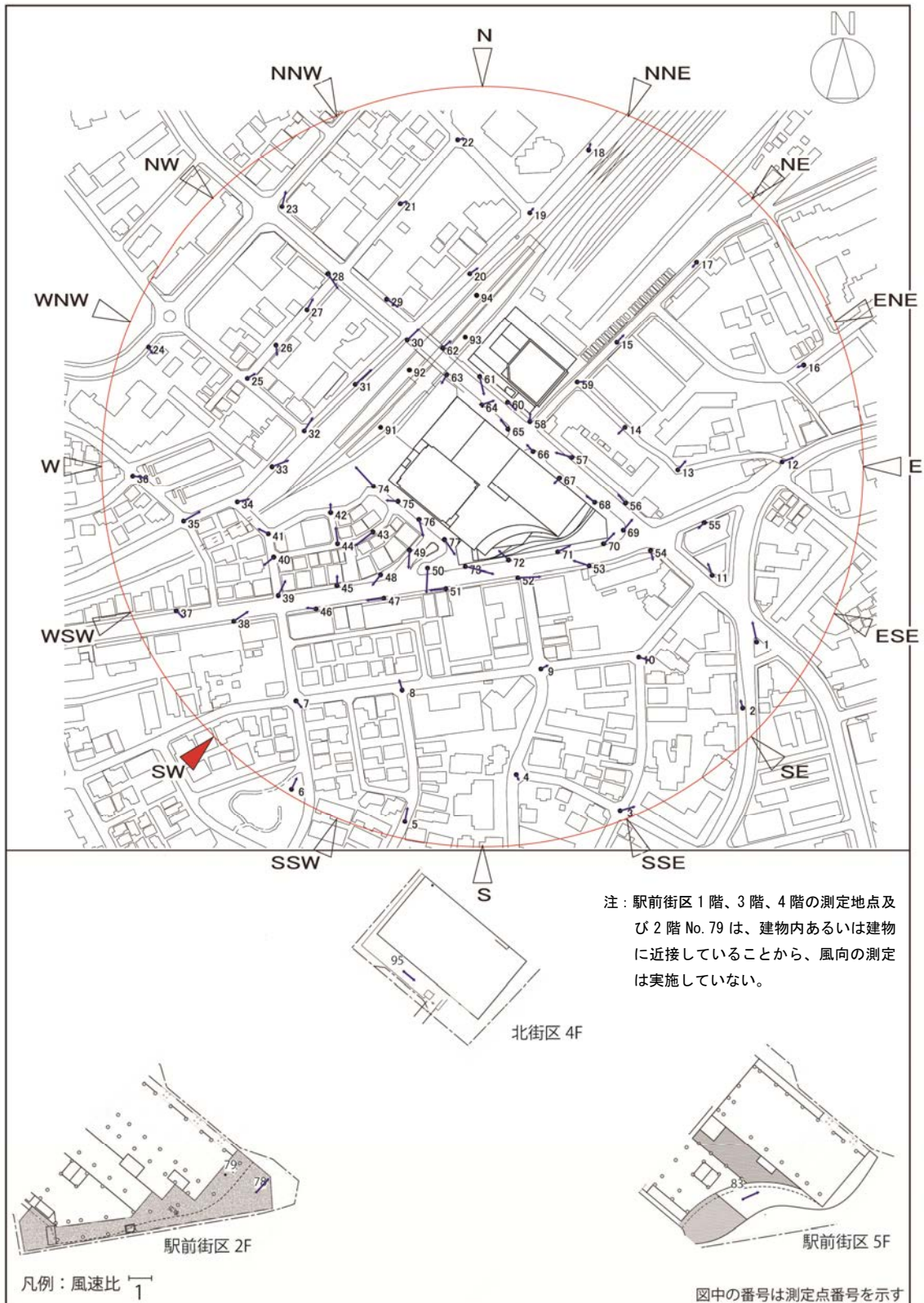
図 8-5 (11) 風速比ベクトル図 (建設後対策後：南西)
