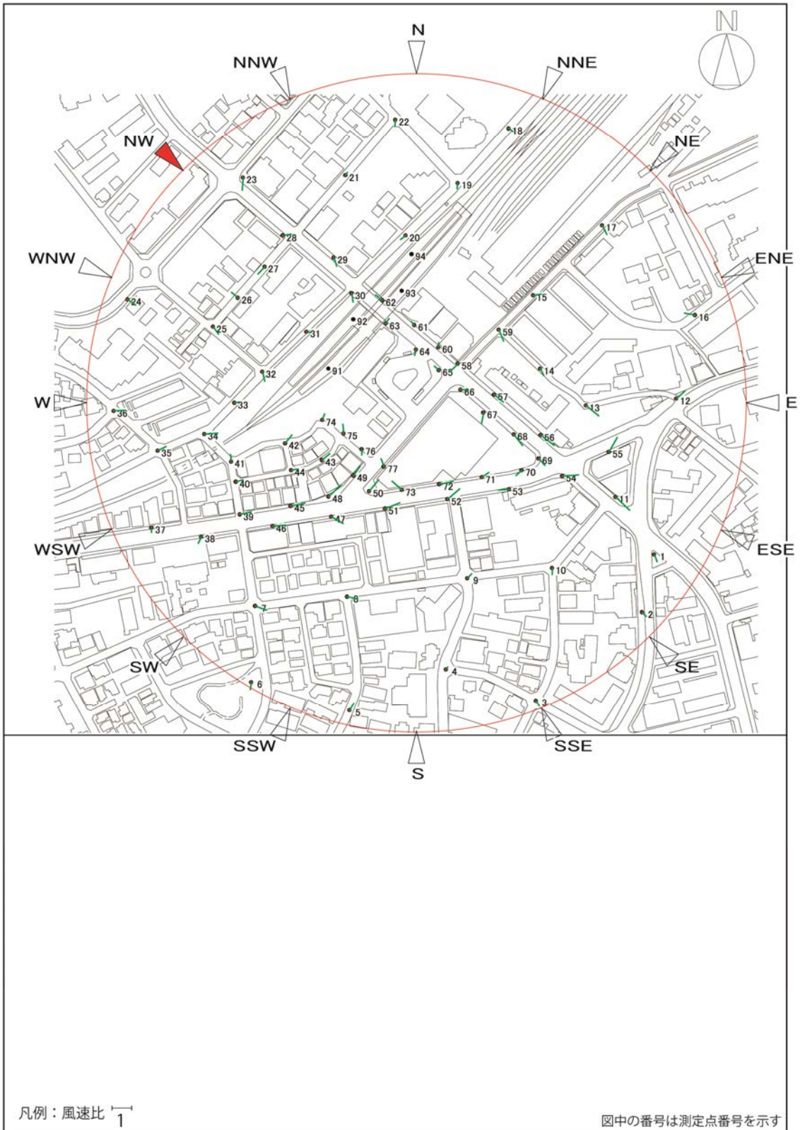
図 8-3 (15) 風速比ベクトル図 (建設前：北西)
