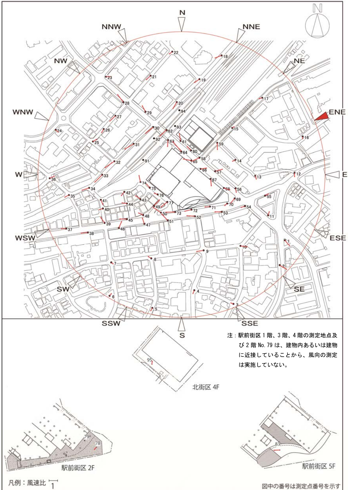
図 8-4 (4) 風速比ベクトル図 (建設後：東北東)
