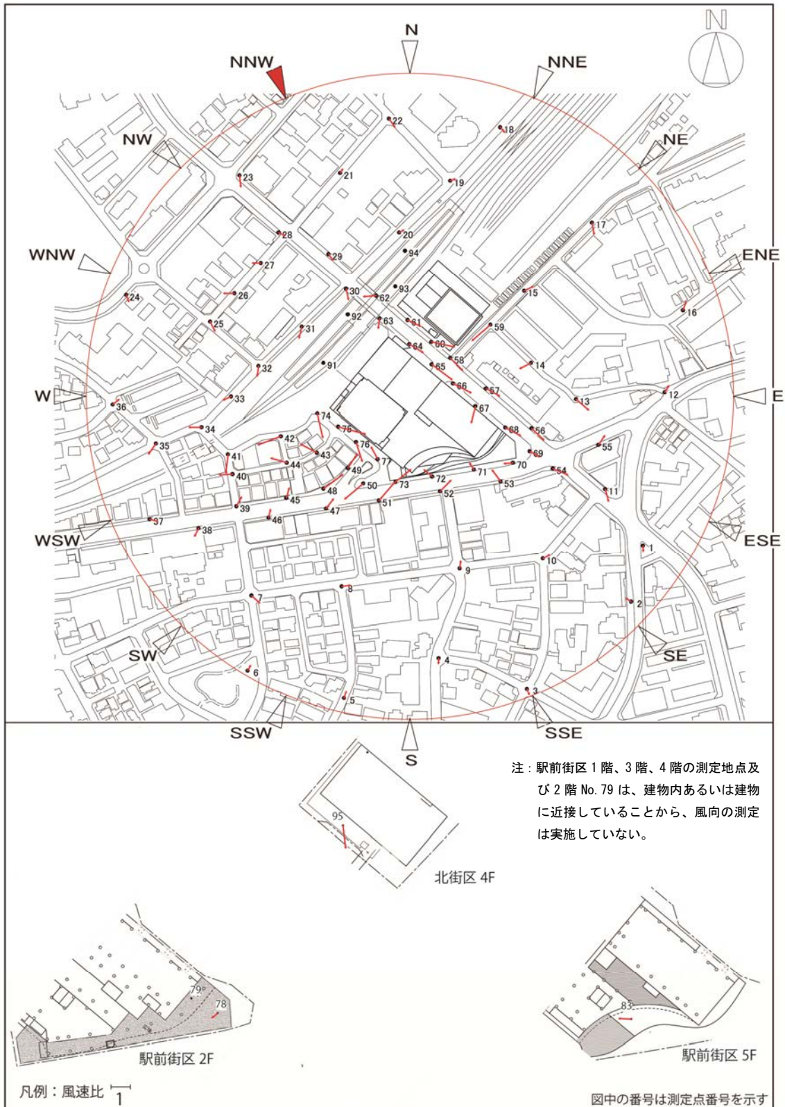
図 8-4 (16) 風速比ベクトル図 (建設後：北北西)
