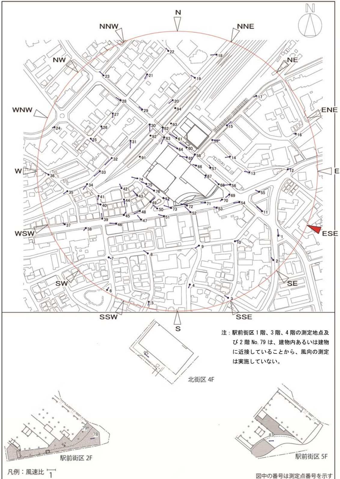
図 8-5 (6) 風速比ベクトル図 (建設後対策後：東南東)
