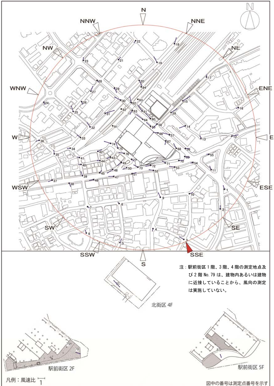
図 8-5 (8) 風速比ベクトル図 (建設後対策後：南南東)
