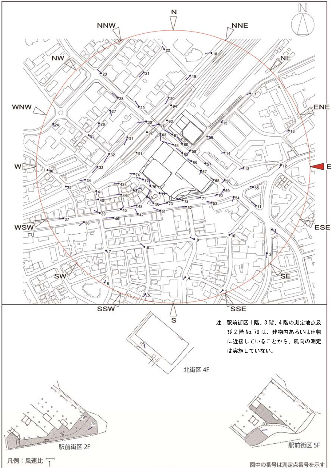
図 8-5 (5) 風速比ベクトル図（建設後対策後：東）
