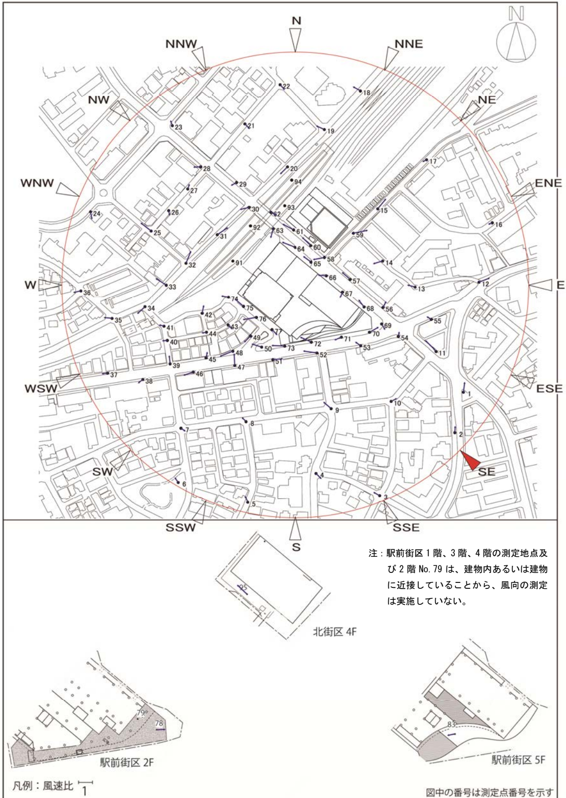
図 8-5 (7) 風速比ベクトル図 (建設後対策後：南東)
