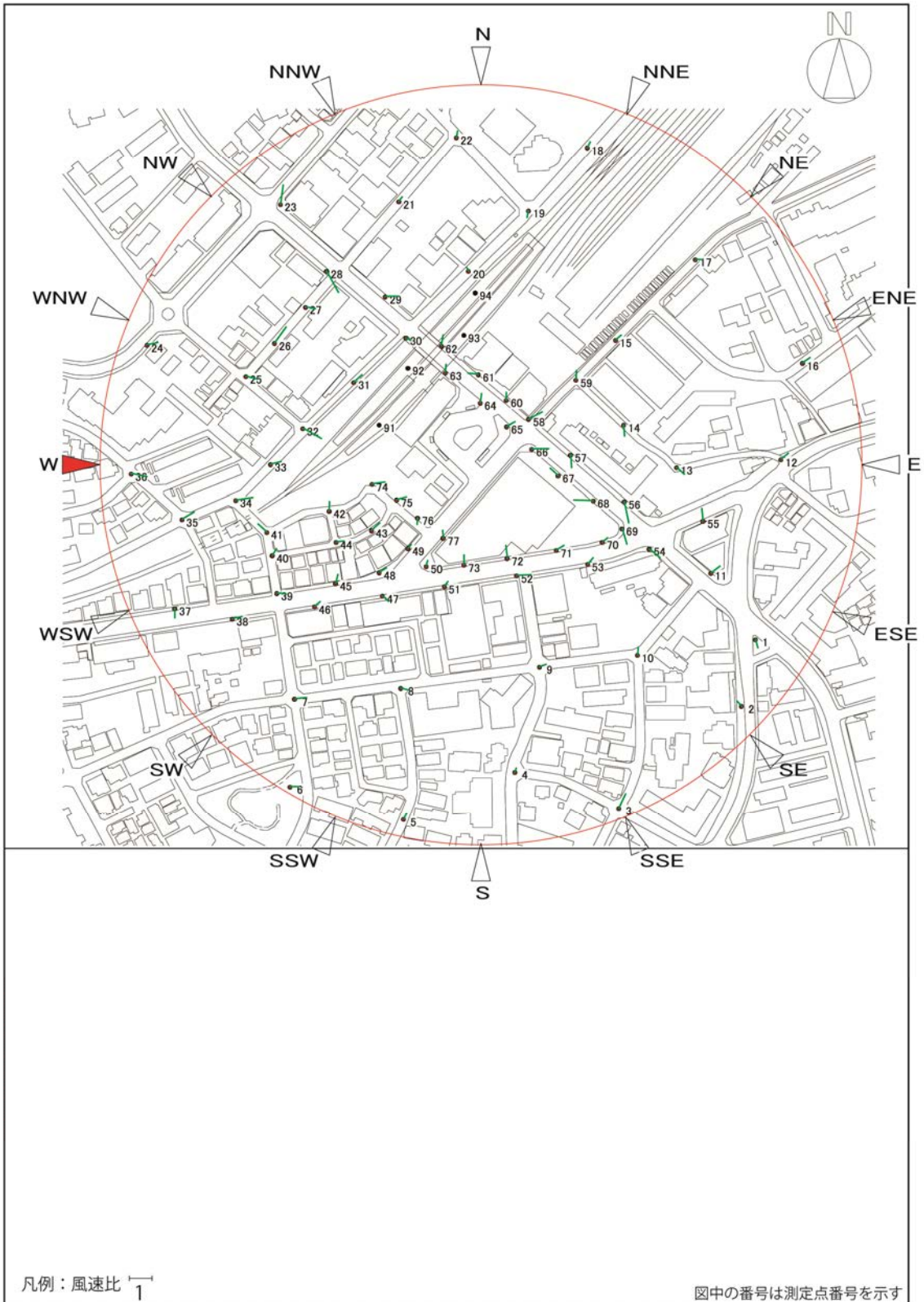
図 8-3 (13) 風速比ベクトル図 (建設前：西)
