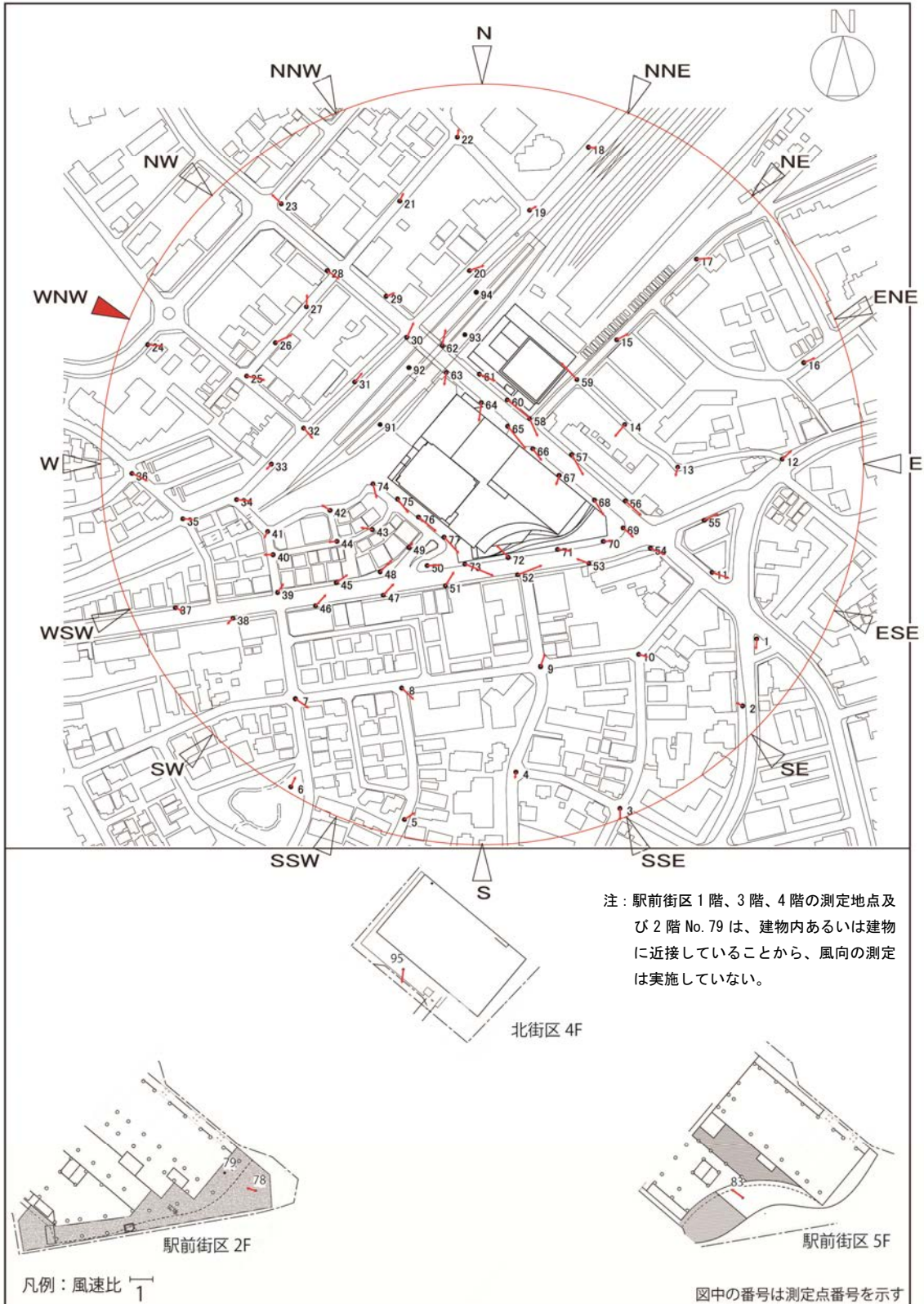
図 8-4 (14) 風速比ベクトル図 (建設後：西北西)
