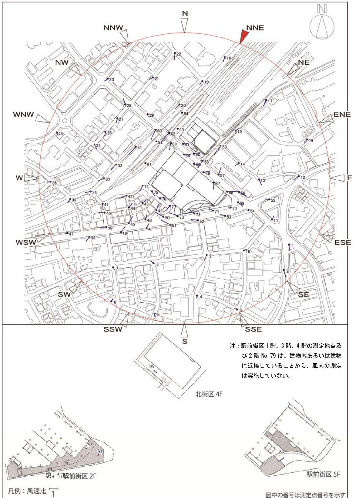
図 8-5 (2) 風速比ベクトル図 (建設後対策後：北北東)
