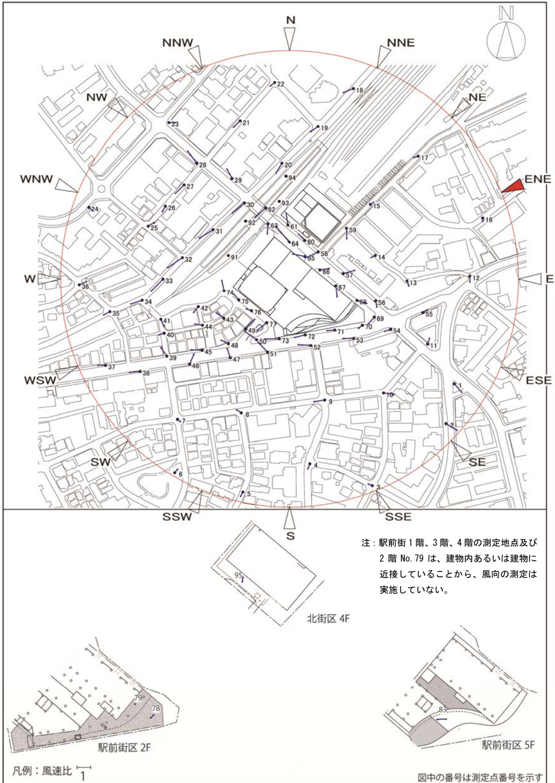
図 8-5 (4) 風速比ベクトル図 (建設後対策後：東北東)
