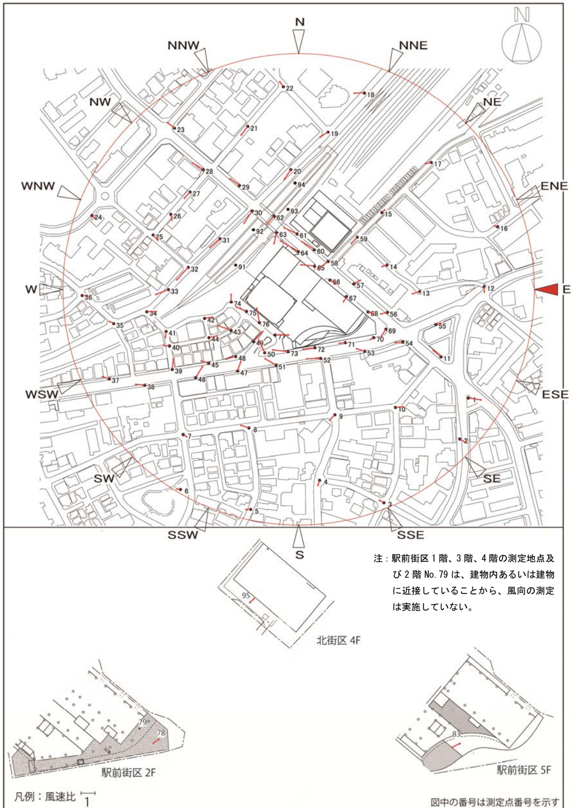
図 8-4 (5) 風速比ベクトル図 (建設後：東)
