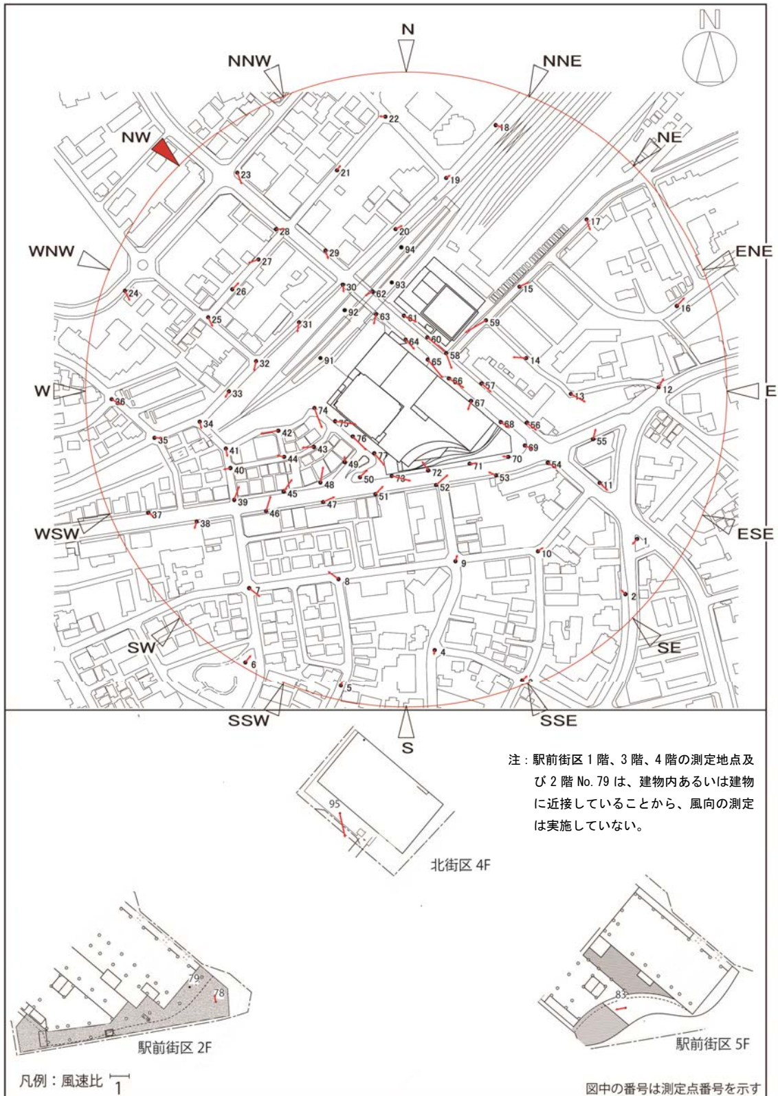
図 8-4 (15) 風速比ベクトル図 (建設後：北西)
