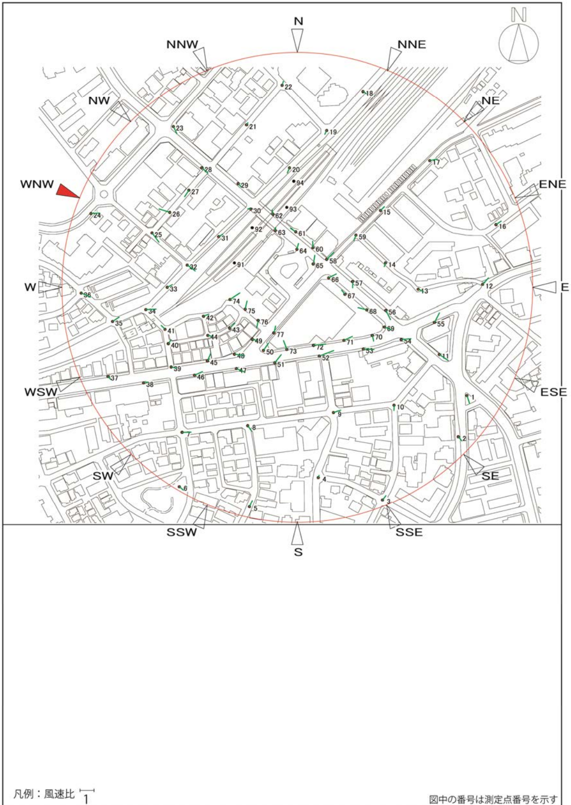
図 8-3 (14) 風速比ベクトル図 (建設前：西北西)
