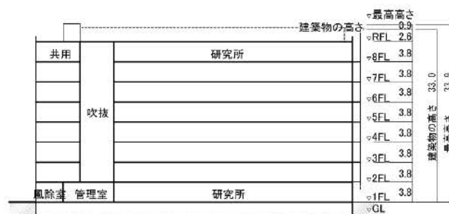
B-B' 断面図
