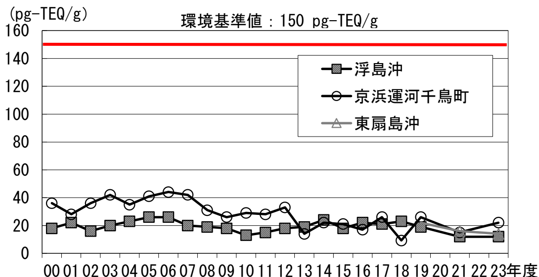
図26 ダイオキシン類濃度の経年推移 (3地点) (海域・底質)
