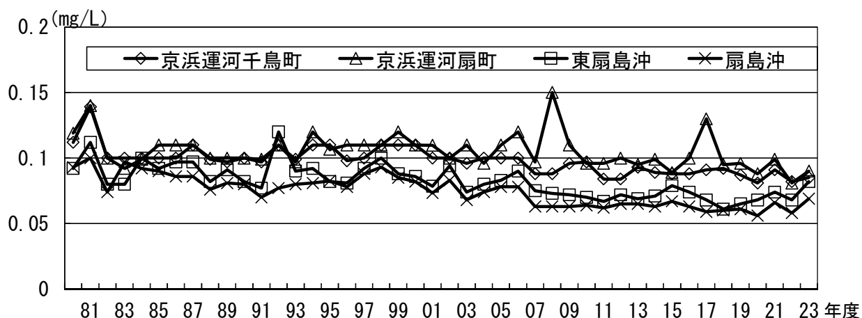
図 24 海域の全磷の年間平均値（全層）の経年推移
