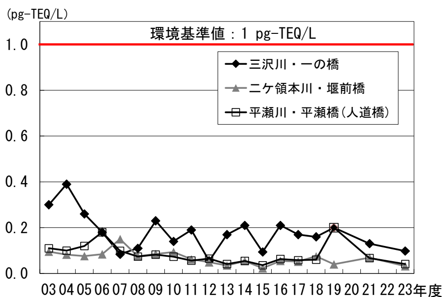
図 19 ダイオキシン類濃度の経年推移(3 地点) (河川・水質)
