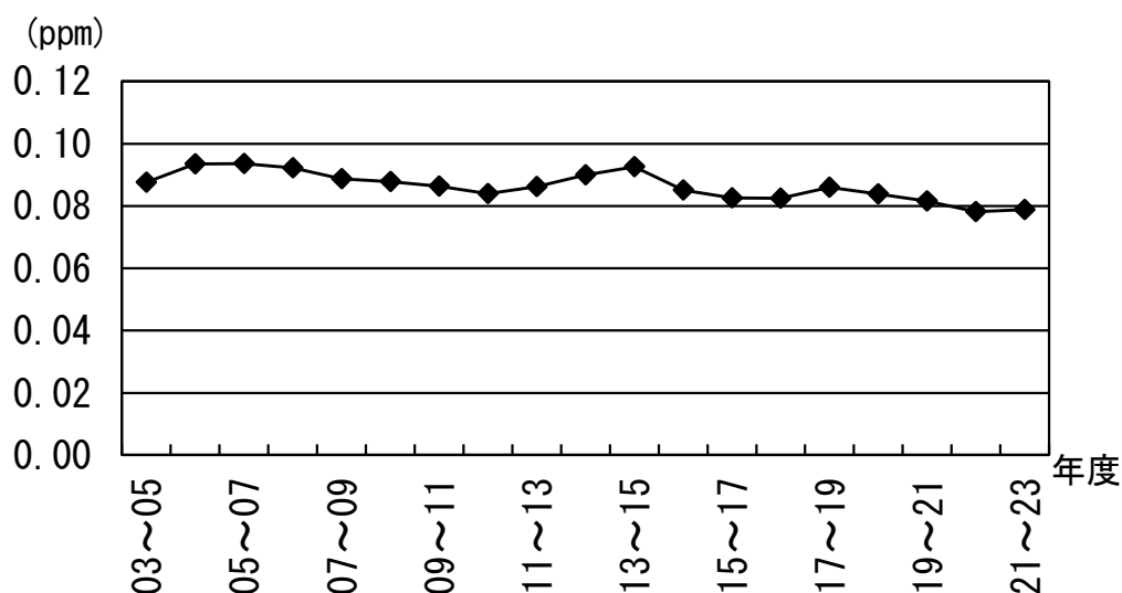
図8 光化学オキシダント濃度の長期的な改善傾向を評価するための指標 （8時間値の日最高値の年間99パーセンタイル値の3年平均値）の経年推移
