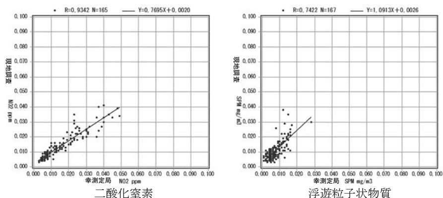
図 1.1.1-4(1) 現地調査結果と幸測定局の大気質濃度相関分析結果（冬季）
