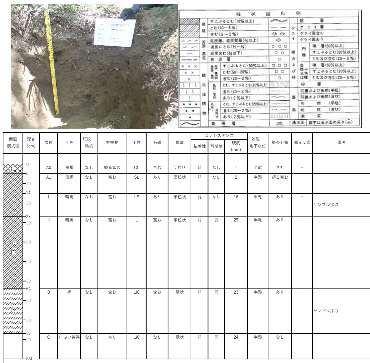
図 1.5.1-1(1) 基本断面調査結果 (地点 A)
