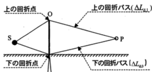
図 1.2.1-3 音源・受音点と障害物の関係
