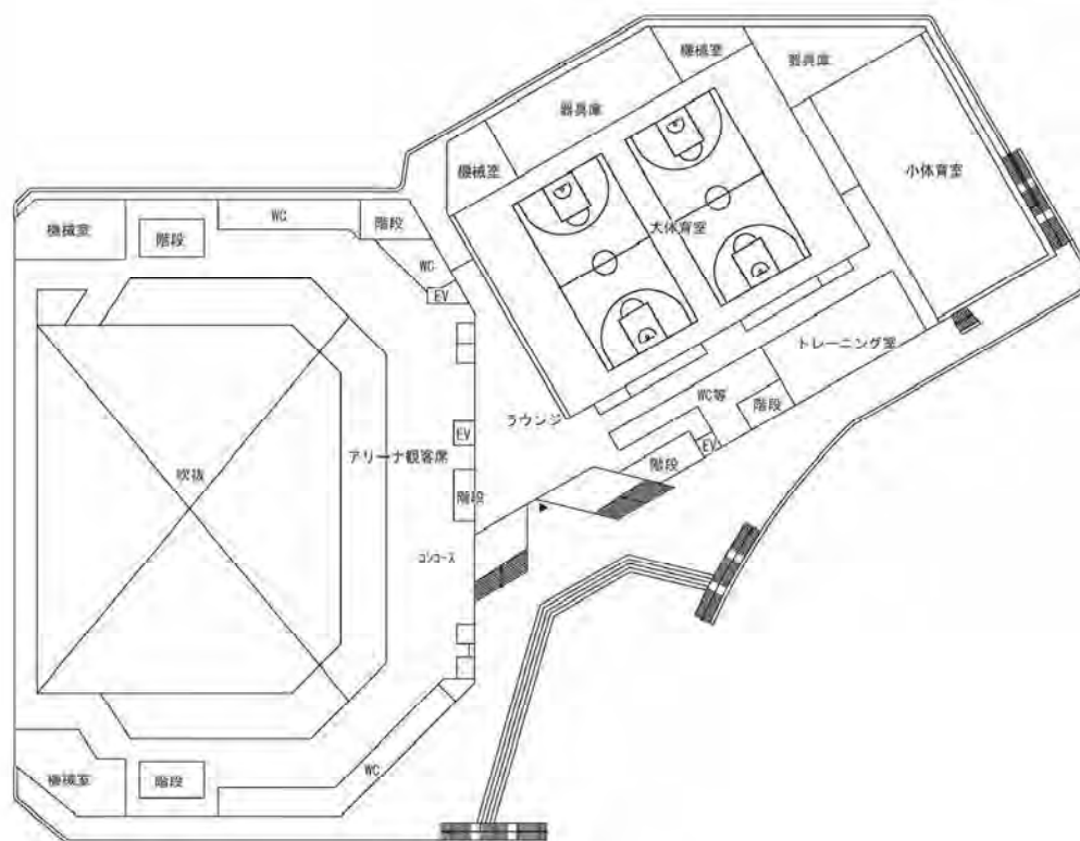
2階平面図
