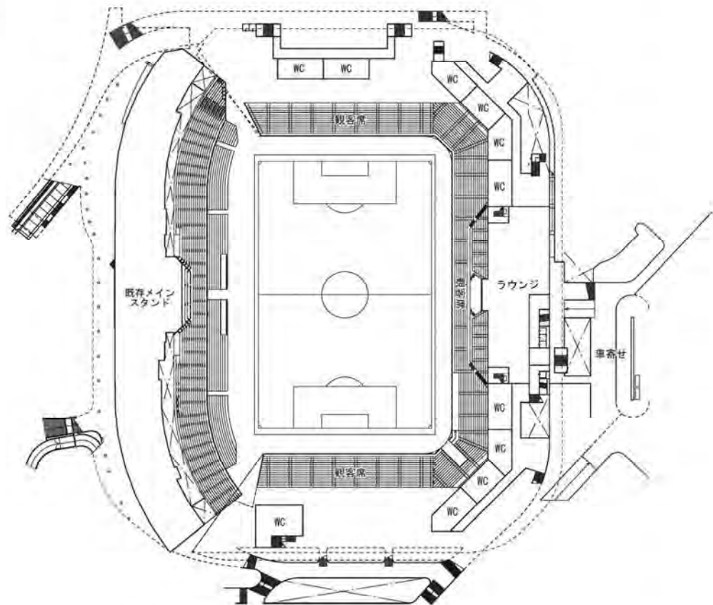
2F平面図
