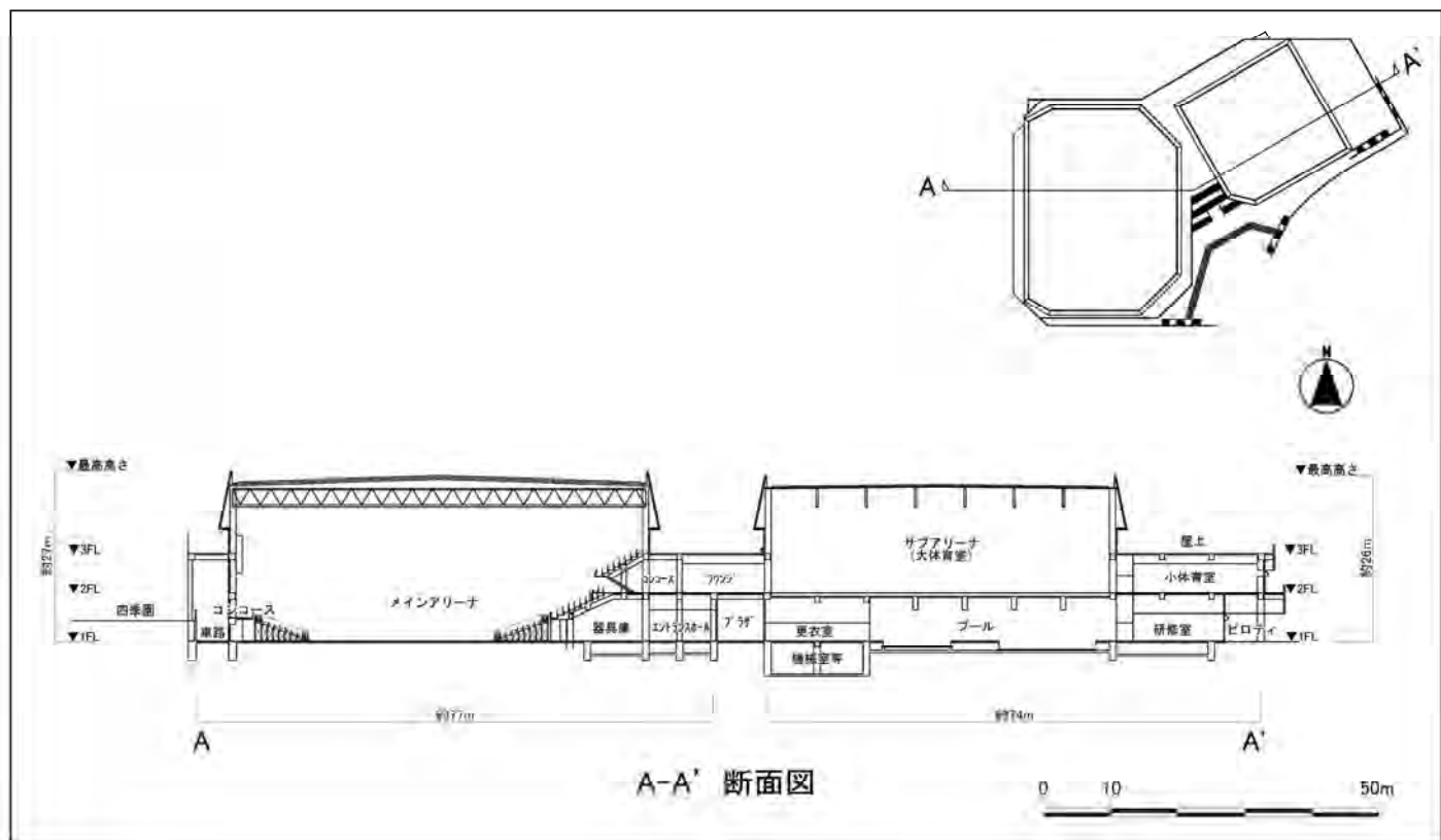
図 1-10(11) (新)とどろきアリーナ・スポーツセンター断面図
