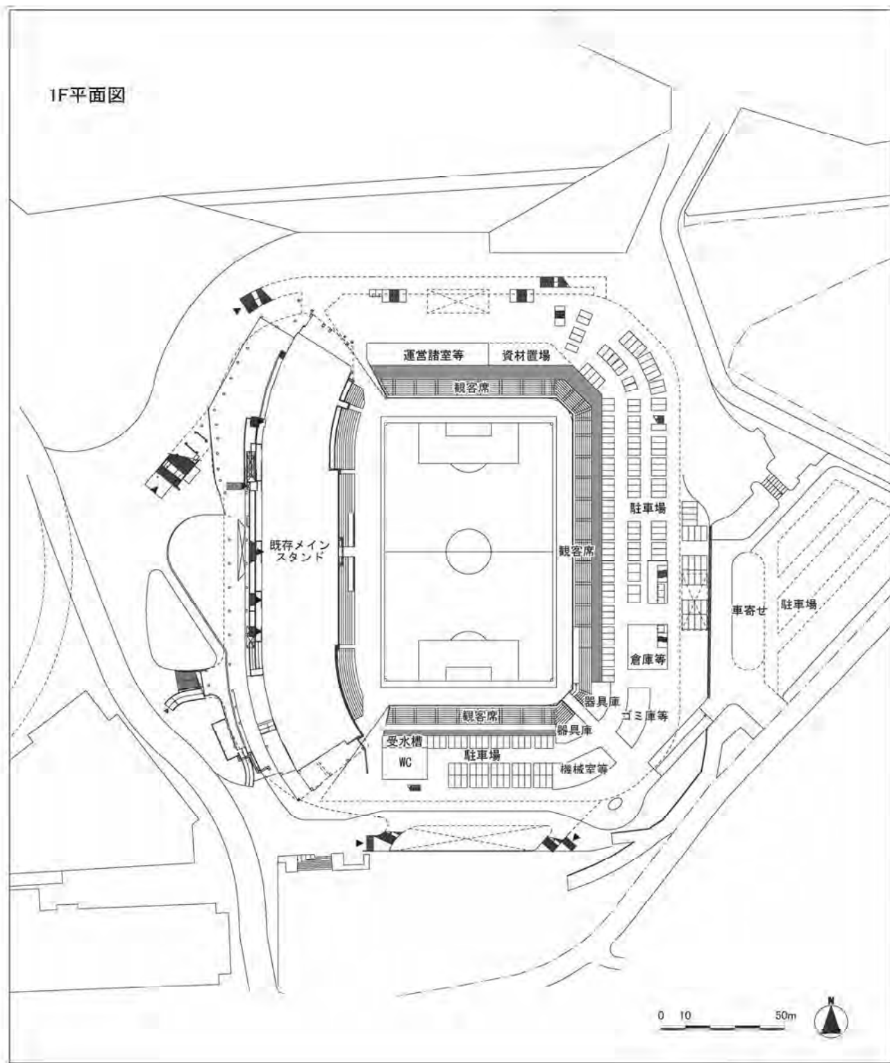
図 1-10(1) 球技専用スタジアム平面図 (1F)
