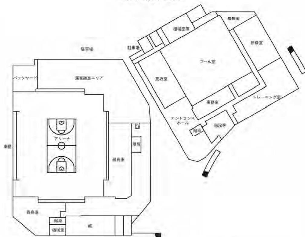
1階平面図
