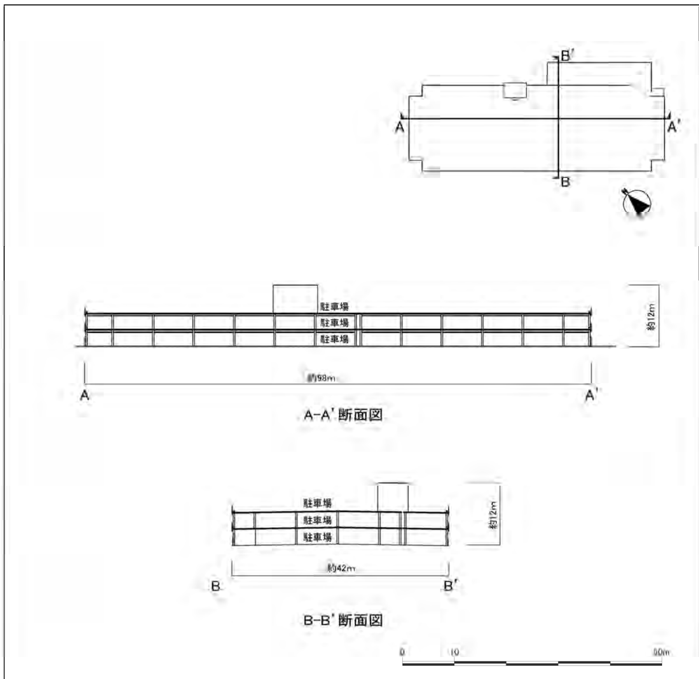
図 1-10(18) 西側立体駐車場 断面図
