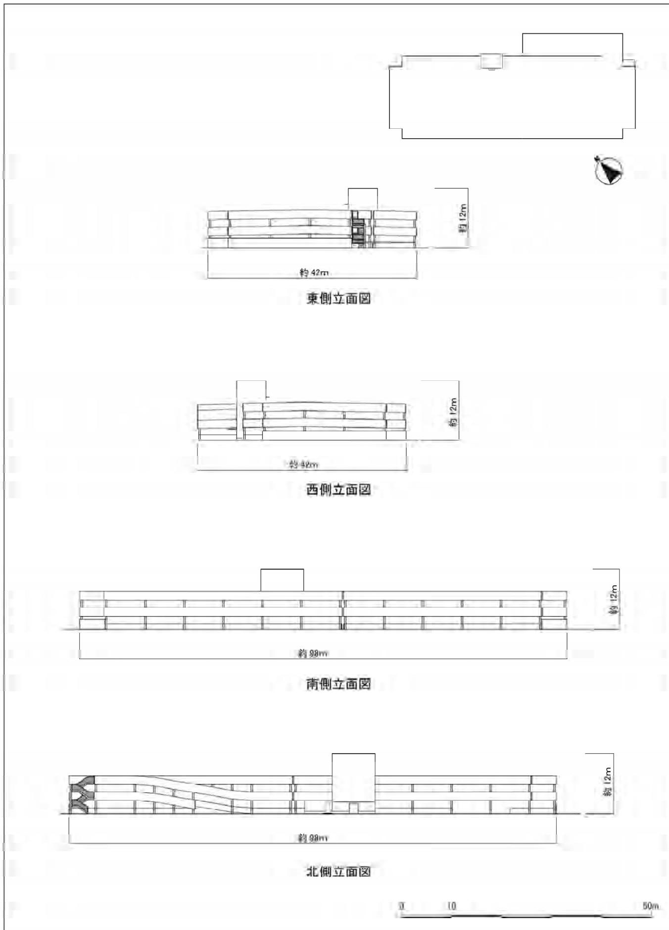
图 1-10(19) 西側立体駐車場 立面图
