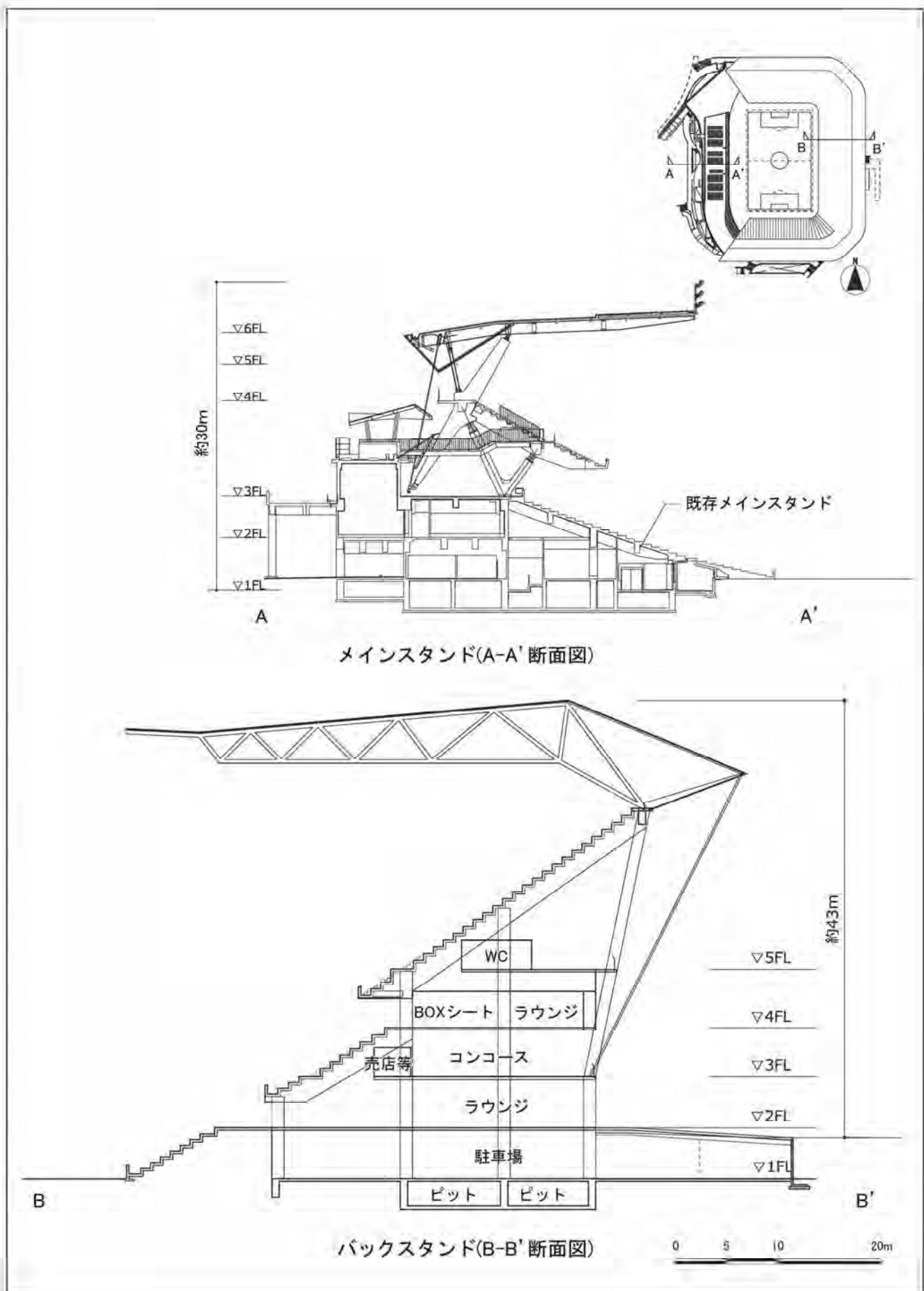
図 1-10(5) 球技専用スタジアム断面図
