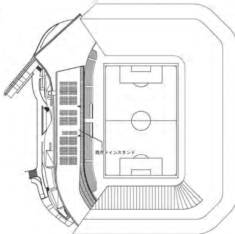
屋根伏図
