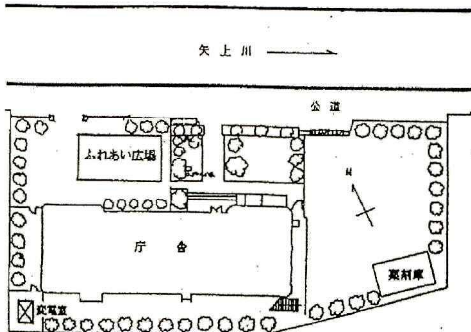
建物平面図
