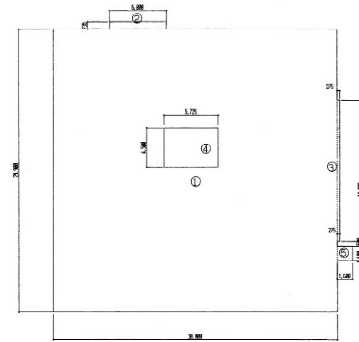
3階床面図 S=1/200
