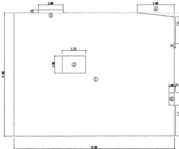
2階床面図 S=1/200
