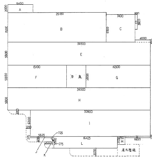
1階床面積求積図
