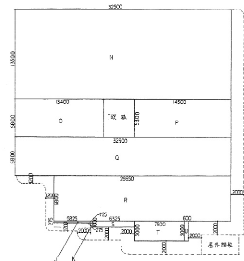
3階床面積求積図
