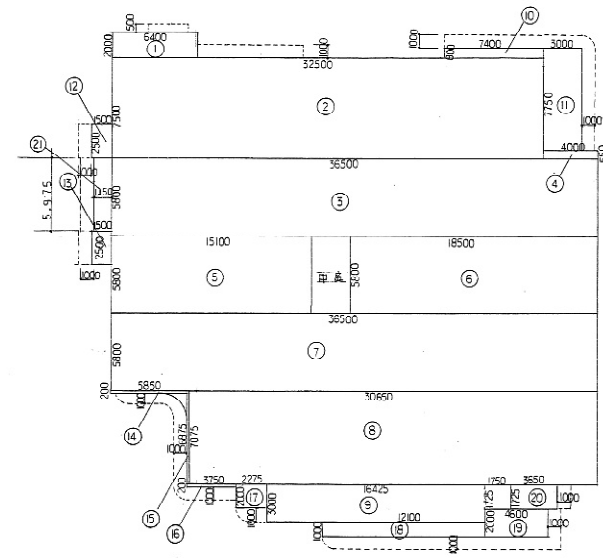
4階床面積求積図
