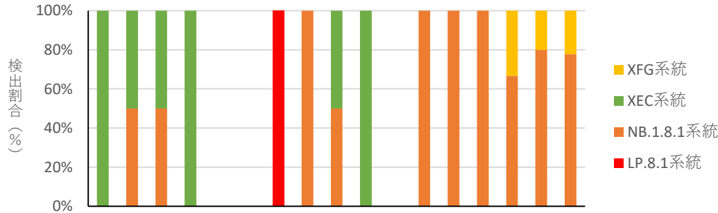
SARS-CoV-2各変異株の検出割合
