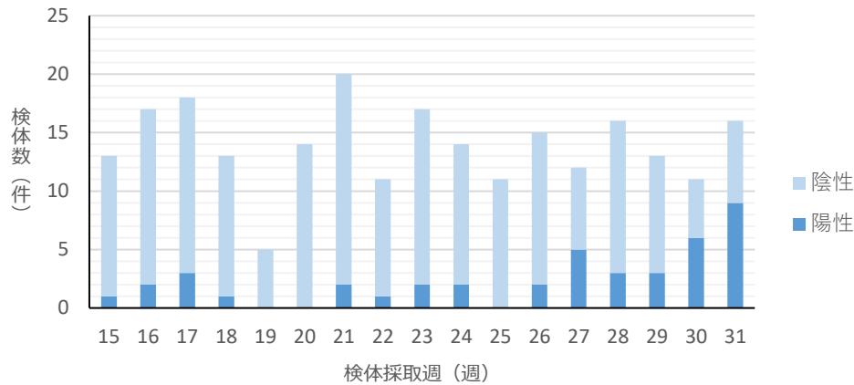
SARS-CoV-2変異株検出状況
