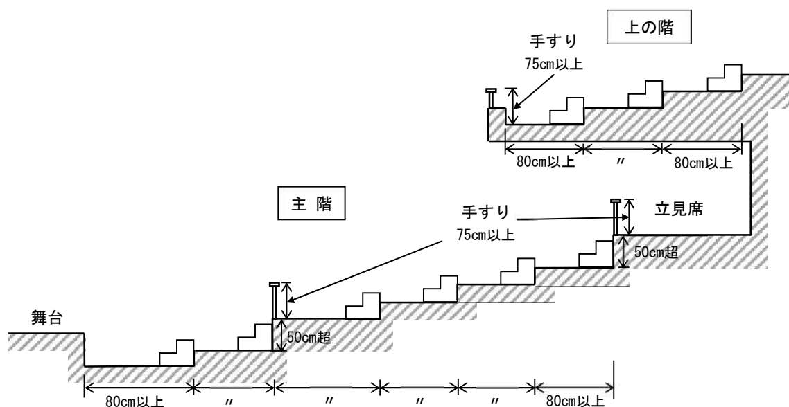
図1 客席の構造
