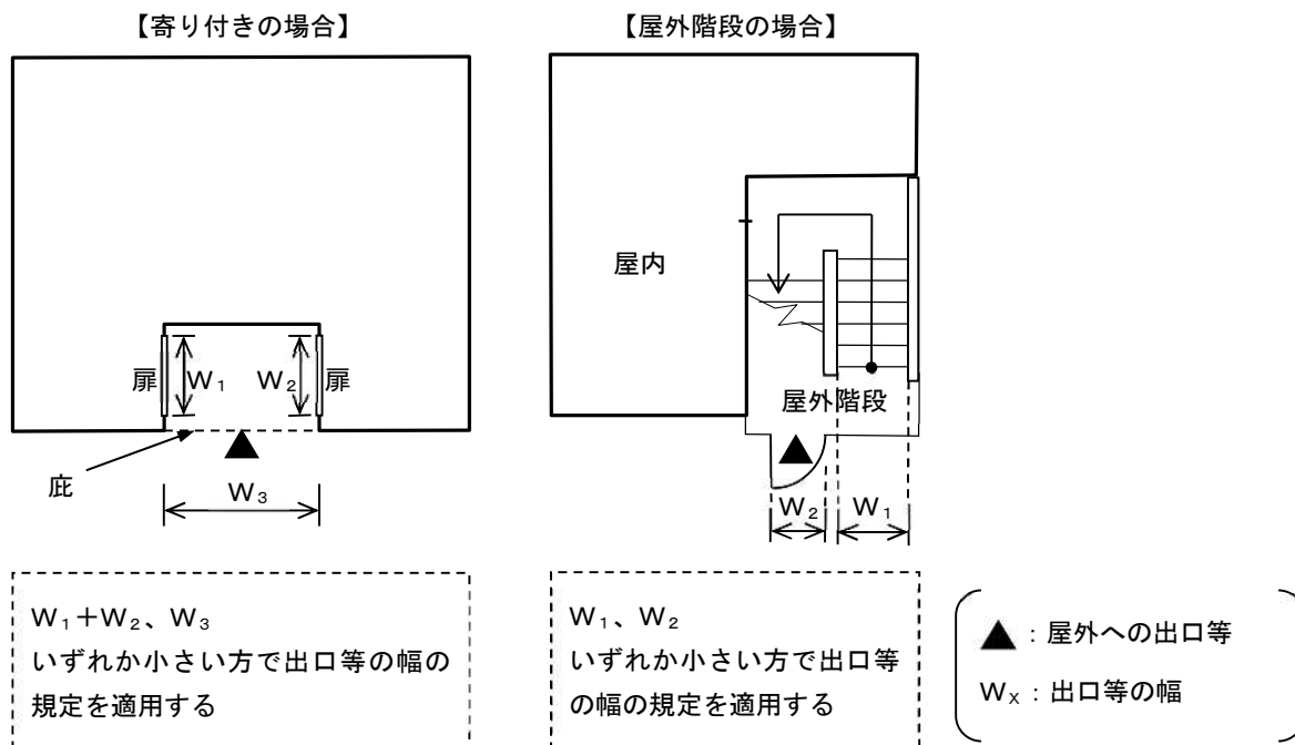
図3 出口等の例
