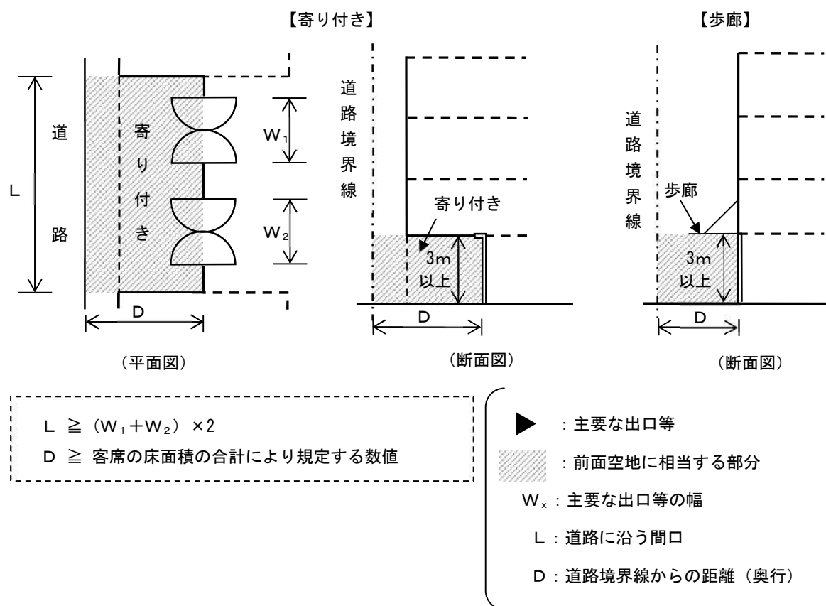
図2 歩廊又は寄り付きの構造
