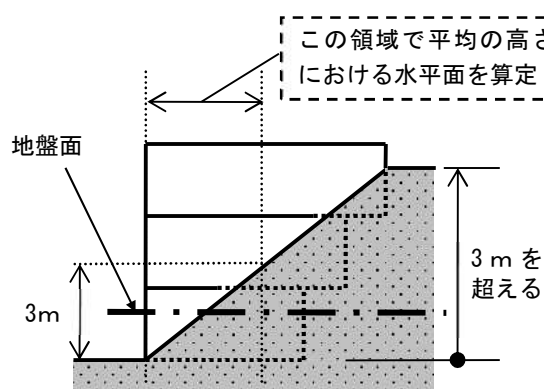
図2 建築物が周囲の地面と接する位置の 高低差が3mを超える場合
