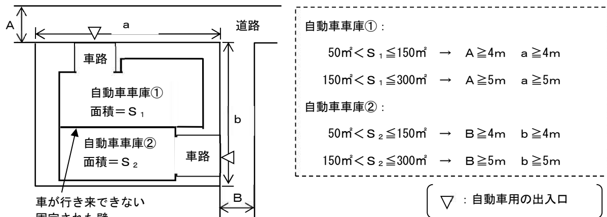
図4 出入口が2以上の道路に接する場合
