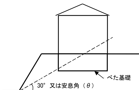
図7 ベた基礎の場合
