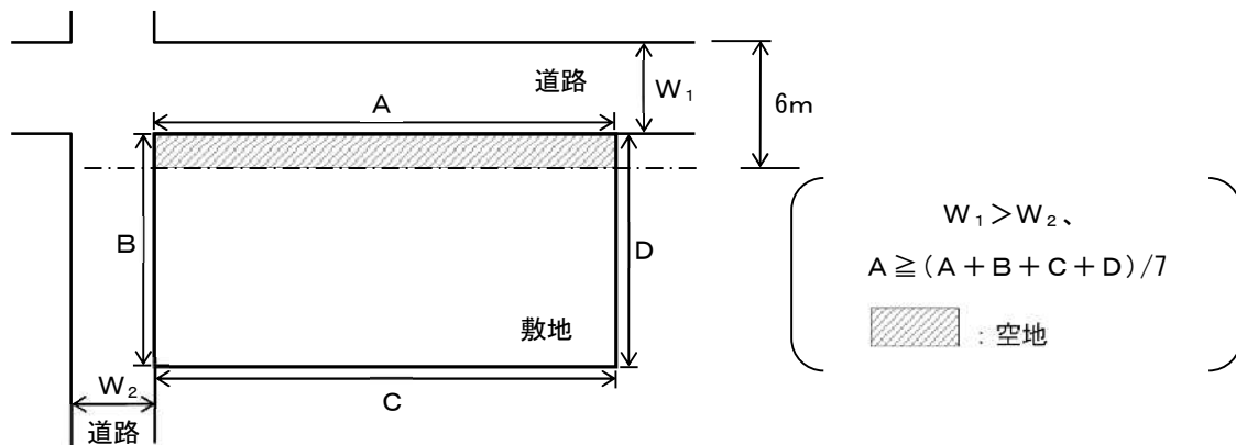
図5 2以上の道路に接する場合の例②
