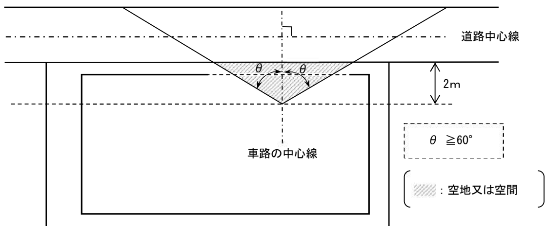
図2 道路の見通しができる空地又は空間を有するものの例
