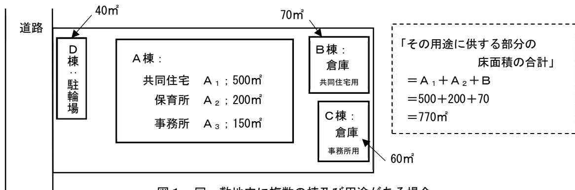
図1 同一敷地内に複数の棟及び用途がある場合
