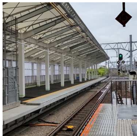
JR 横須賀線下りホーム新設工事の現状（令和 4 年 5 月）
