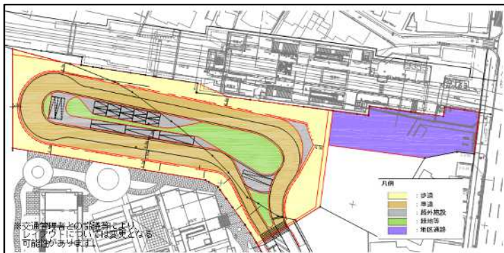
駅前交通広場イメージ図
