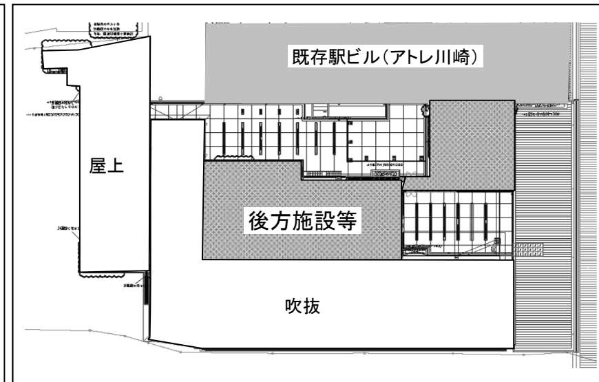
5階平面図
