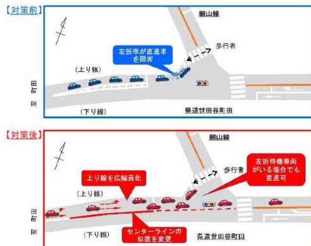
渋滞対策の効果の例（高石歩道橋下交差点） （川崎市報道発表資料より）
