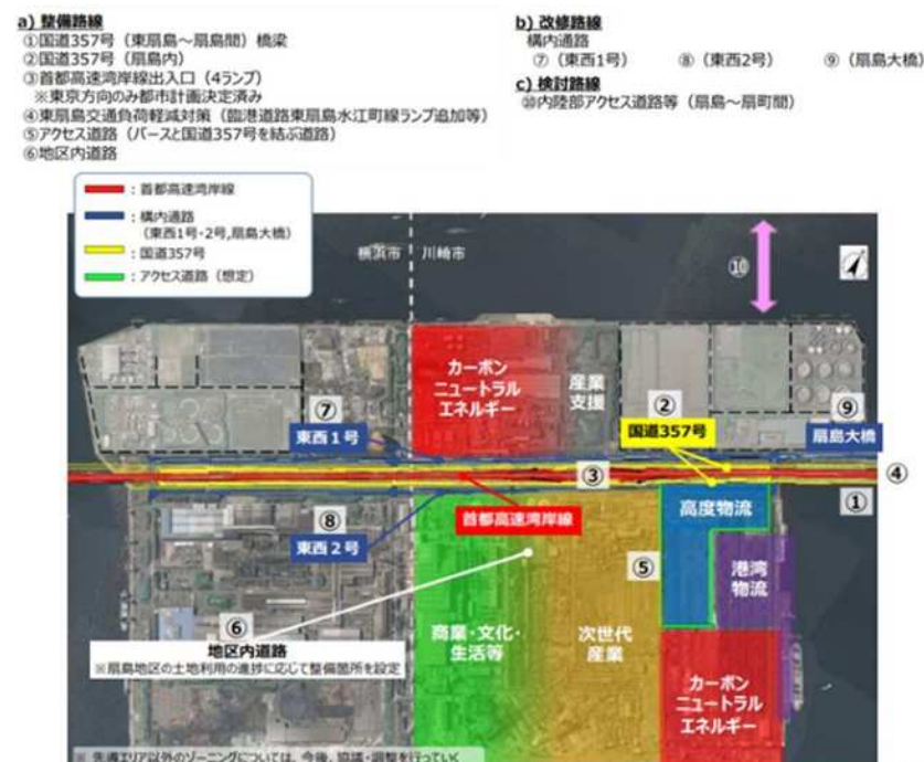
図 扇島地区において必要と想定する主な道路・交通アクセス路線と整備箇所 (出典)JFEスチール株式会社東日本製鉄所京浜地区の高炉等休止に伴う土地利用方針(令和5(2023)年8月)
