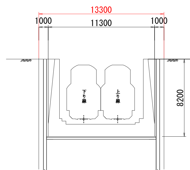
B-B断面
