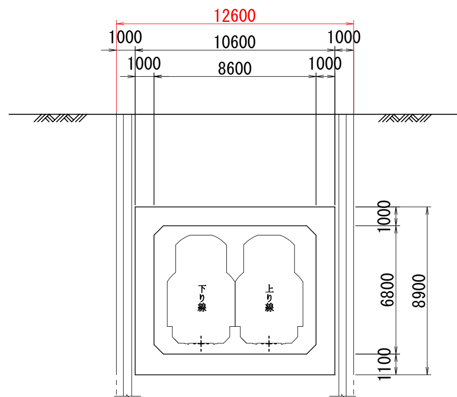
A-A断面
