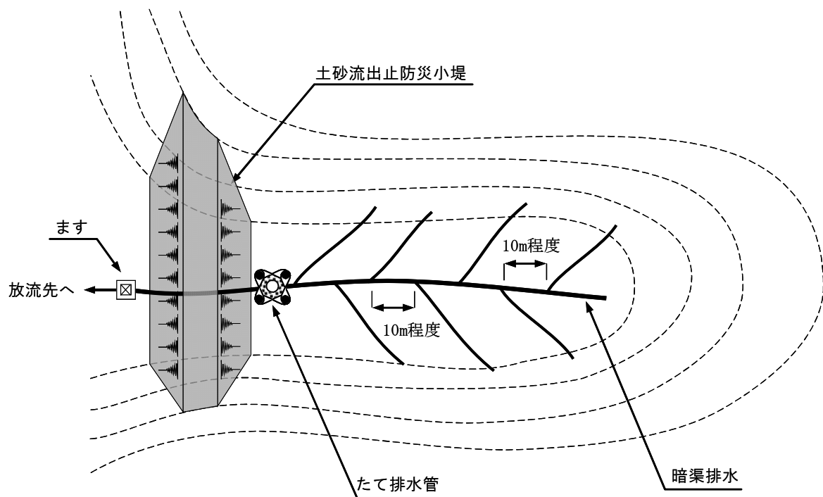
図 9-1 土砂流出止・仮排水のイメージ
