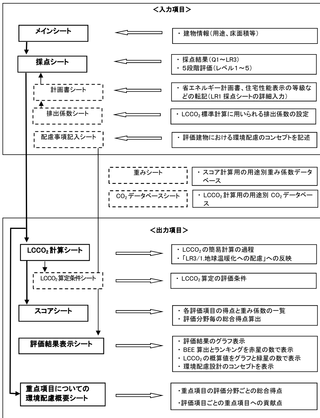
図6 評価シートの全体構成
