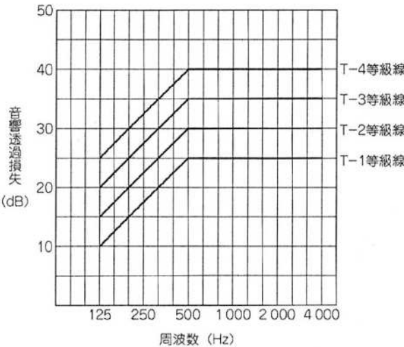
■参考) サッシ等の遮音等級曲線 (JIS A 4706)
