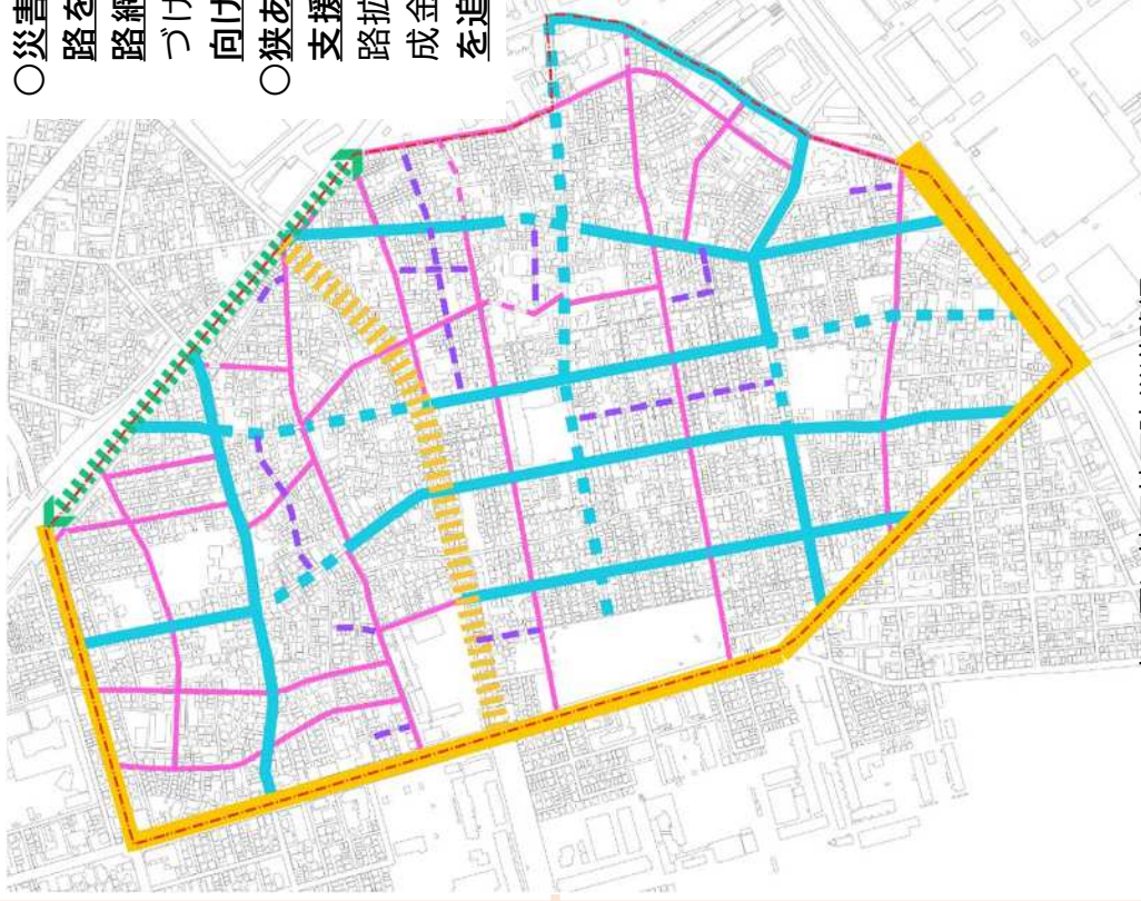
<小田周辺地区地区防災道路網>
