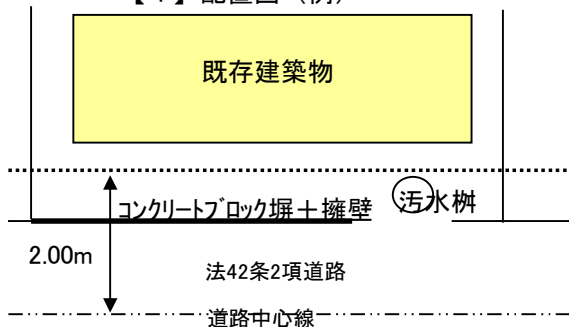
【1】配置図（例）
