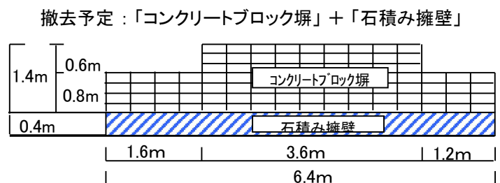
【2】展開図（例）
