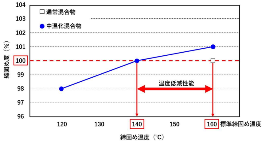
図3-2-6 温度-締固め度のグラフの作成例
