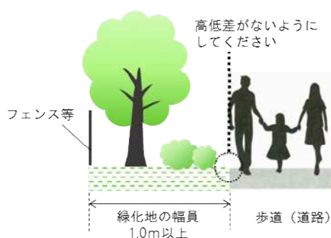
断面図
