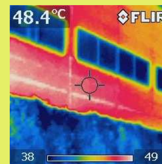
同一箇所でのサーモグラフィー測定結果
