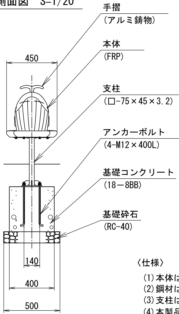
側面図 S=1/20
