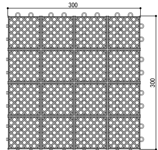
ジョイント式特殊樹脂マット (300×300×15(厚み)) S=1/5
