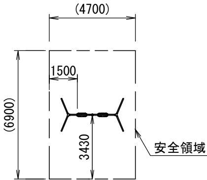
安全領域 S=1/200
