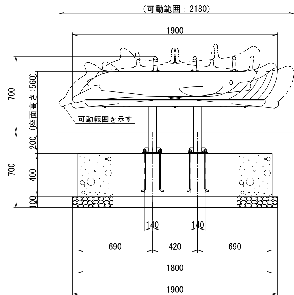
立面図 S=1/20
