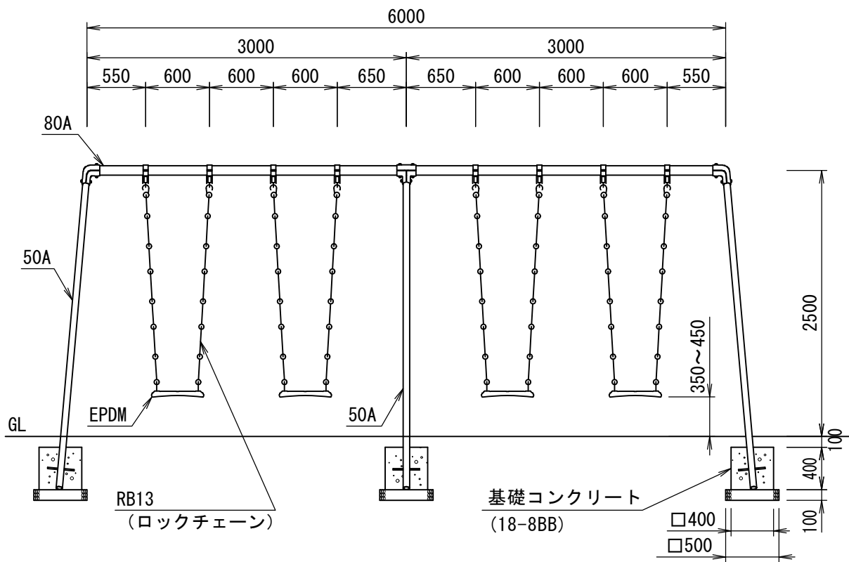
立面図 S=1/50
