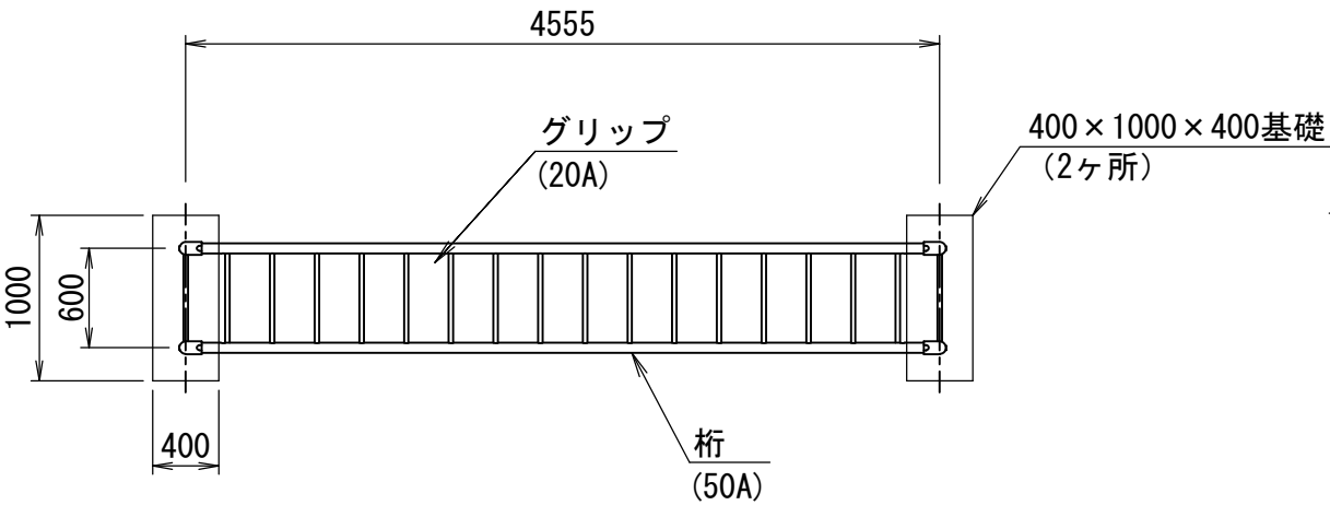
平面図 S=1/50
