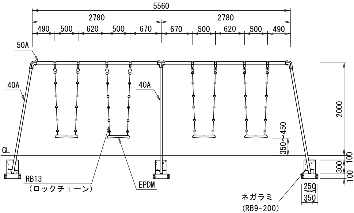
立面図 S=1/50
