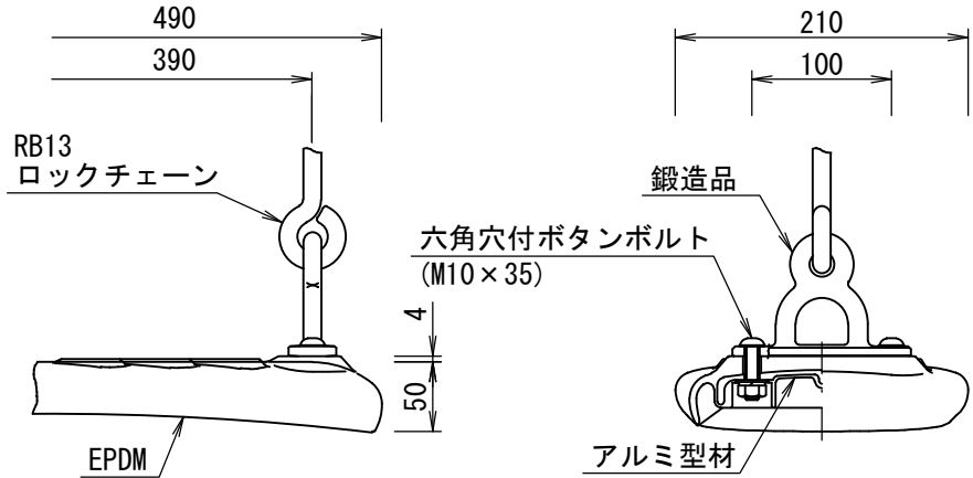
吊席詳細図 S=1/6
