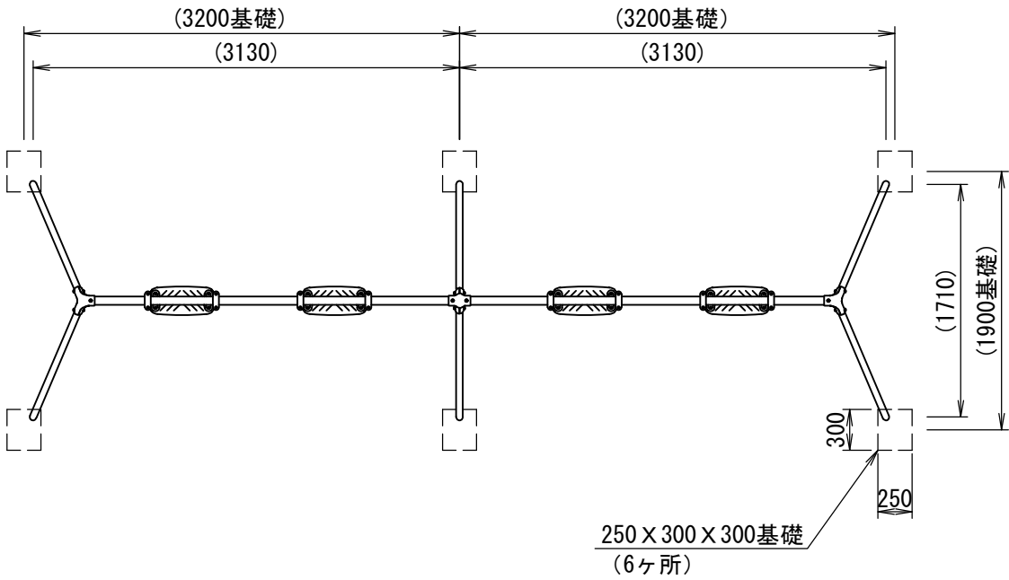
平面図 S=1/50
