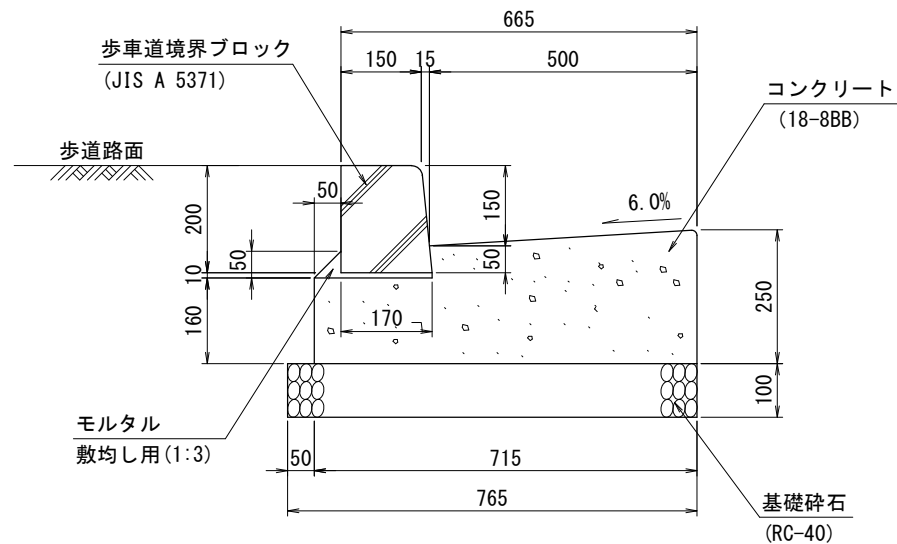
横断歩道部
