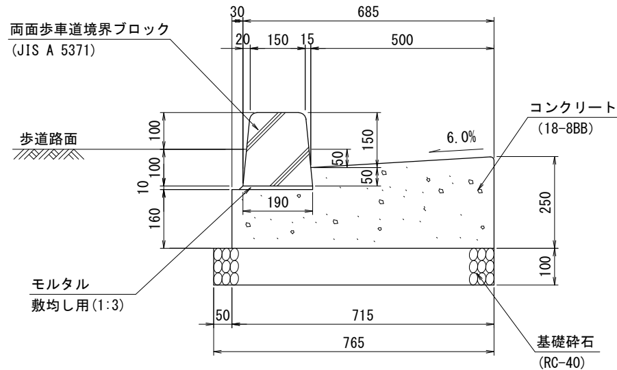
一般部
