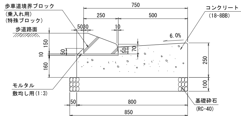
歩車道境界A種斜ブロック
