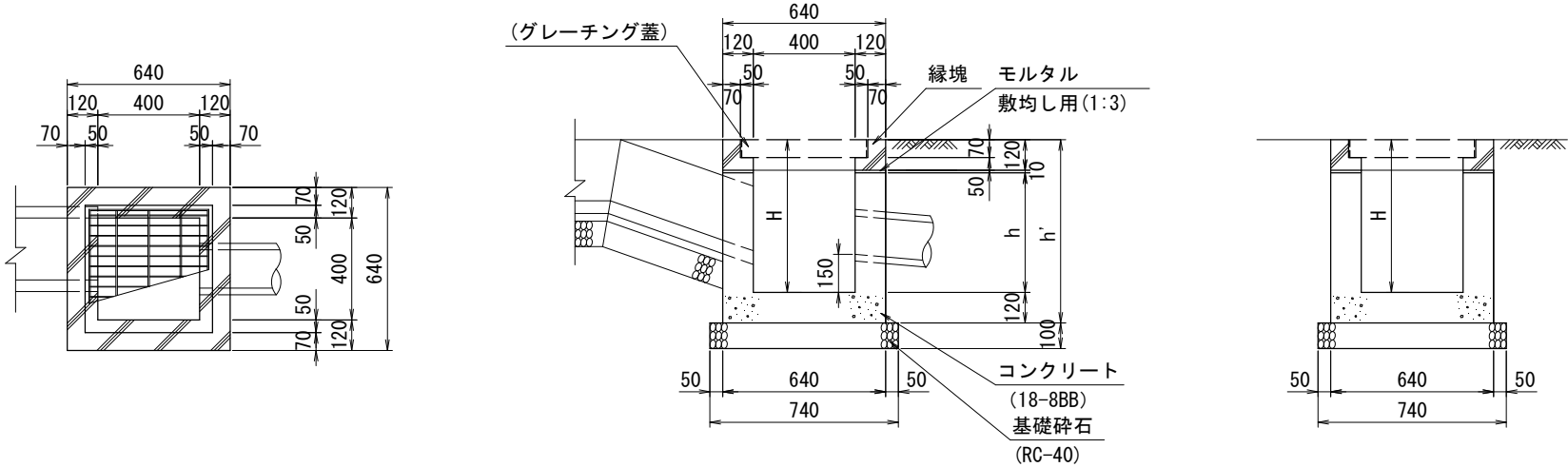
寸法表
