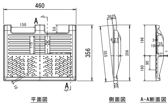
平面図
