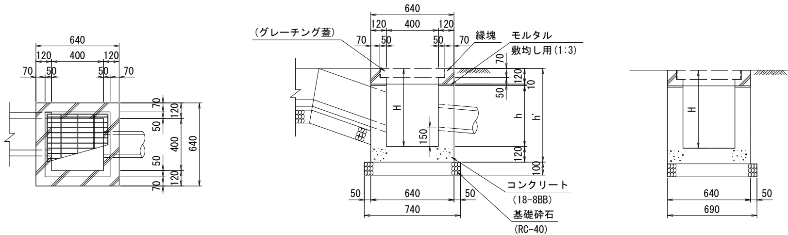
寸法表
