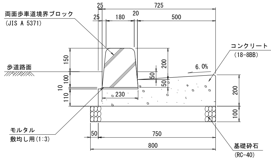
横断歩道部
