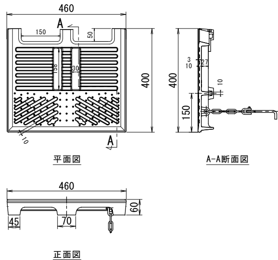
鑄鉄蓋（落葉対応型）
