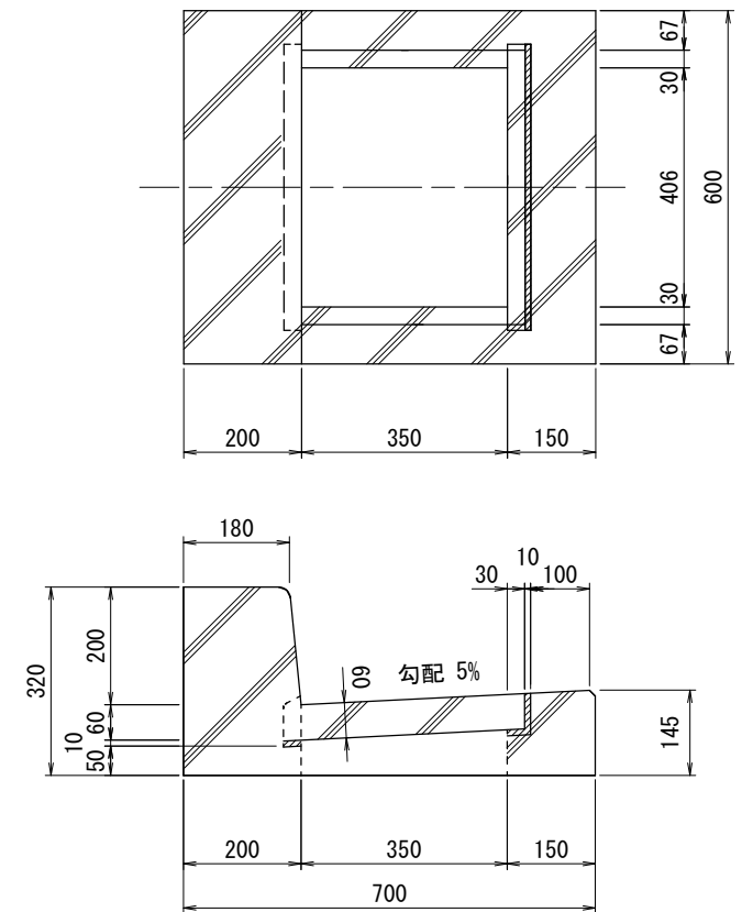
縁塊（205A用）
