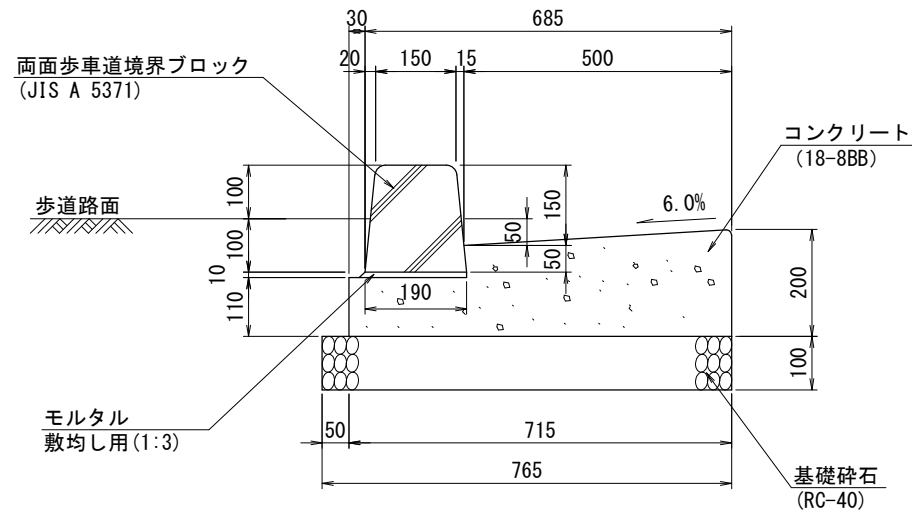
横断歩道部
