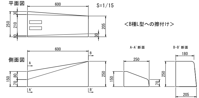
歩車道境界B種斜ブロック
