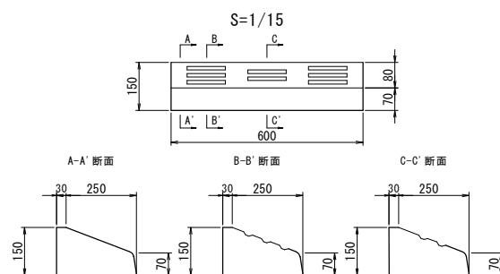
歩車道境界平ブロック（A、B共通）
