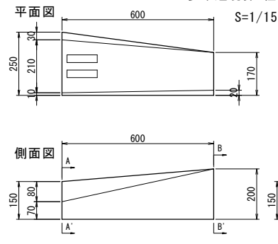
歩車道境界A種斜ブロック
