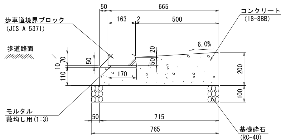
横断歩道部
