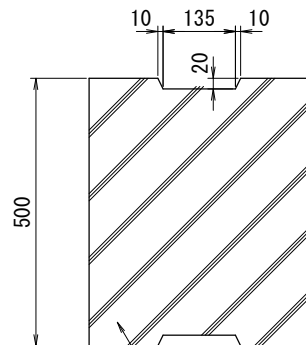
U型側溝ふた（落ちふた式）－（1種） (JIS A 5372)
