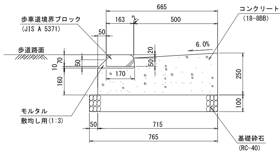
横断歩道部
