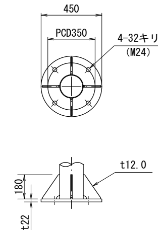
ベースプレート詳細図 S=1/20
