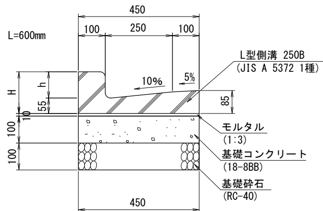
寸法表
