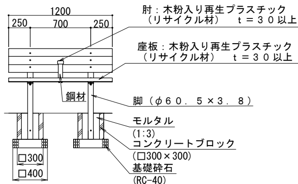
立面図
