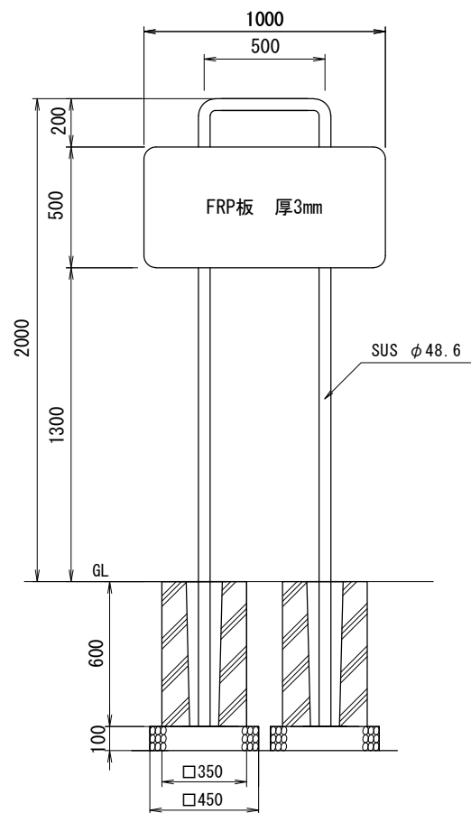
正面図 S=1/20
