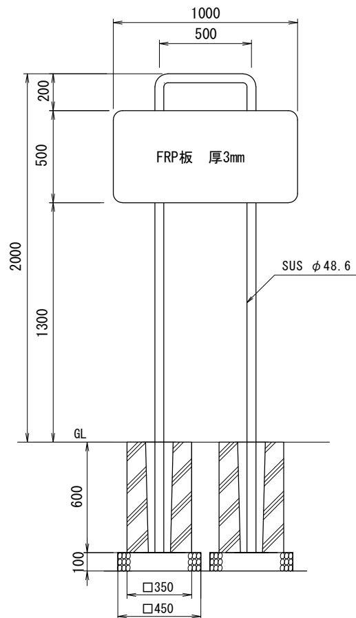
正面図 S=1/20
