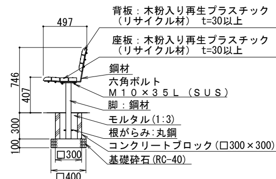
側面図
