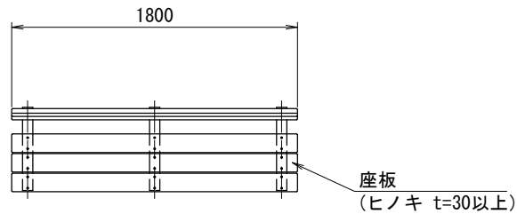
立面図
