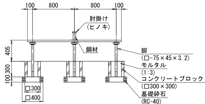
立面図
