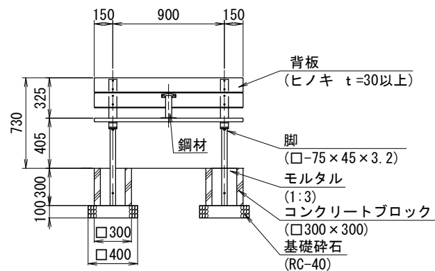
立面図
