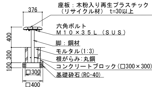
側面図
