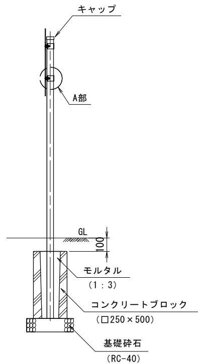
側面図 S=1/20
