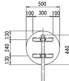
裏面図 S=1/20
