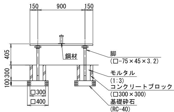
立面図
