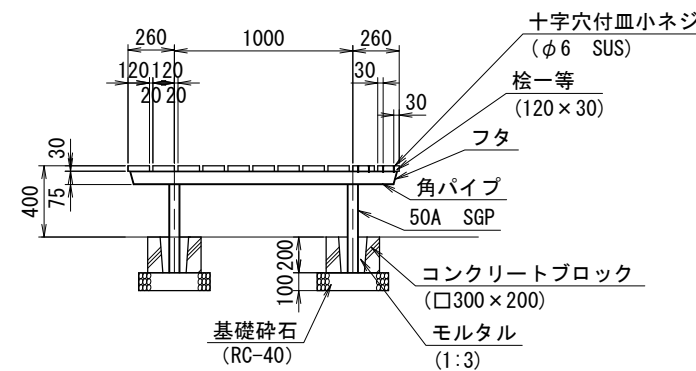
側面図
