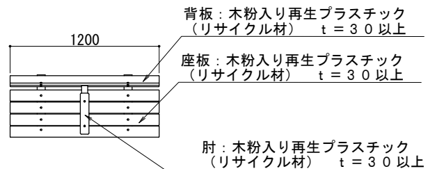
立面図
