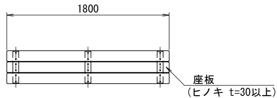
立面図
