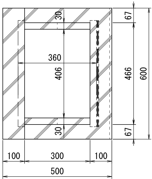
縁塊（鋳鉄蓋用）
