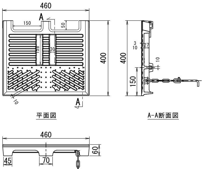
正面図
