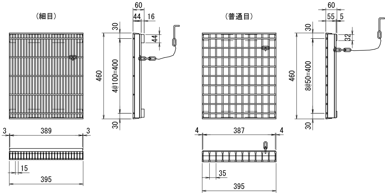
グレーチング蓋
