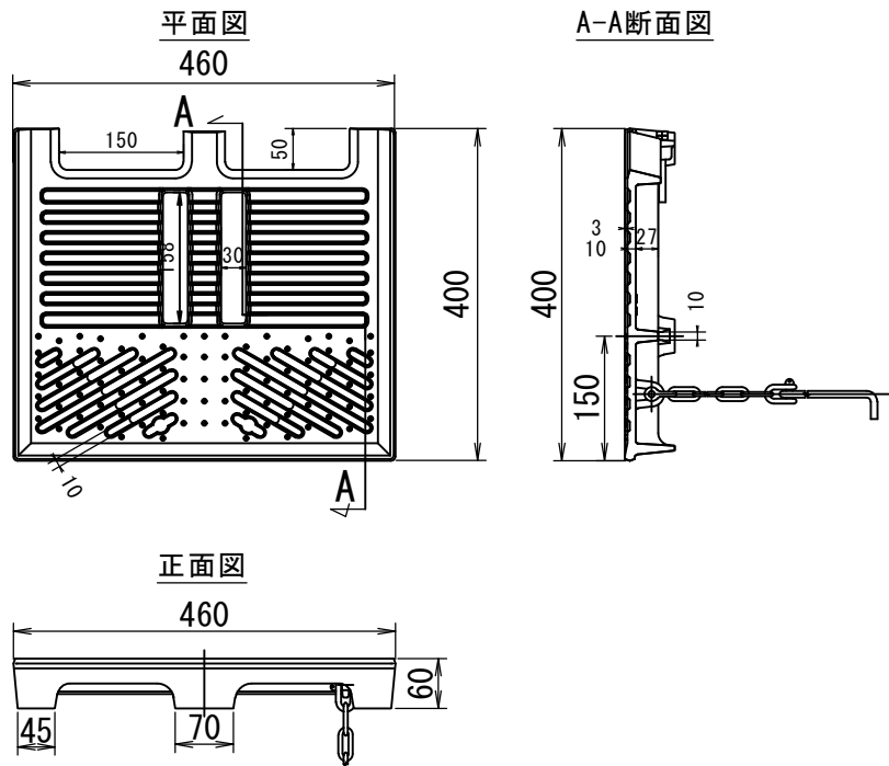
鋳鉄蓋（落葉対応型）
