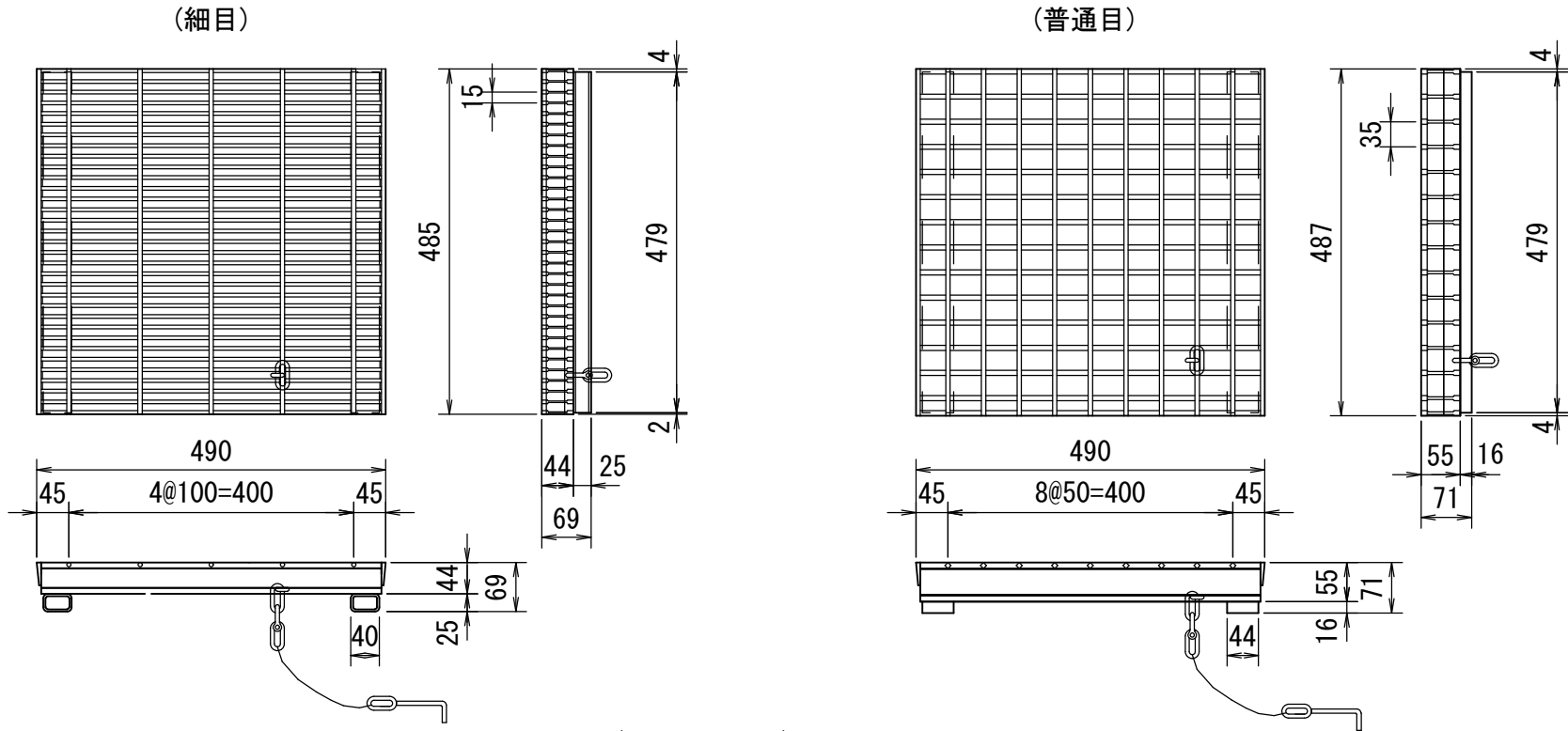
グレーチング蓋-500用
