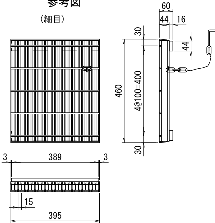
グレーチング蓋 参考図
