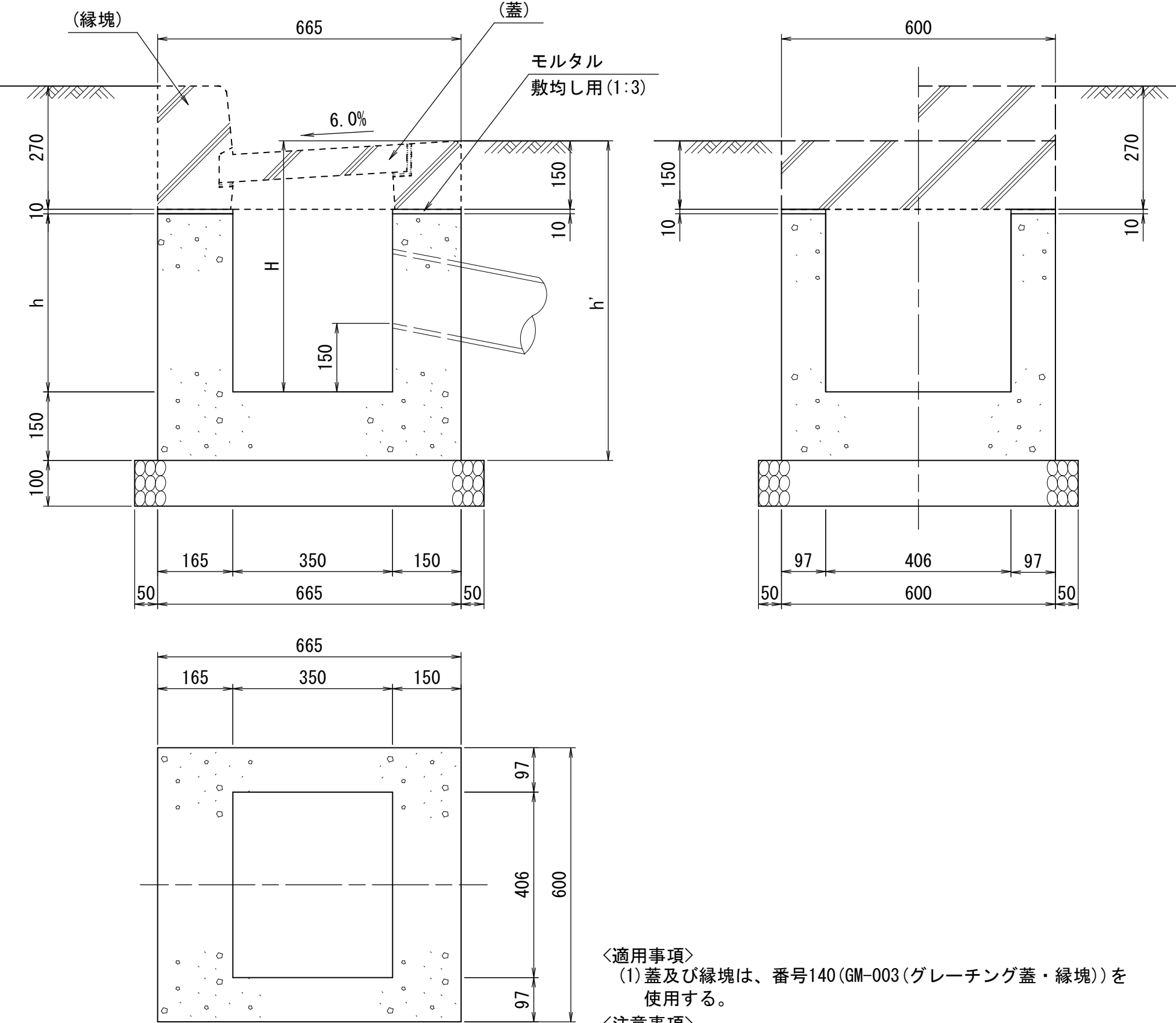
寸法表
