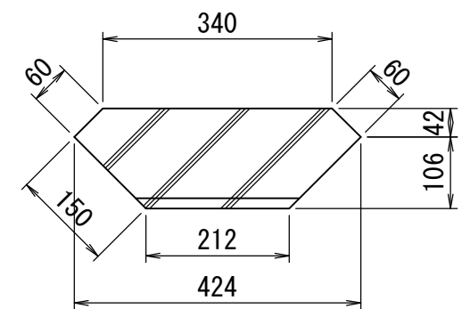
コーナーブロック S=1/10
