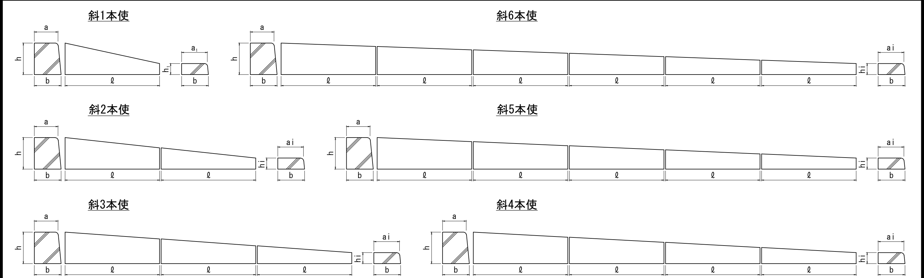
寸法表 (mm)
