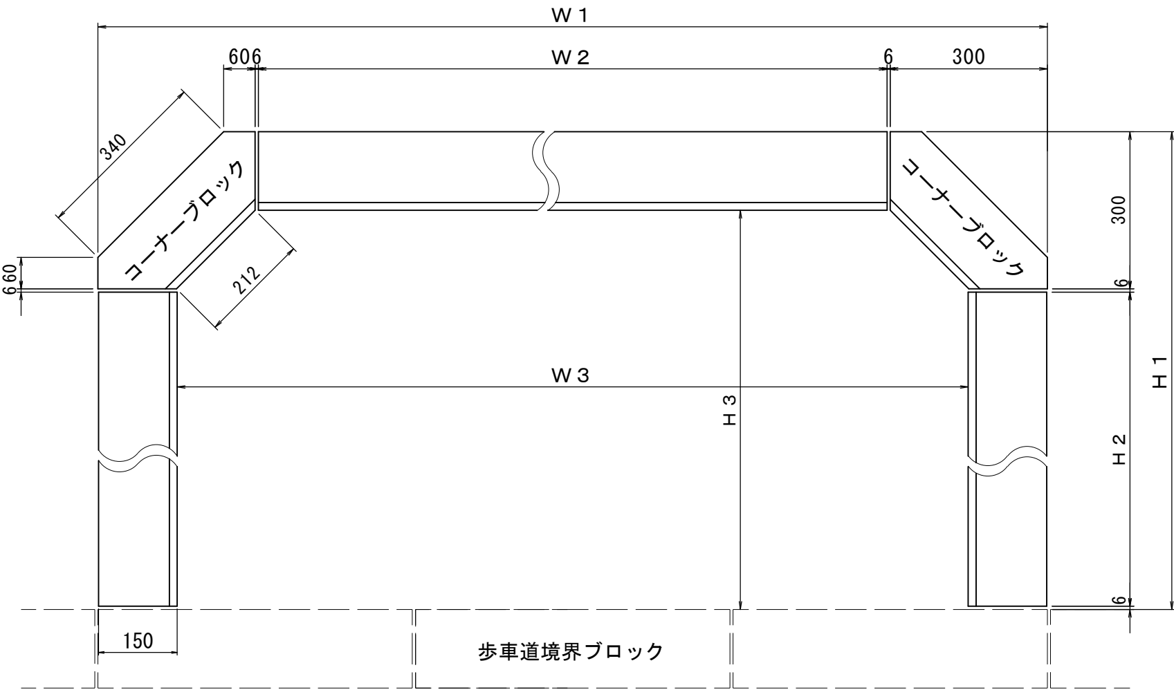
組合せ平面図
