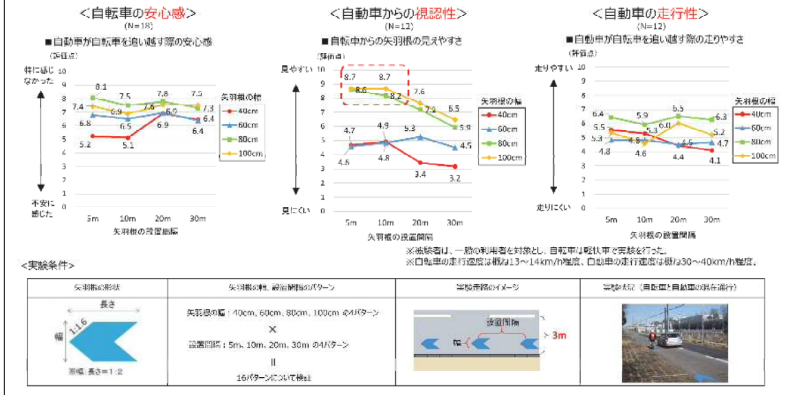
図 2-13 矢羽根型路面表示による効果の検証 (出典：国土技術政策総合研究所資料)
